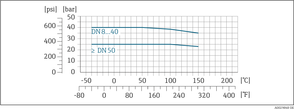
21 Mit Anschlusswerkstoff 1.4404 (316/316L)
