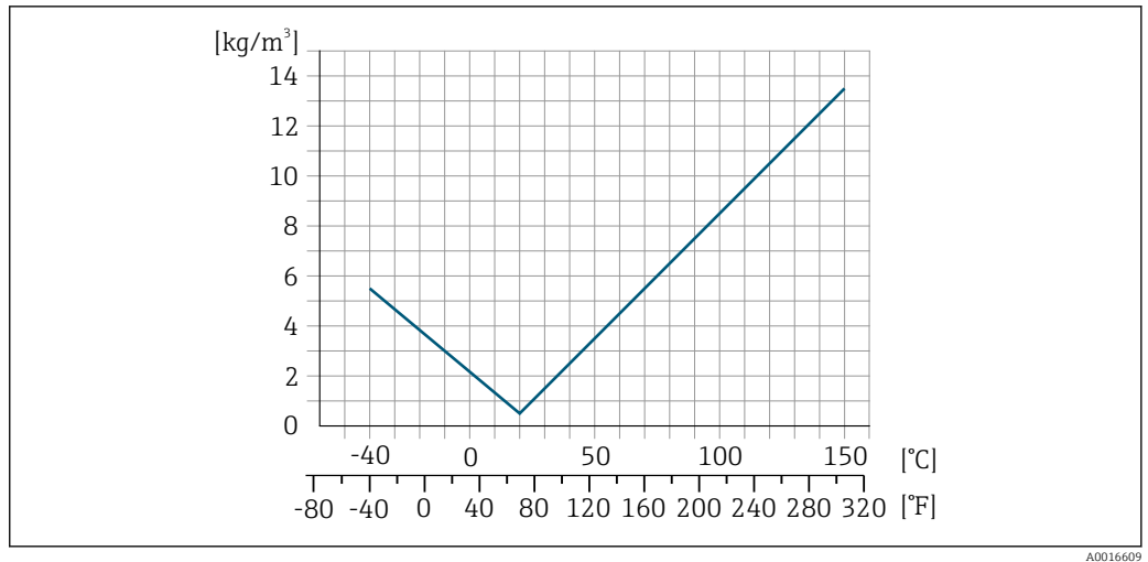
12 Felddichtejustierung, Beispiel bei +20 °C (+68 °F)
