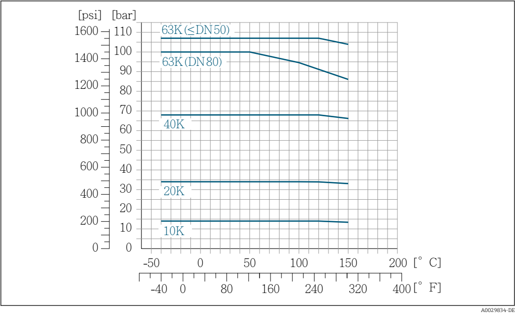
19 Mit Flanschwerkstoff 1.4404 (F316/F316L)
