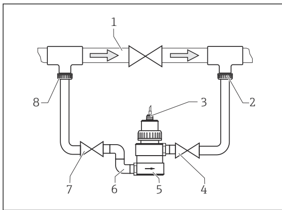
图 8 手动动作阀或电磁阀的旁路安装
