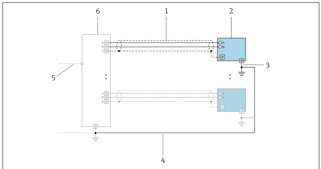
図 6 PROFINET over Ethernet-APL の接続例
