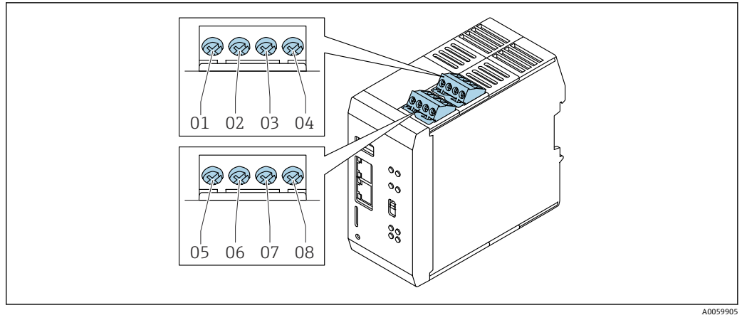
图 2 接线端子分配
