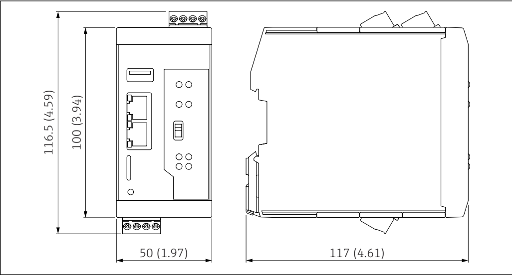
图 7 外形尺寸。测量单位 mm (in)
