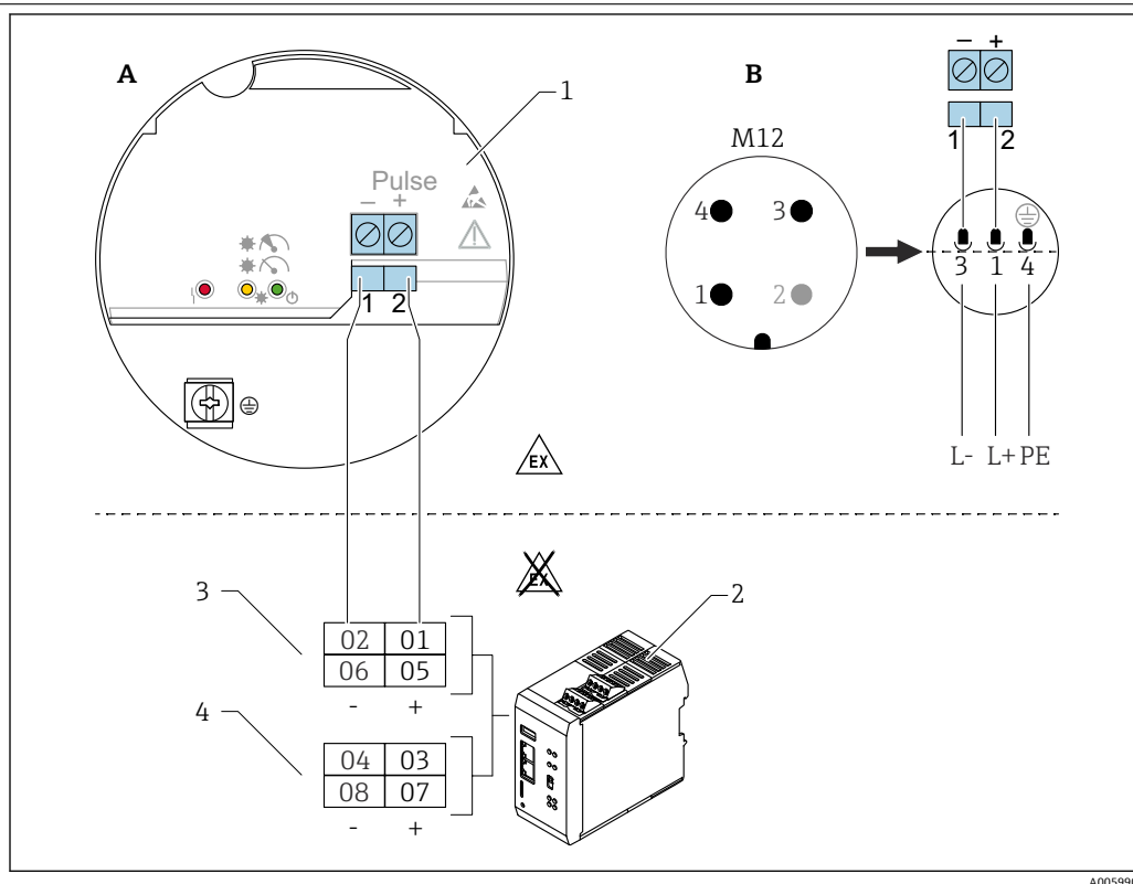
图 3 电子插件 FEL60D 和密度计算仪 QML51 的接线图
