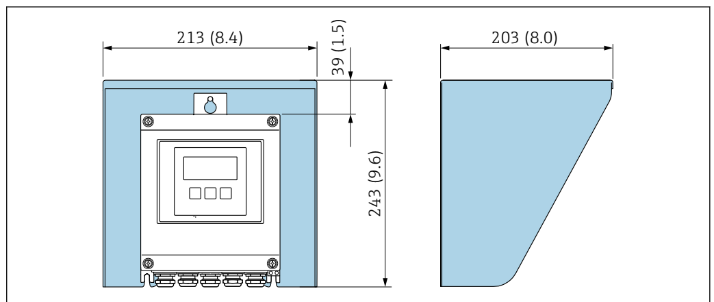
33 Tettuccio di protezione dalle intemperie per Proline 500 – digital; unità ingegneristica mm (in)
