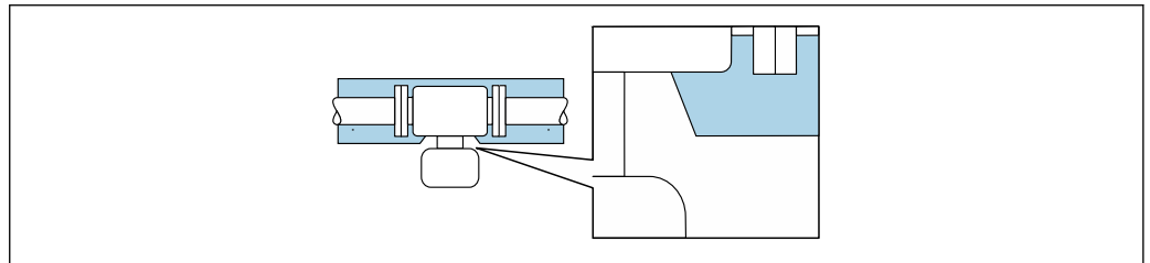
32 Coibentazione con collo esteso a vista
