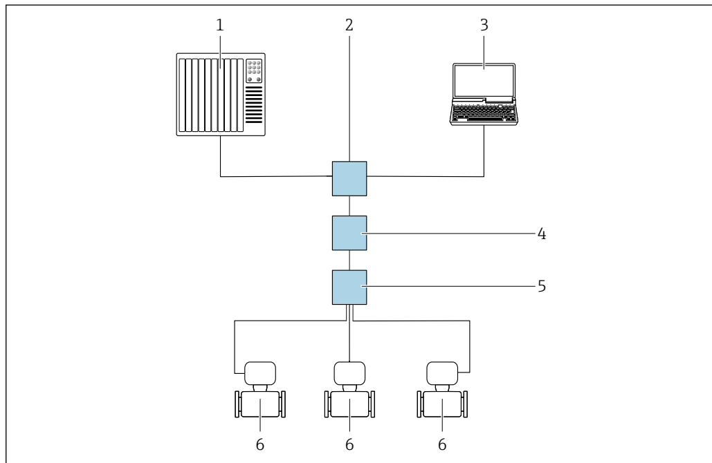
図 30 Modbus TCP over Ethernet-APL プロトコル経由のリモート操作オプション（アクティブ）
