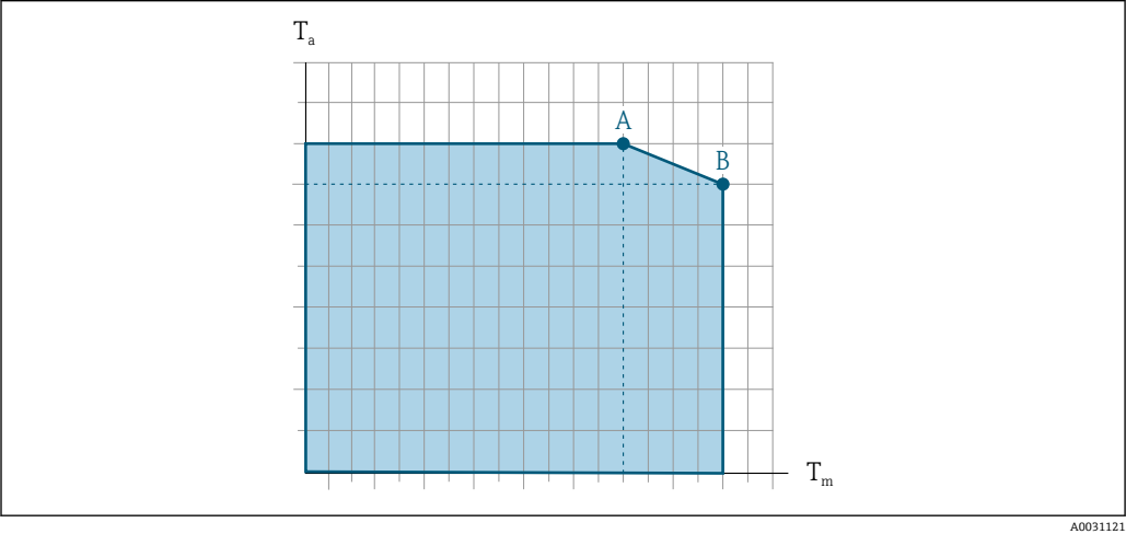
図 41 例示、値は下表を参照 Ta 周囲温度 Tm 測定物温度 A 許容最高測定物温度 Tm、Ta max = 60 °C (140 °F) 時；測定物温度 Tm が高い場合は、周囲温度 Ta を下げる必要があります。 B 規定されたセンサの最高測定物温度 Tm における許容最高周囲温度 Ta
