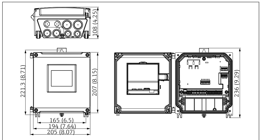
5 Abmessungen Feldgehäuse Polycarbonat. Maßeinheit mm (in)
