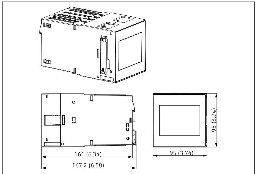
50 Hutschienengehäuse. Maßeinheit mm (in)
