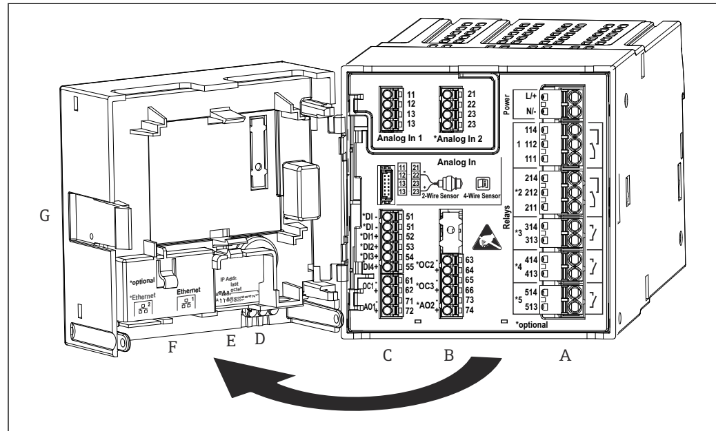
17 Anschlussklemmen Hutschienengerät; Klemmenausrüstung: steckbare Push-in-Klemmen
