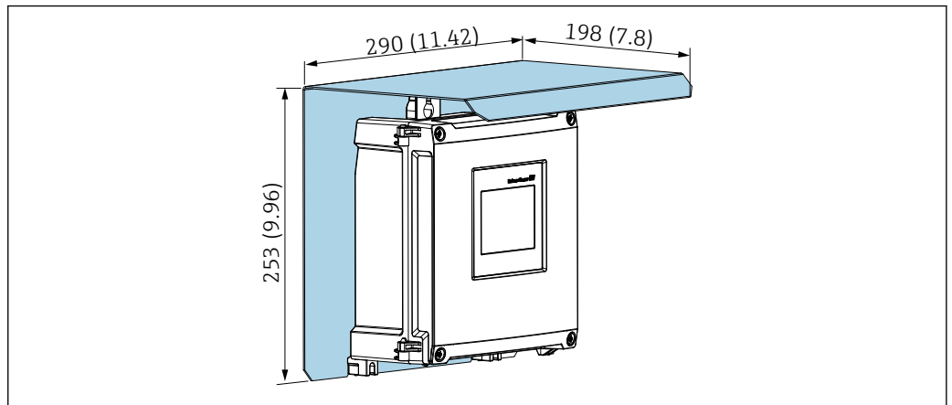
8 Wetterschutzhaube (Zubehör) zur direkten Wandmontage oder mittels Montageplatte (Zubehör) zur Rohrmontage. Maßeinheit mm (in)
