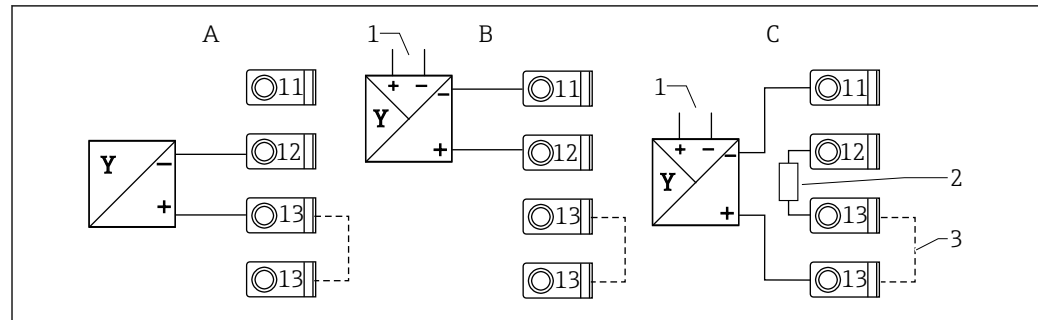
23 Anschlussbeispiele 2-Leiter- und 4-Leiter Sensor am 4 ... 20 mA Stromeingang bzw. HART
