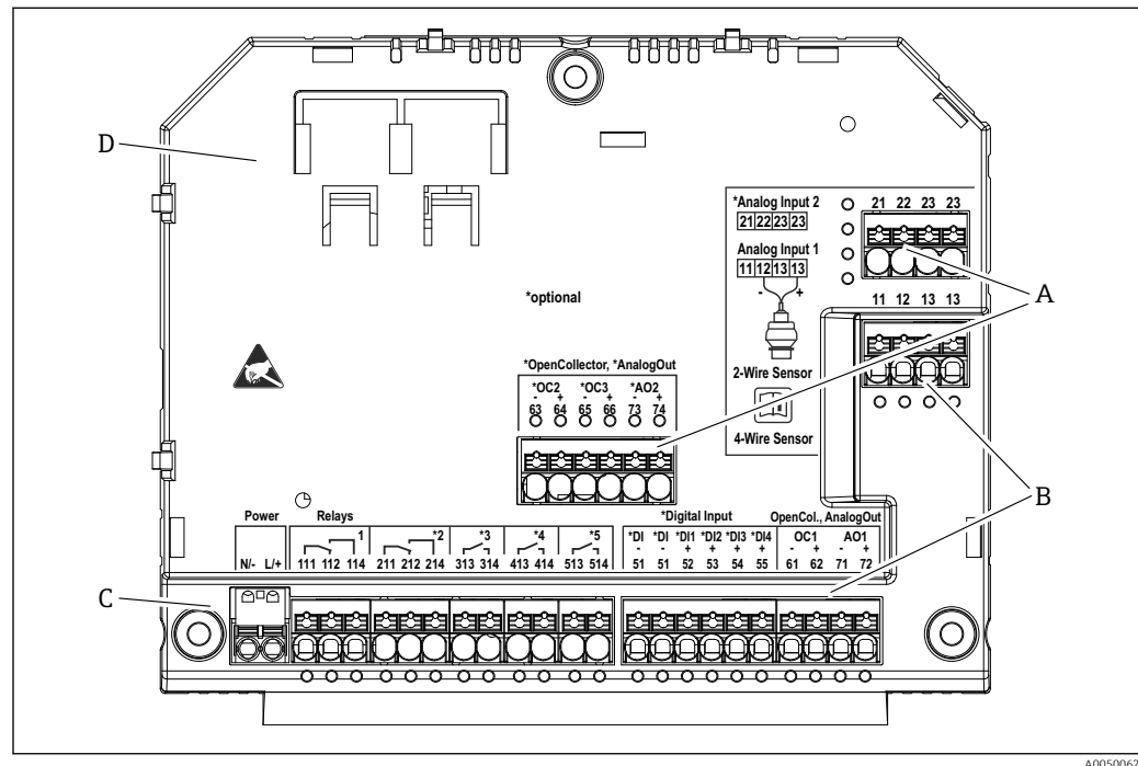
45 Anschlussklemmen im Klemmenraum Feldgehäuse Polycarbonat; Klemmenausführung: Push-in-Klemmen
