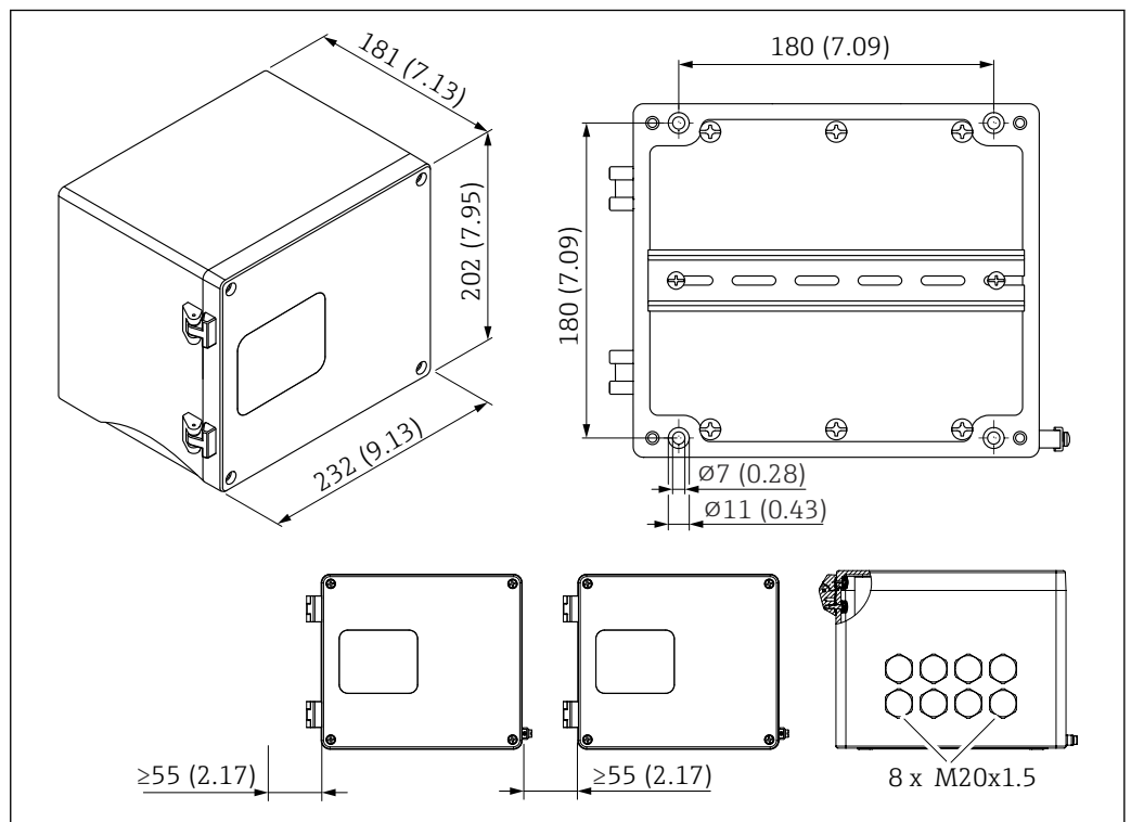
9 Abmessungen Feldgehäuse Aluminium. Maßeinheit mm (in)
