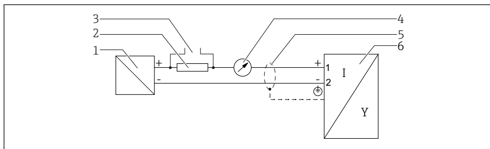
12 Diagrama de bloco, 2 fios: 4-20 mA HART
