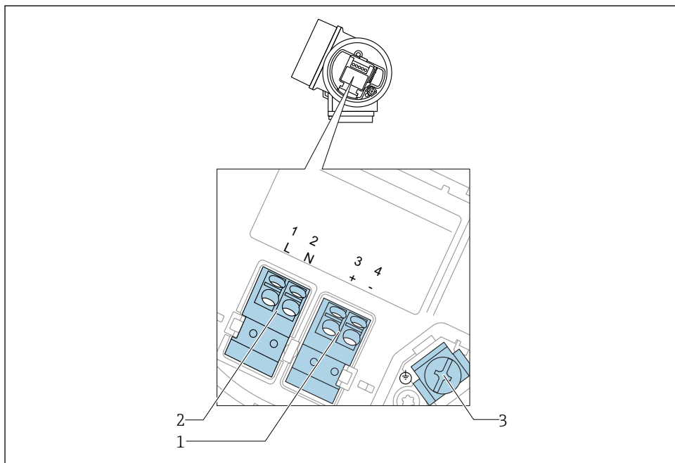
19 Esquema de ligação elétrica 4 fios: 4-20 mA HART (90 para 253 V AC )
