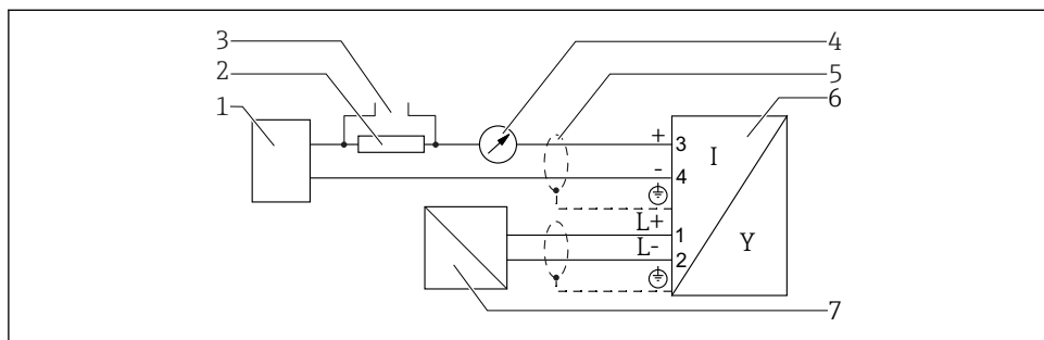
18 Diagrama de bloco, 4 fios: 4-20 mA HART (10.4 para 48 V DC )
