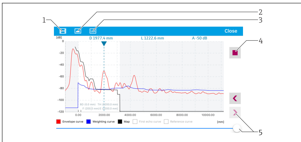
30 Display de curva envelope (exemplo) em SmartBlue; visualização iOS
