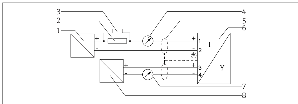
16 Diagrama de bloco, 2 fios: 4-20 mA HART, 4-20 mA
