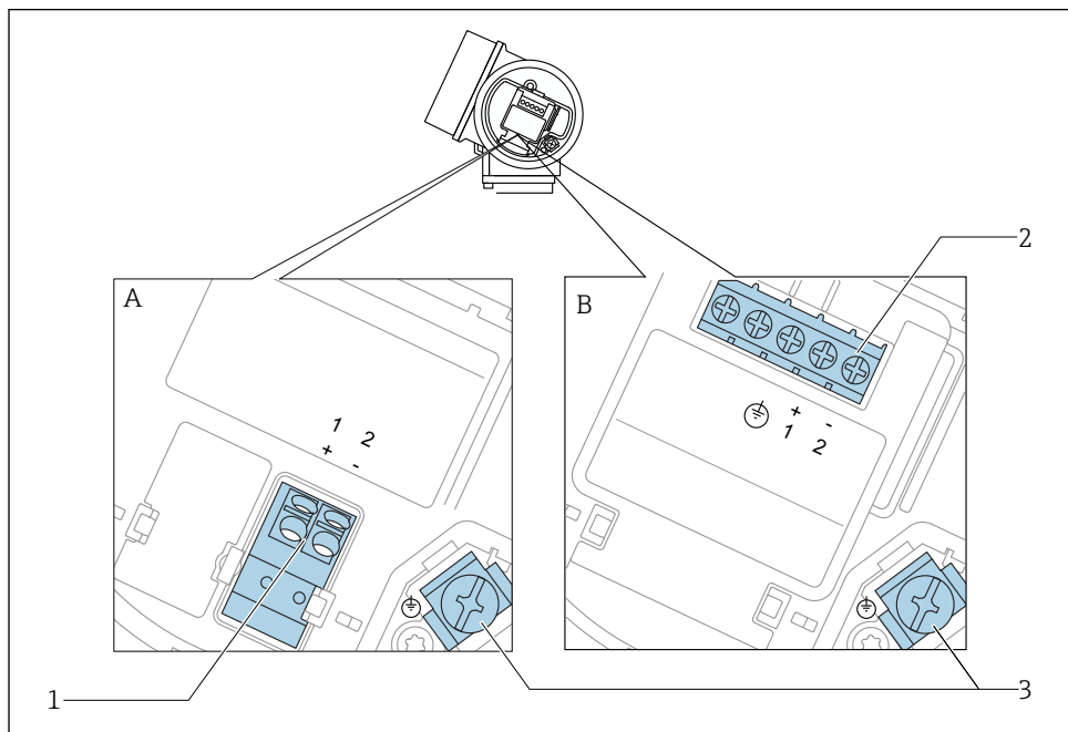
11 Esquema de ligação elétrica, 2 fios: 4-20 mA HART
