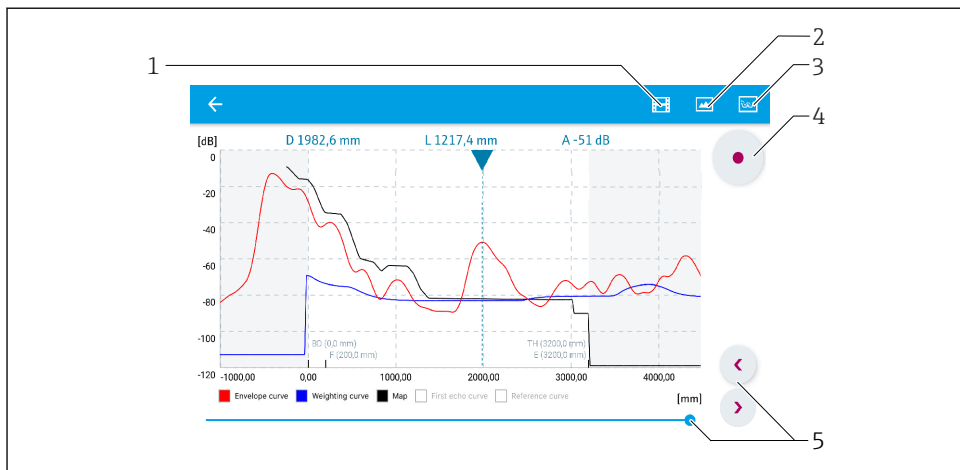
29 Display de curva envelope (exemplo) em SmartBlue; visualização Android
