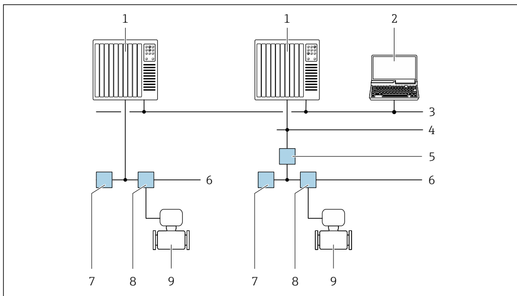
32 Варианты дистанционного управления по сети FOUNDATION Fieldbus
