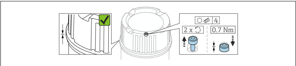
🖼 16 带锁定螺丝的外壳盖
