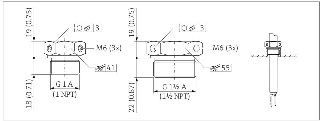
图 37 常压滑动套管 p_e = 0 \text{ bar} (0 psi)。测量单位 mm (in)
