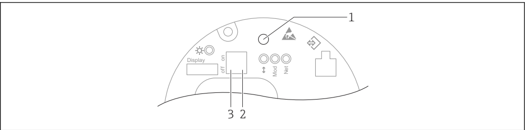
图 21 Ethernet-APL 通信型电子插件（FEL60P）上的操作按键和 DIP 开关
