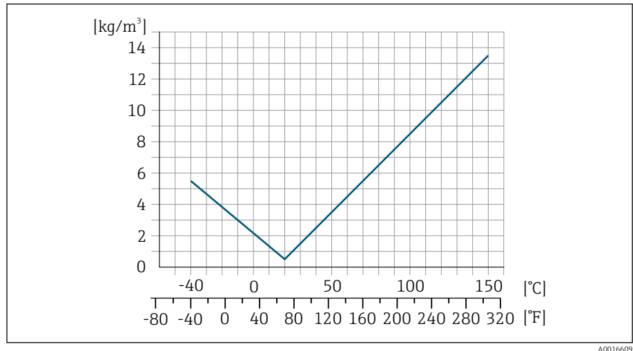
8 Étalonnage sur site de la masse volumique, exemple pour +20 °C (+68 °F)
