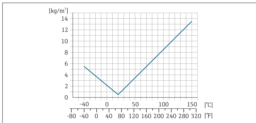
図 13 現場密度調整、例：+20 °C (+68 °F) 時
