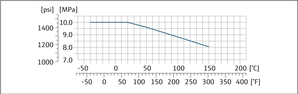
図 26 接続部の材質 1.4404 (SUS 316 相当または SUS 316L 相当)
