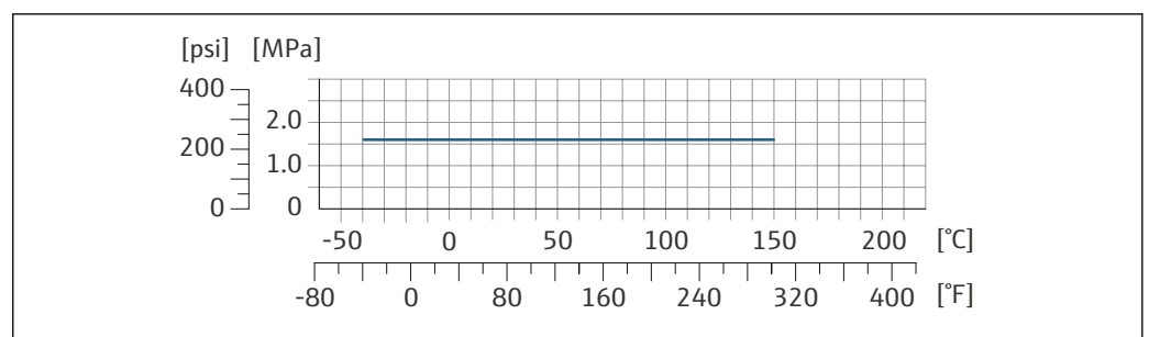
図 25 接続部の材質 1.4404 (SUS 316 相当または SUS 316L 相当)
