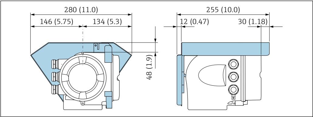
16 単位 mm (in)
