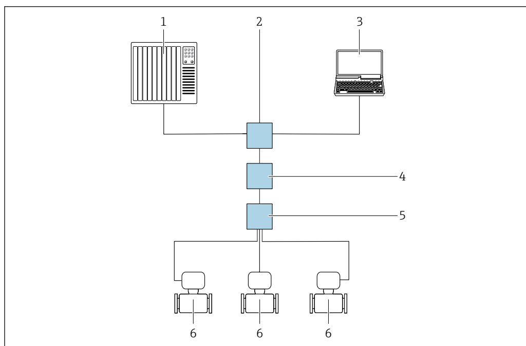
図 46 Modbus TCP over Ethernet-APL プロトコル経由のリモート操作用オプション（アクティブ）
