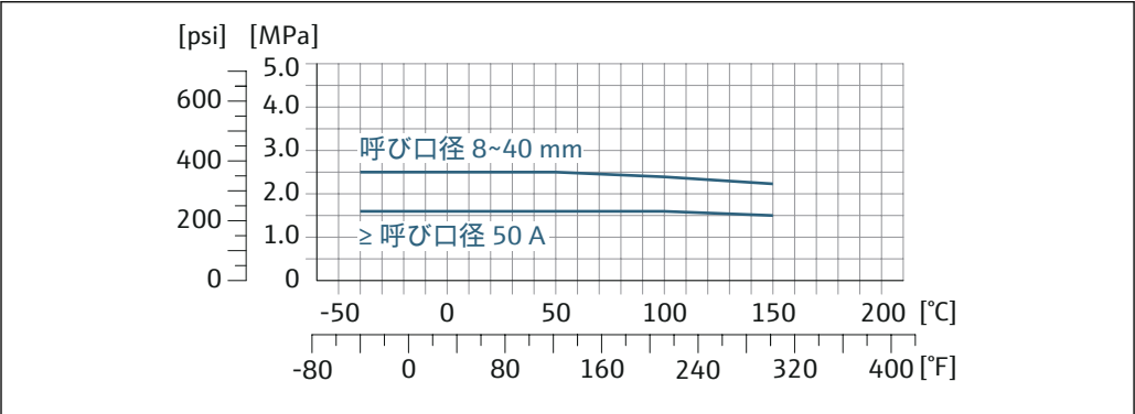
図 21 フランジ材質 1.4404 (SUS 316 相当または SUS 316L 相当)
