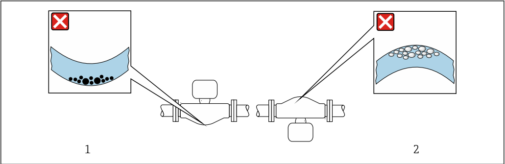
☒ 15 弓形計測チューブセンサの取付方向
