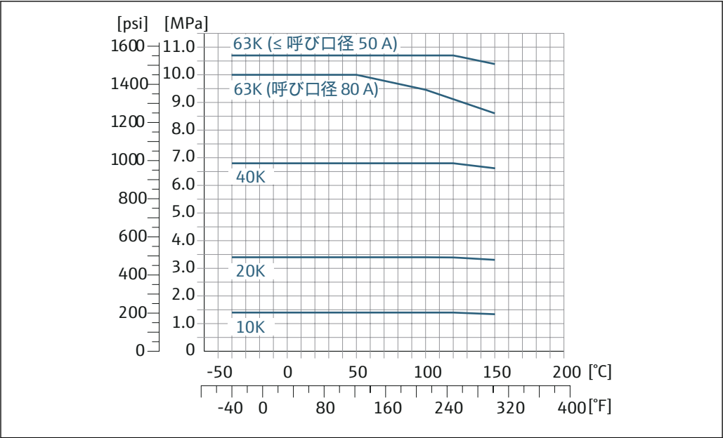
図 20 フランジ材質 1.4404 (SUS F316 相当または SUS F316L 相当)
