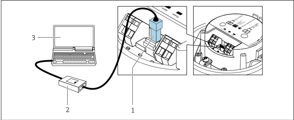
1 Interface service (CDI) de l'appareil de mesure 2 Commubox FXA291 3 Ordinateur avec outil de configuration FieldCare et DTM COM "CDI Communication FXA291"
