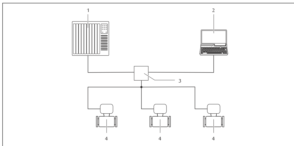
47 Options de configuration à distance via réseau PROFINET
