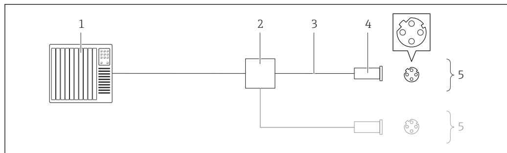
14 Exemple de raccordement pour EtherNet/IP
