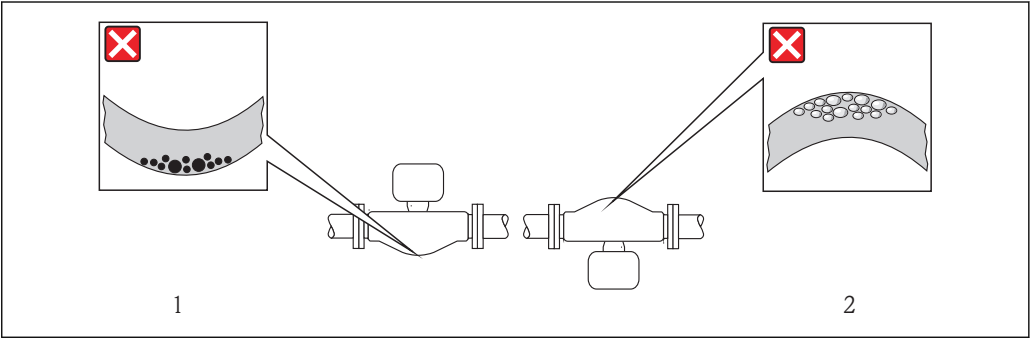
☒ 19 Orientation du capteur avec tube de mesure soudé
