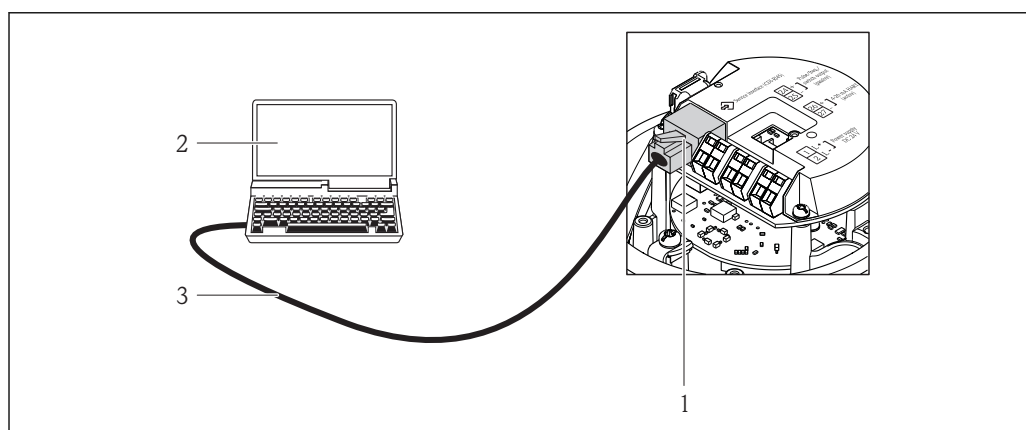
48 Raccordement pour variante de commande "Sortie", Option B : 4-20 mA HART, sortie impulsion/fréquence/tor
