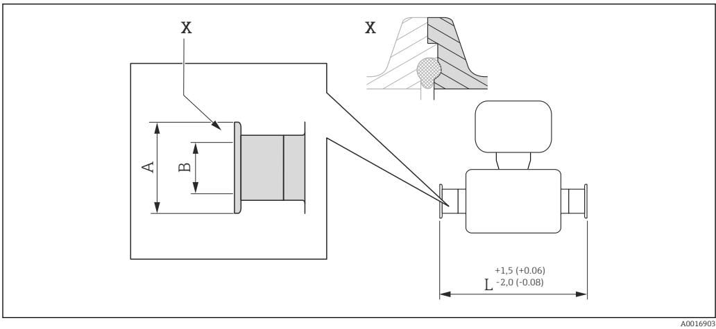
36 Détail X : raccord process asymétrique, la partie grisée fait partie de la livraison. Unité de mesure mm (in).
