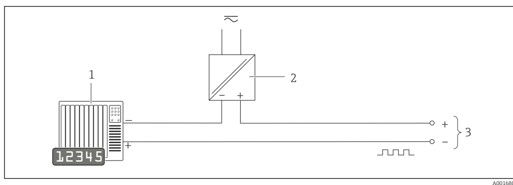
9 Exemple de raccordement pour sortie impulsion/fréquence (passive)
