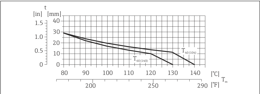
31 Epaisseur d'isolation maximale recommandée en fonction de la température du produit et ambiante
