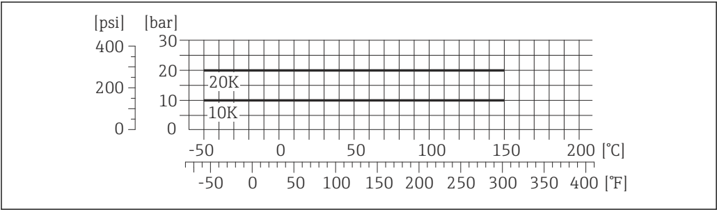
24 Avec matériau de bride 1.4404 (F316/F316L)
