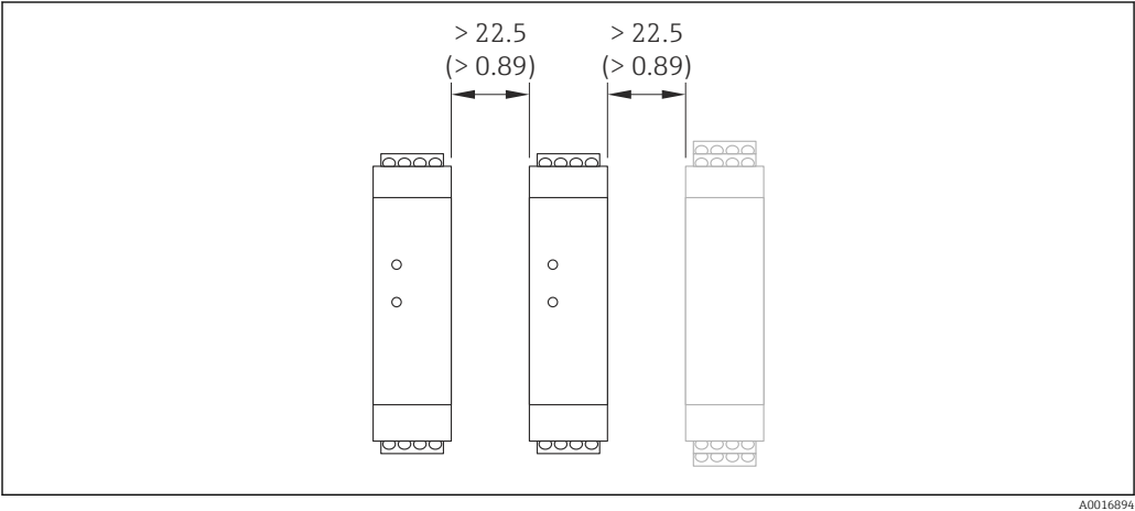
20 Ecart minimal avec d'autres barrières de sécurité Promass 100 ou d'autres modules. Unité de mesure mm (in)
