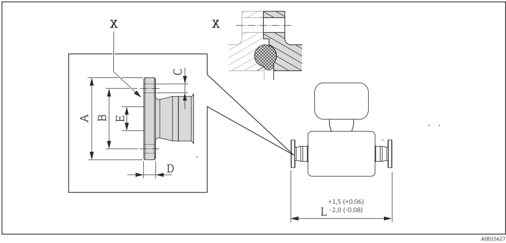
34 Détail X : raccord process asymétrique, la partie grisée fait partie de la livraison. Unité de mesure mm (in).
