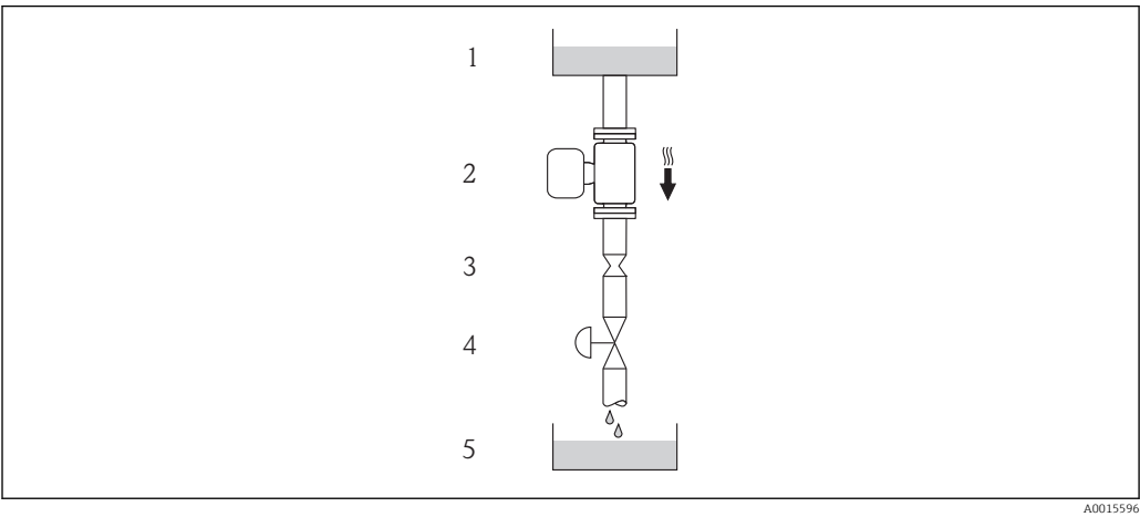
18 Montage dans un écoulement gravitaire (par ex. applications de dosage)
