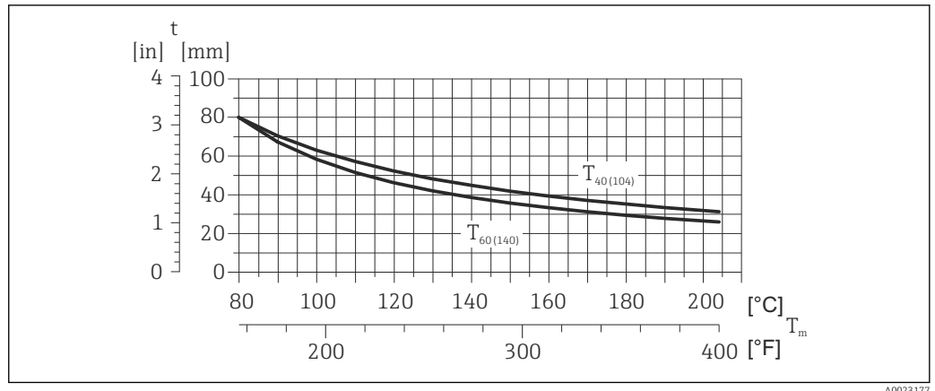
32 Epaisseur d'isolation maximale recommandée en fonction de la température du produit et ambiante
