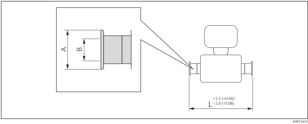
35 Unité de mesure mm (in)
