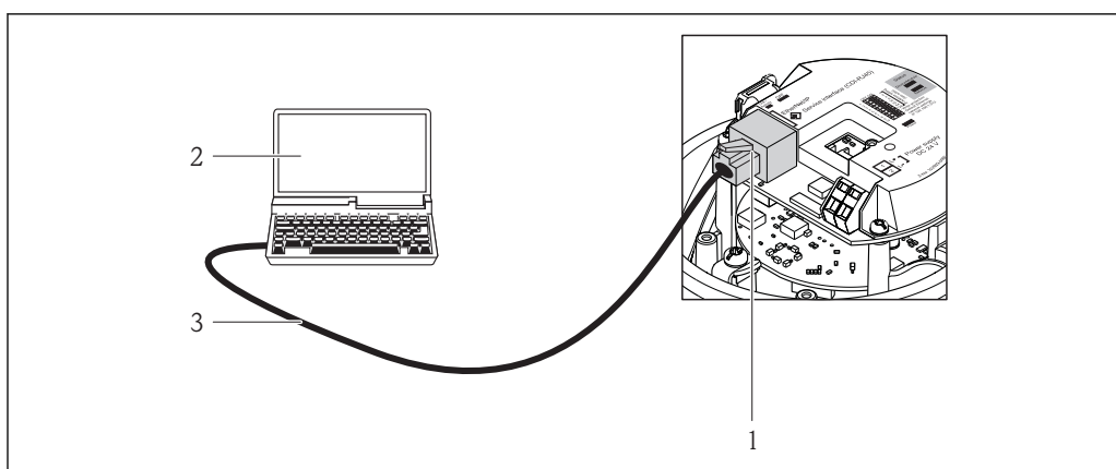
51 Connexion pour la variante de commande "Sortie", option R : PROFINET
