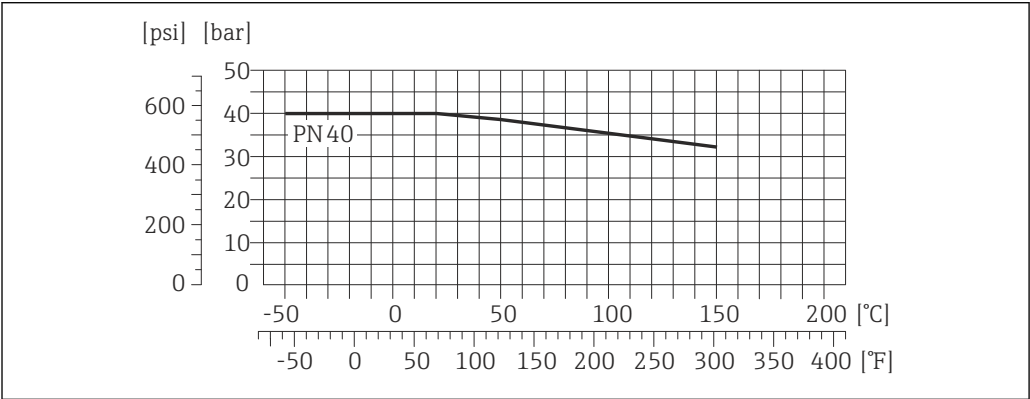
22 Avec matériau de bride 1.4404 (F316/F316L)
