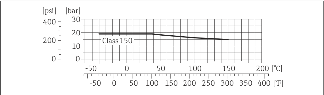
23 Avec matériau de bride 1.4404 (F316/F316L)
