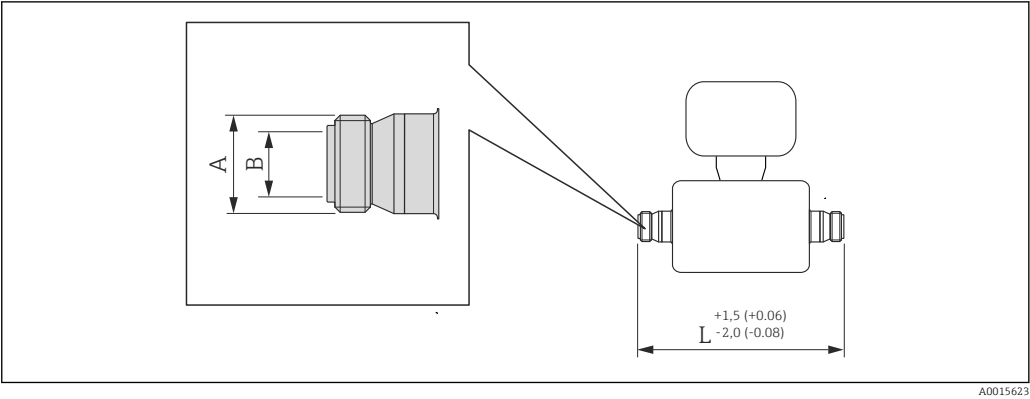
39 Unité de mesure mm (in)
