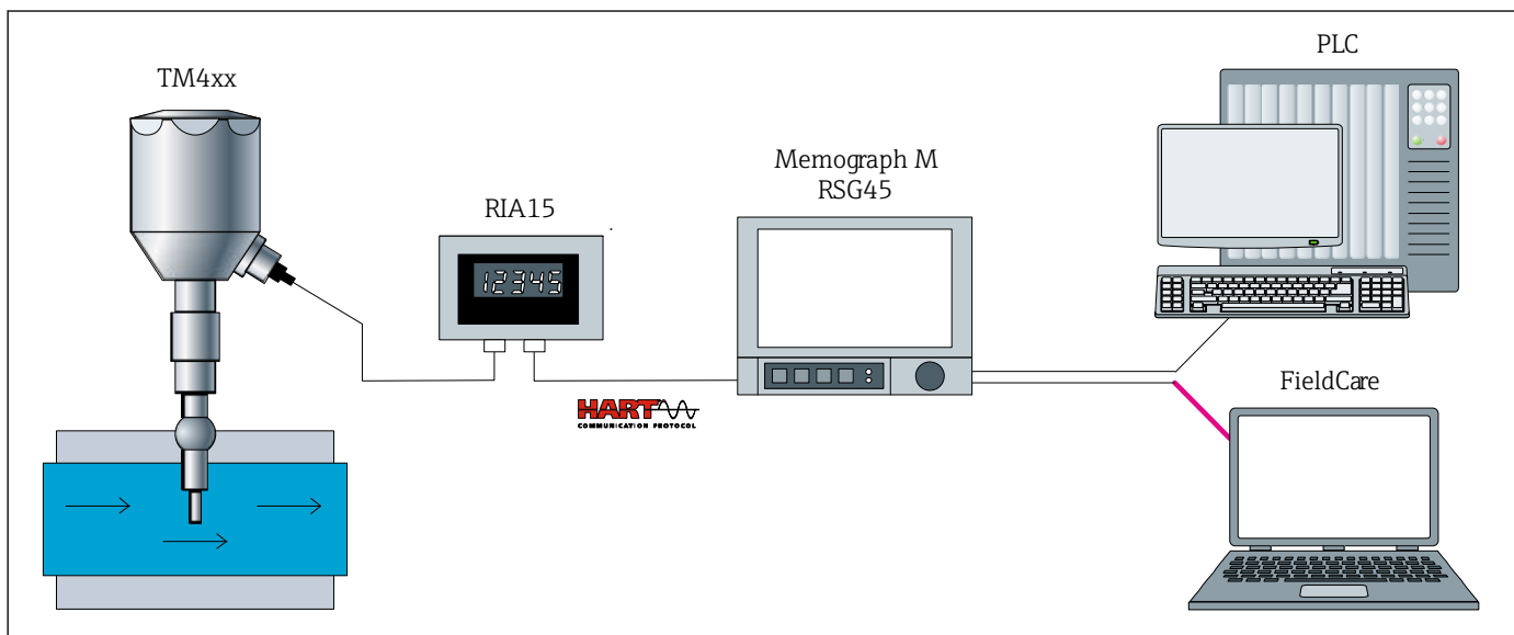
1 Exemple d'application, agencement du point de mesure avec d'autres composants Endress+Hauser
