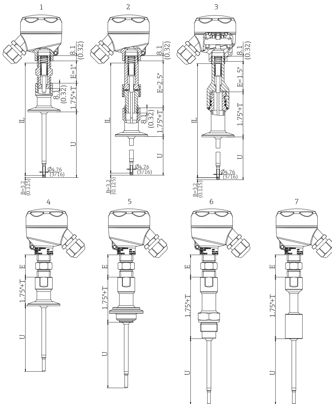
12 Protecteur avec raccord de tube NPT 1/2" et différentes versions de raccord process :
