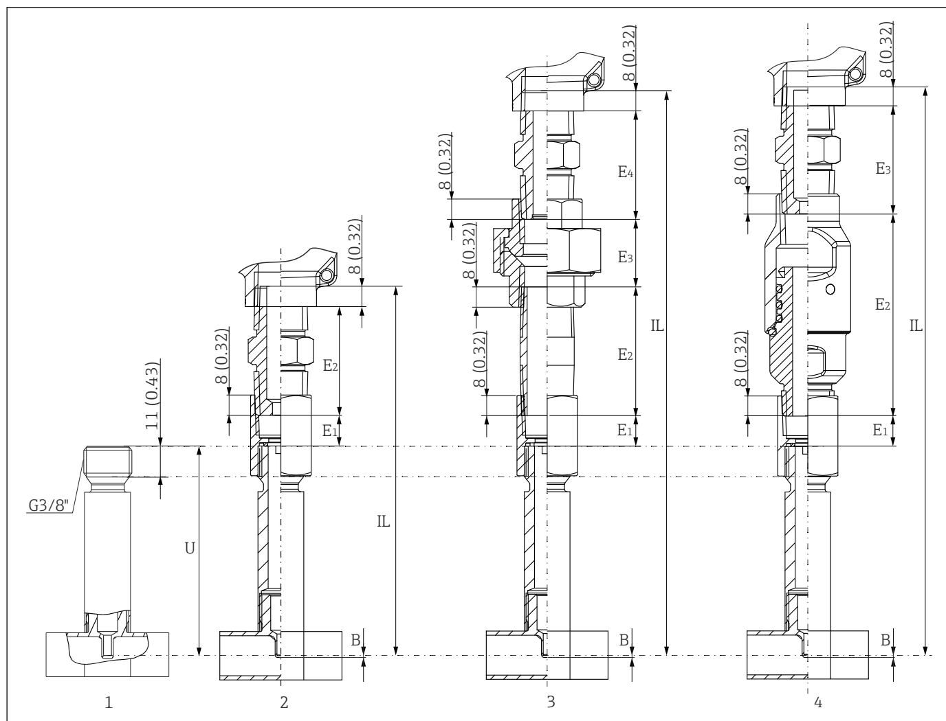
13 Protecteur en T selon DIN 11865 ou ASME BPE
