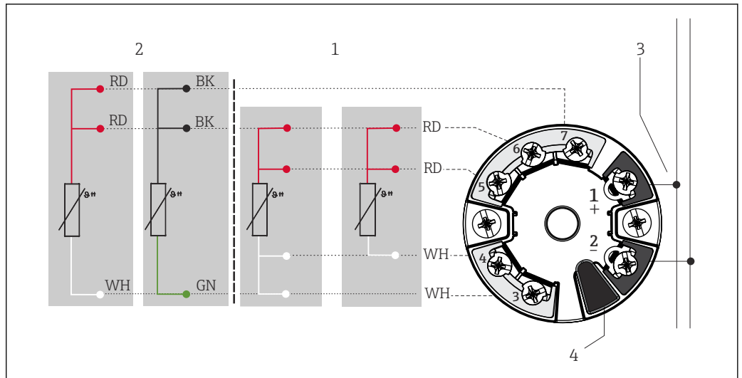
4 Transmetteur monté dans la tête de raccordement TMT8x (deux entrées).
