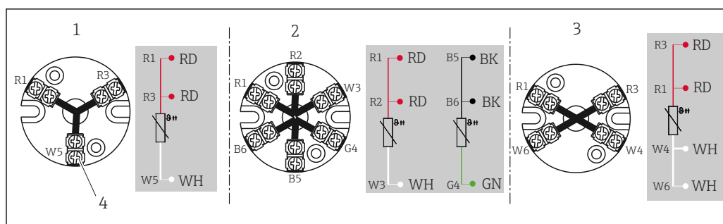
6 Bornier de raccordement monté
