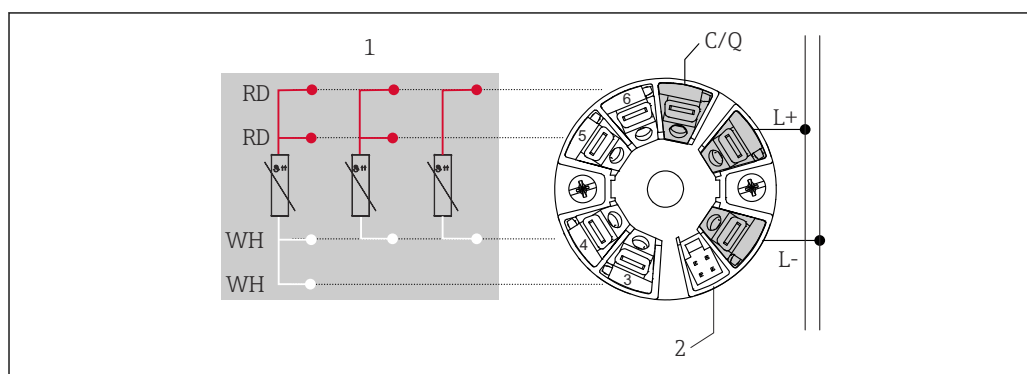
3 Transmetteur monté en tête iTEMP TMT36 (une entrée capteur)
