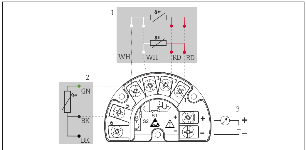
5 Transmetteur monté sur le terrain TMT162 (deux entrées)
