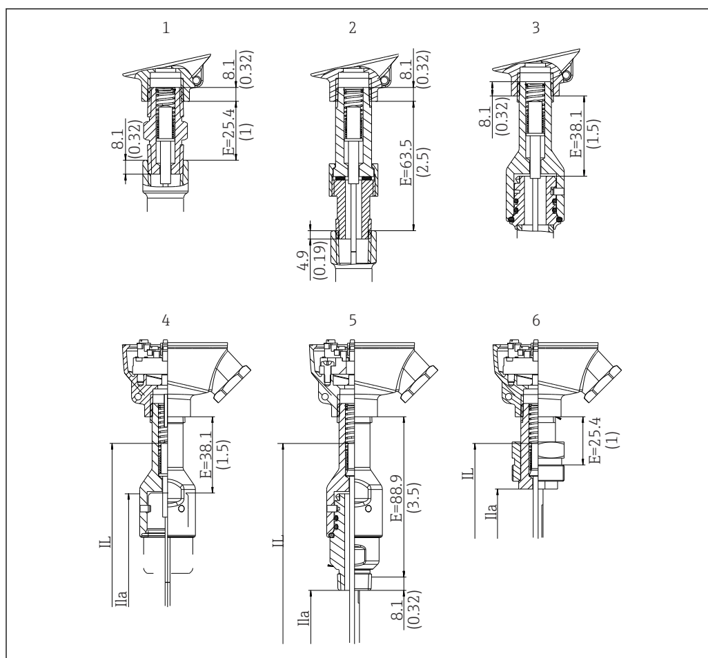
15 Dimensions du tube prolongateur, différentes versions, chacune avec filetage 1/2" NPT vers la tête de raccordement
