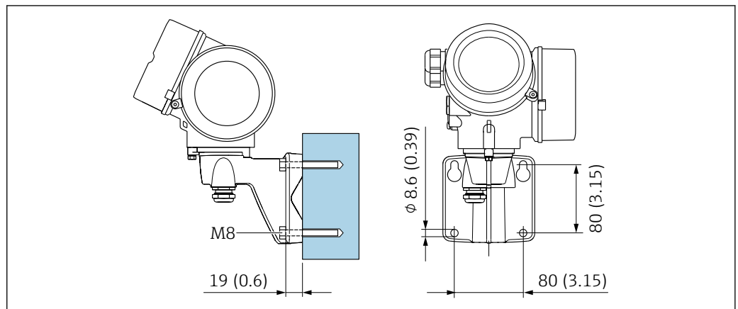
図 13 mm (in)
