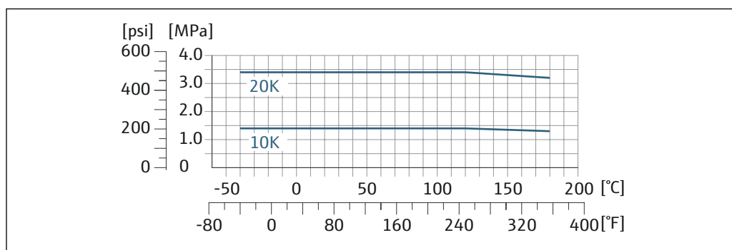
図 18 フランジ接続材質：ステンレス、複数の認証、1.4404、SUS F316 相当または F316L 相当
