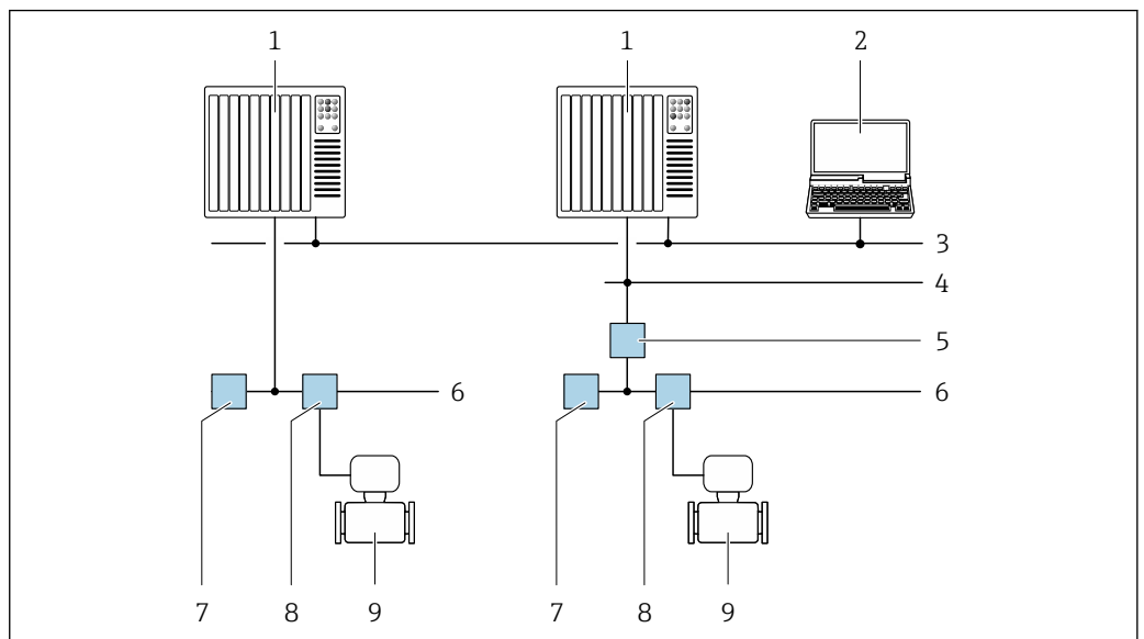
図 28 FOUNDATION Fieldbus ネットワークを介したリモート操作のオプション
