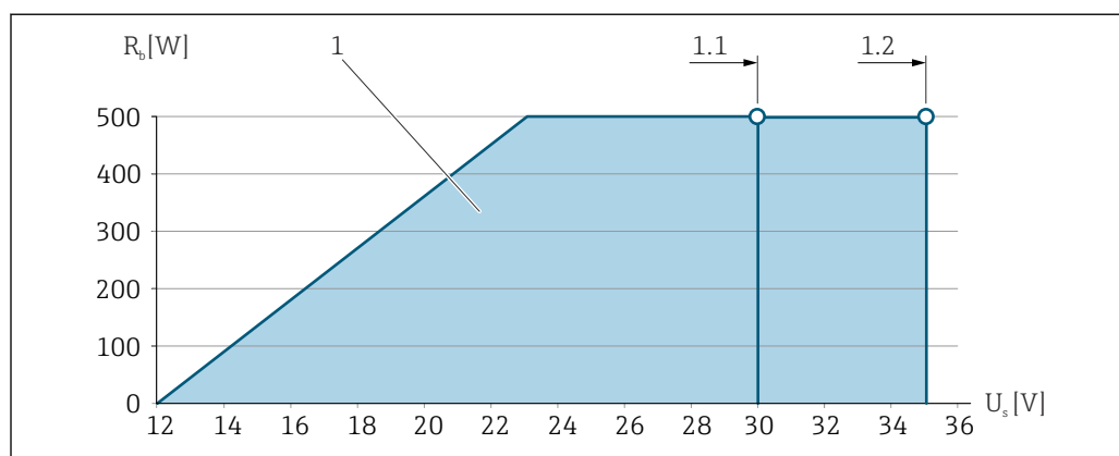
図 2 現場表示器なしの一体型の負荷
