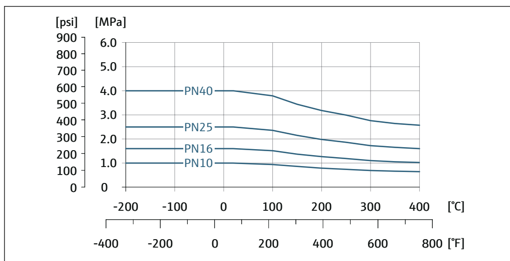
図 16 フランジ接続材質：ステンレス、複数の認証、1.4404、SUS F316 相当または F316L 相当
