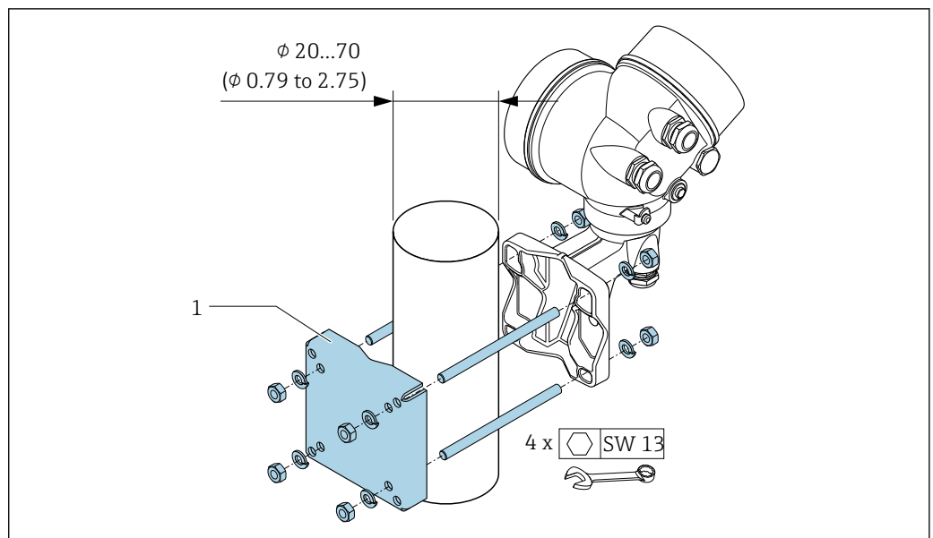
図 14 mm (in)
