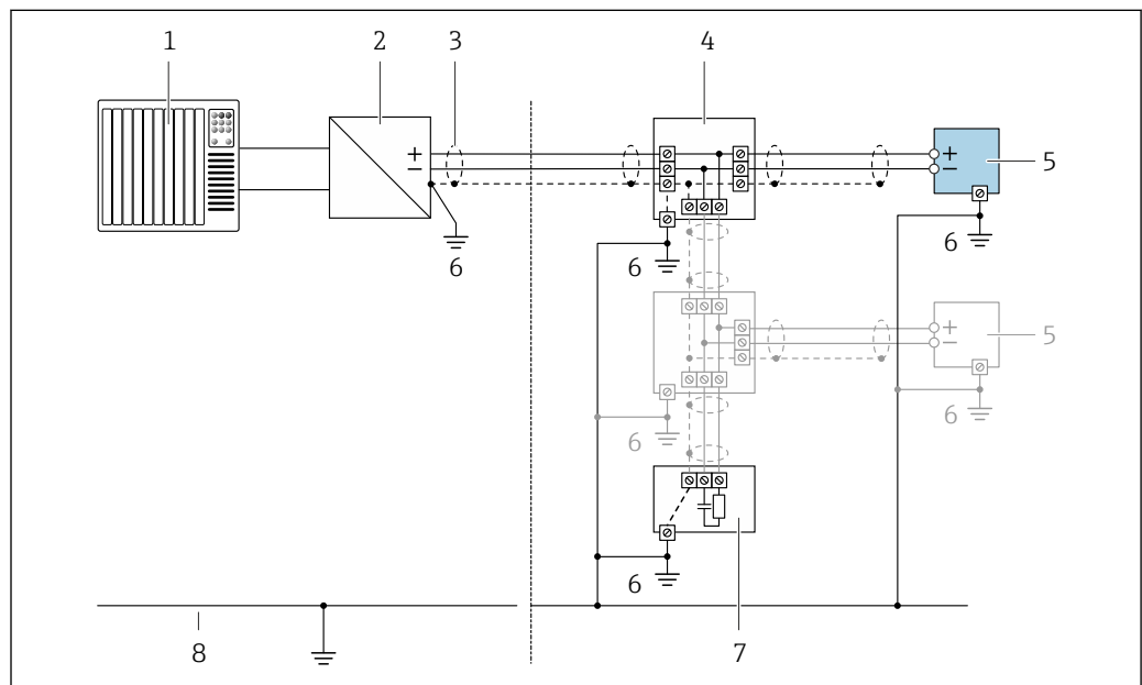
図 10 FOUNDATION Fieldbus の接続例
