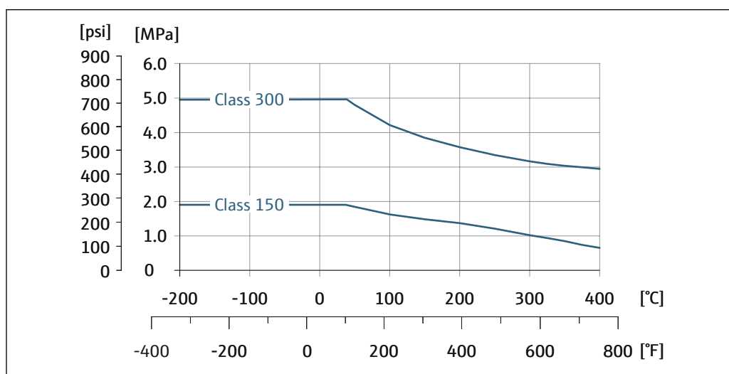
図 17 フランジ接続材質：ステンレス、複数の認証、1.4404、SUS F316 相当または F316L 相当
