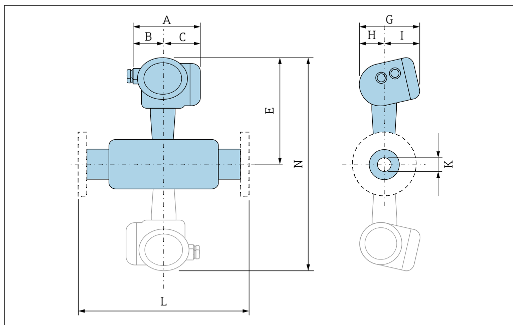
図 22 灰色表示：デュアルセンサタイプ
