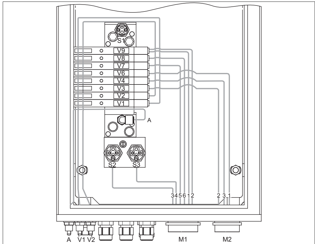
Fig. 70: Pneumatic
