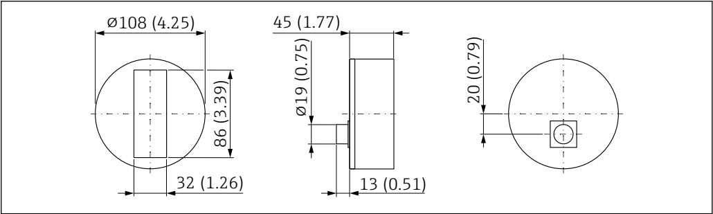
14 短型圆形传感器的外形尺寸示意图。测量单位 mm (in)
