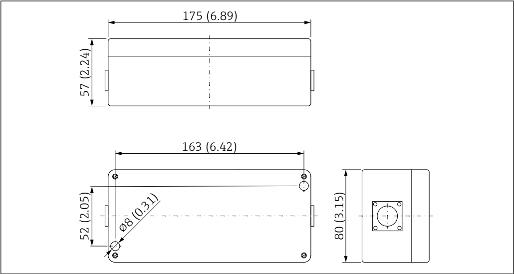
19 分体式电子模块外壳的外形尺寸示意图。测量单位 mm (in)
