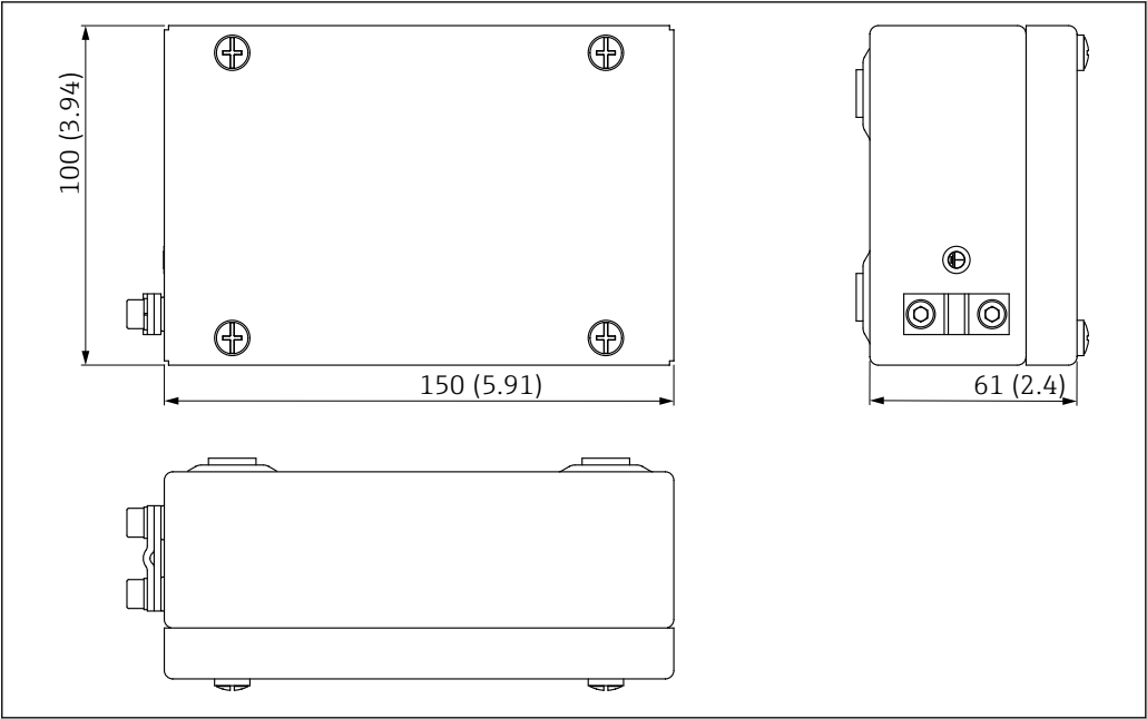
18 ATEX 防爆型电子部件腔的外形尺寸示意图。测量单位 mm (in)
