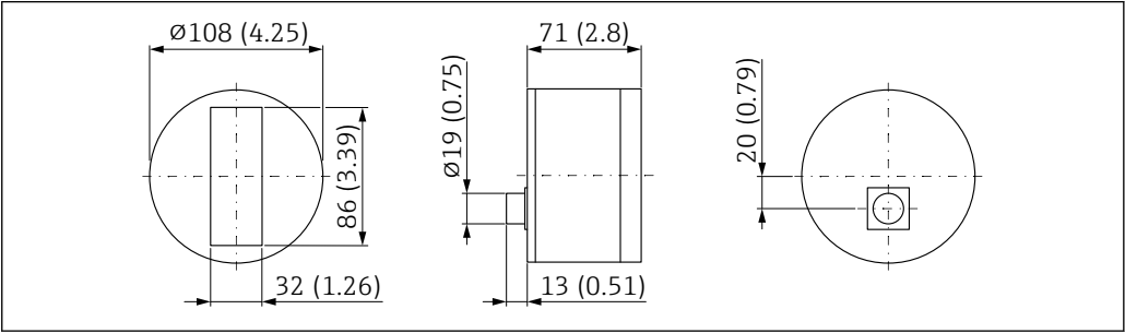
15 中长型圆形传感器的外形尺寸示意图。测量单位 mm (in)
