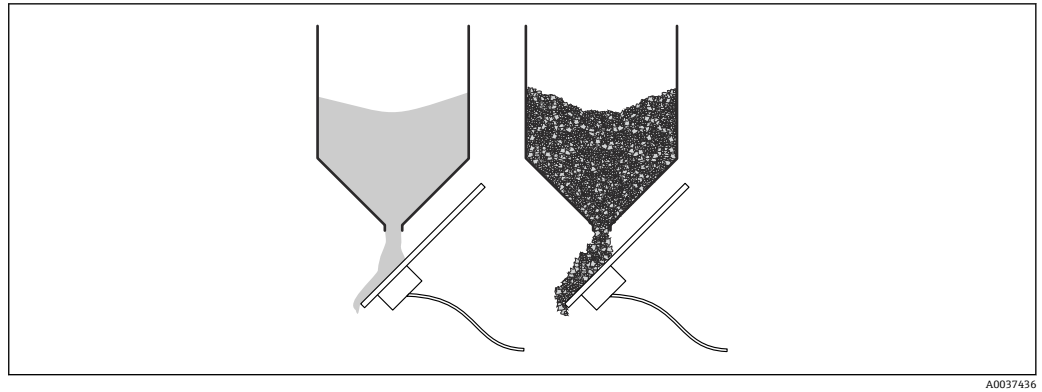
图 5 在料仓出料口下方安装用于测量固体散料的圆形传感器
