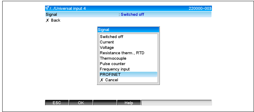
5 Configuración de PROFINET como señal de entrada
