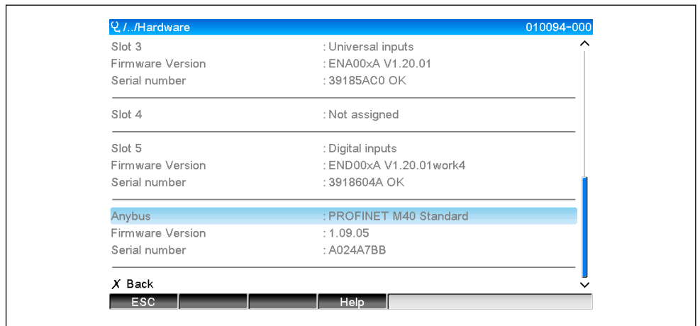
3 Información sobre el módulo PROFINET detectado en "Hardware"
