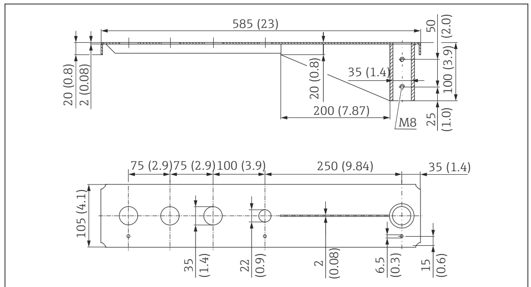
17 Dimensioni. Unità di misura mm (in)
