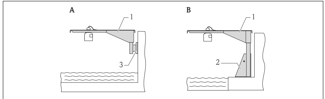
16 Montaggio del sensore con braccio a sbalzo
