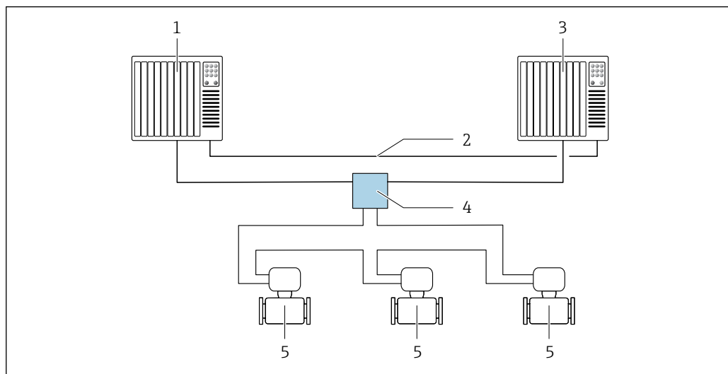
28 Exemple de configuration d'un système redondant (S2) : topologie en anneau
