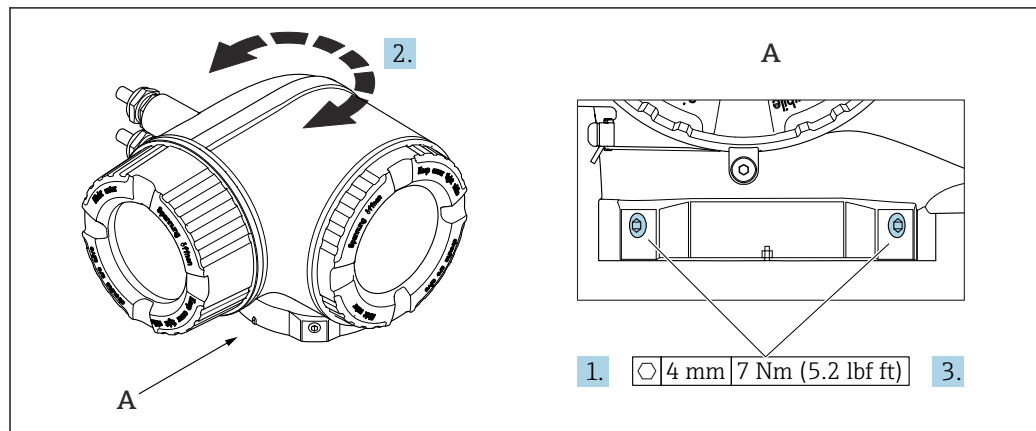
11 Boîtier Ex
