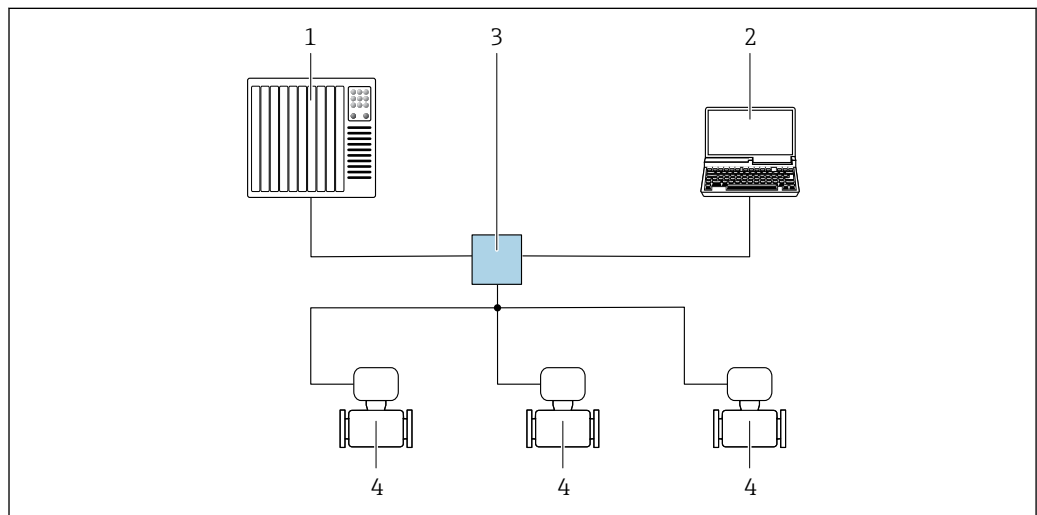
25 Options de configuration à distance via réseau PROFINET : topologie en étoile
