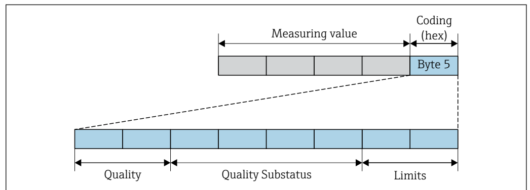
34 Structure de l'octet d'état
