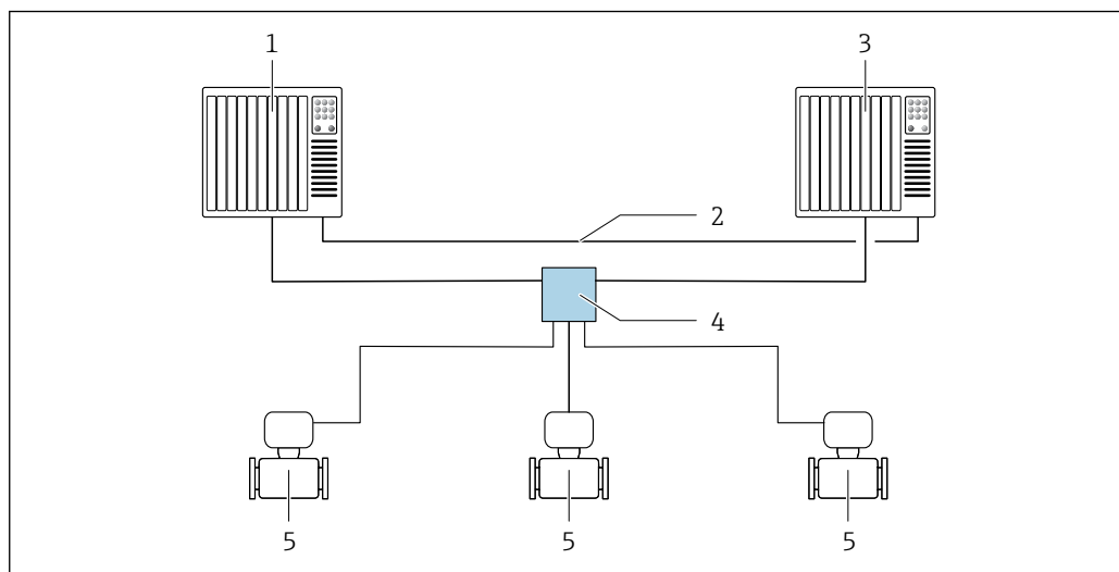
29 Exemple de configuration d'un système redondant (S2) : topologie en étoile
