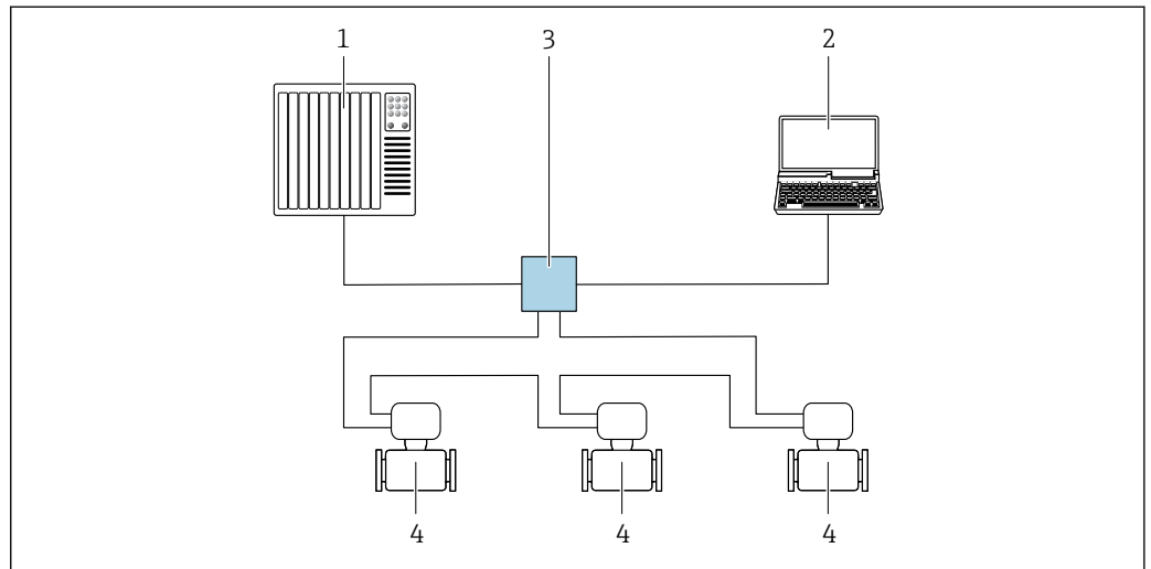
26 Options de configuration à distance via réseau PROFINET : topologie en anneau
