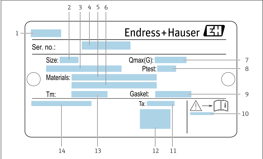
1 传感器的铭牌示意图
