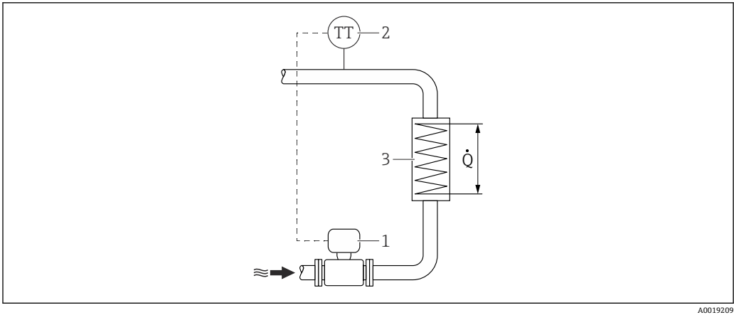
图 5 蒸汽和水热量差值测量示意图
