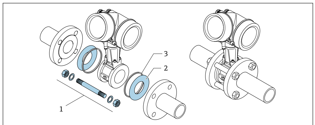
图 6 夹持式仪表的安装套件
