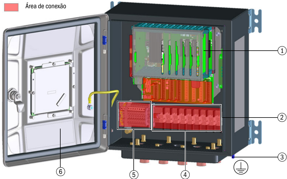
Figura 75 Área de conexão e eletrônica interna da interface unit
