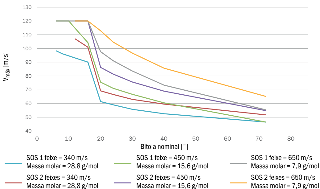
Figura 128 Exemplo V_{\max} de versões cross-duct de 1 feixe e 2 feixes dependentes da velocidade do som (SOS)
