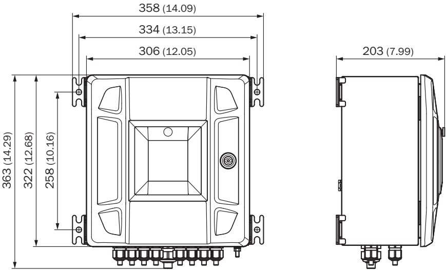
Figura 136 Interface unit zona 2 (dimensões em mm (pol))
