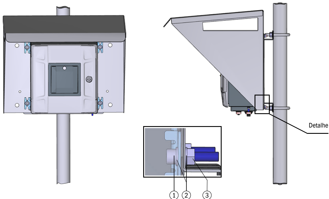
Figura 70 Interface unit zona 2 montada com proteção contra intempéries
