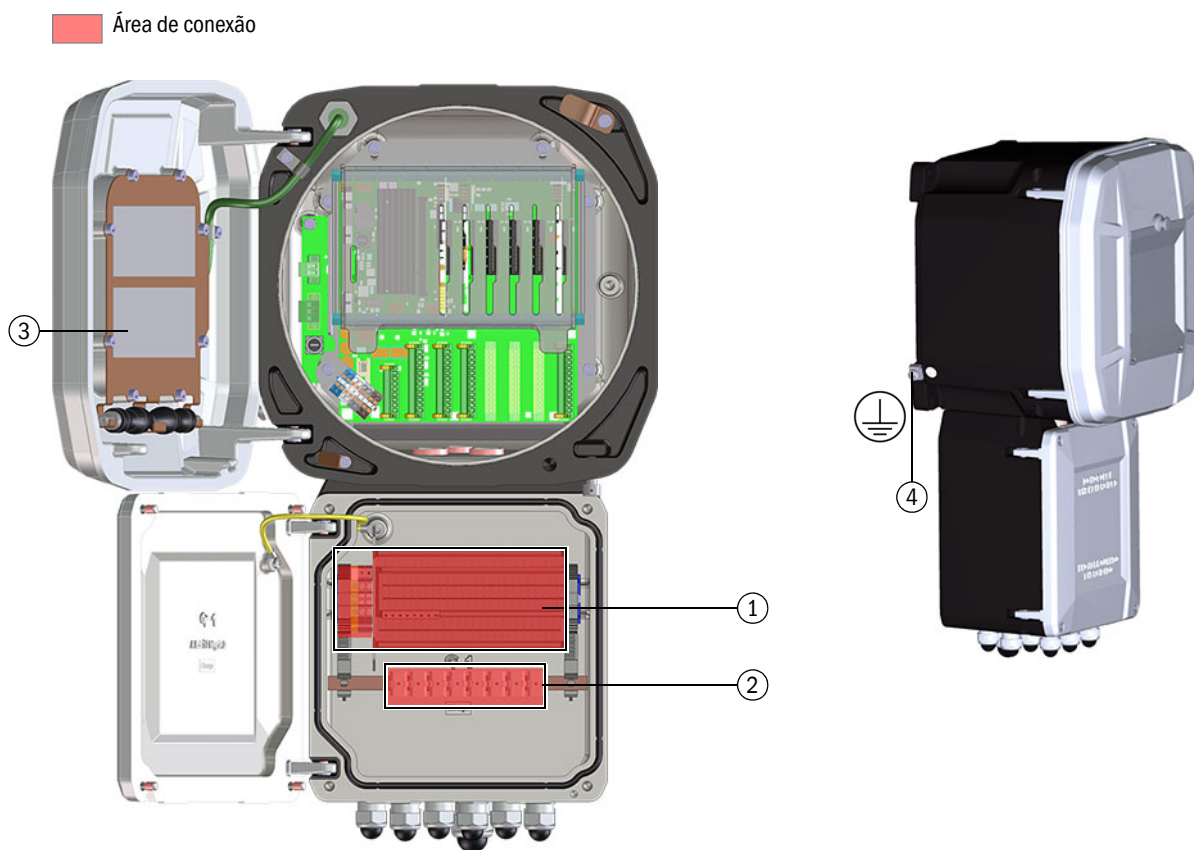
Figura 77 Área de conexão e eletrônica interna da interface unit zona 1 Ex d e
