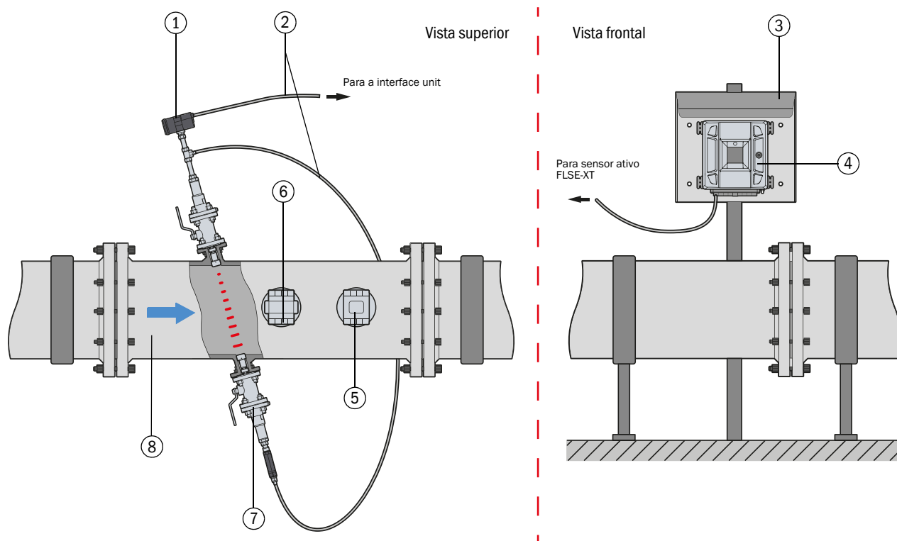
Figura 2 Visão geral do sistema FLOWSIC100 Flare-X T
