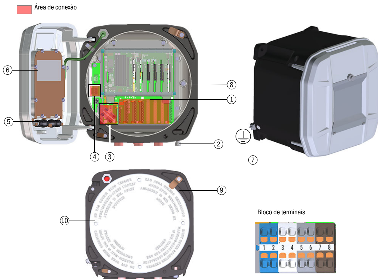
Figura 76 Área de conexão e eletrônica interna da interface unit zona 1 Ex d
