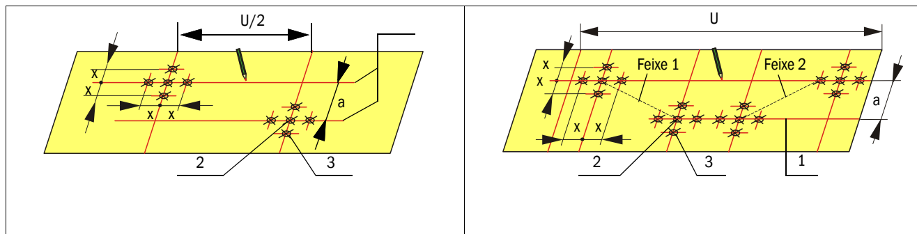
Figura 22 Marcar as posições do bocal na tubulação para versões cross-duct
