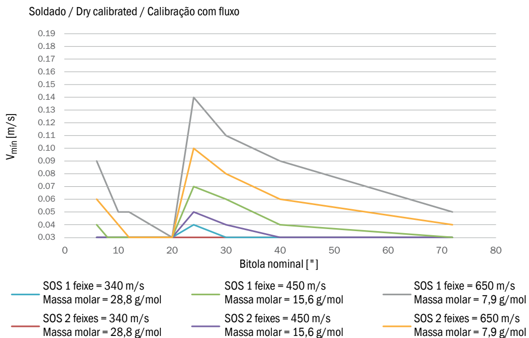
Figura 129 V_{\min} com incerteza 20% de soluções de 1 feixe e 2 feixes dependentes da velocidade do som (SOS)
