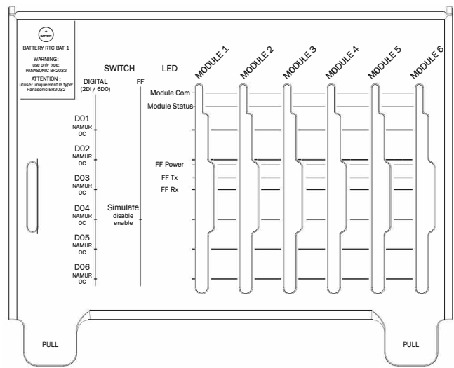
Figura 88 Tampa da eletrônica
