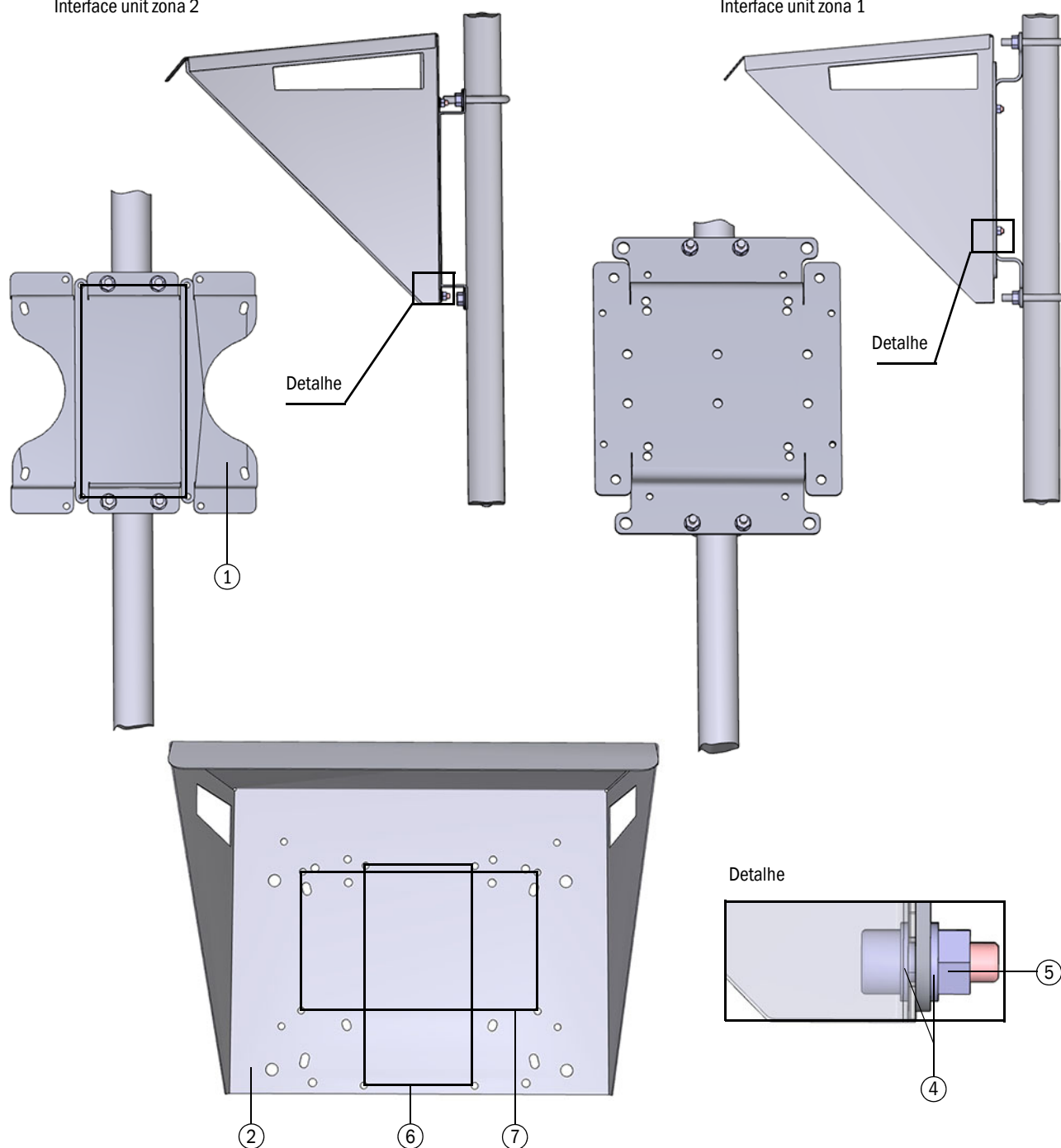
Figura 68 Instalação da proteção contra intempéries na placa de montagem Interface unit zona 2
