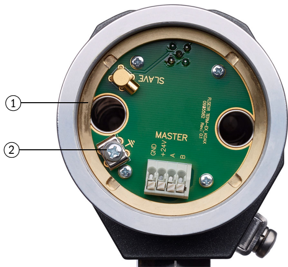
Figura 44 Caixa de terminais da unidade emissor / receptor FLSE100-XT com eletrônica (sensor ativo)
