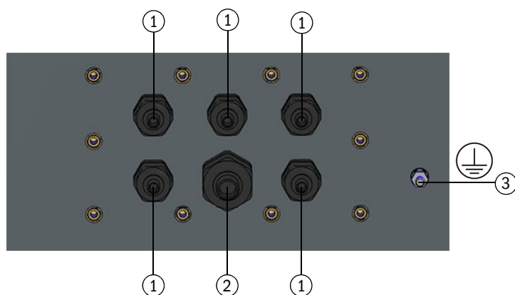
Figura 54 Prensa cabos métricos (opcionalmente disponível com 9 prensa cabos)
