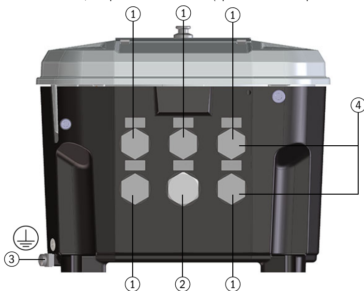
Figura 58 Caixa Ex d, tampão roscado métrico (opcionalmente disponível com 9 tampões roscados)
