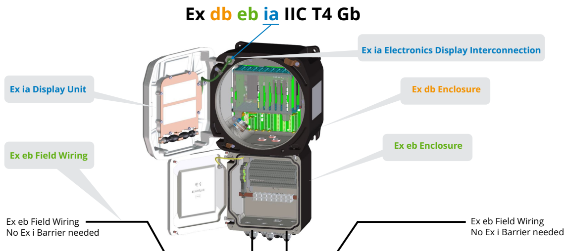
Figura 154 Interface unit zona 1 Ex d e
