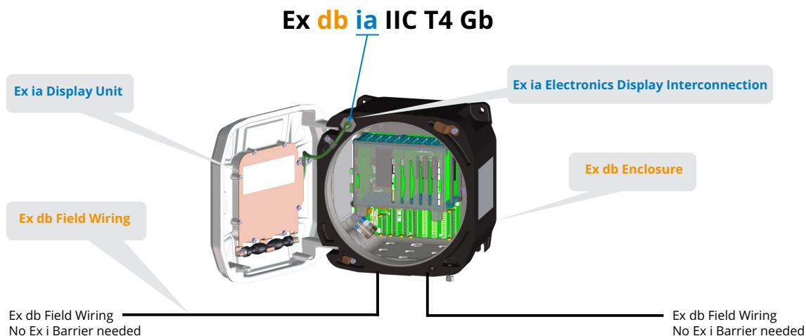
Figura 153 Interface unit zona 1 Ex d
