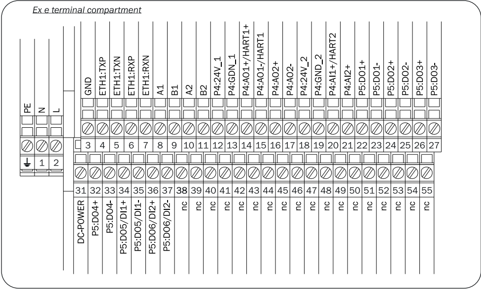
Figura 86 Exemplo configuração AC (variante A)
