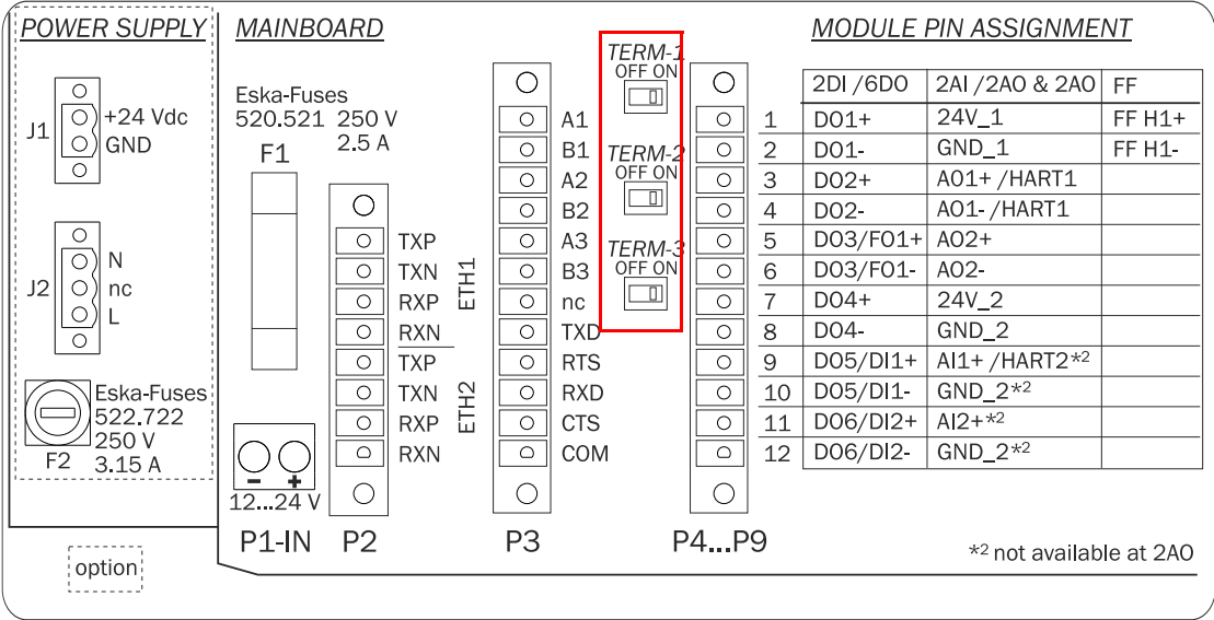
Figura 92 Posição das chaves de terminação
