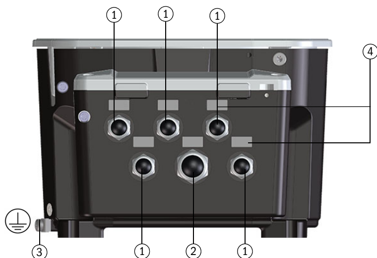
Figura 60 Caixa Ex d e, prensa cabos métricos (opcionalmente disponível com 9 prensa cabos)
