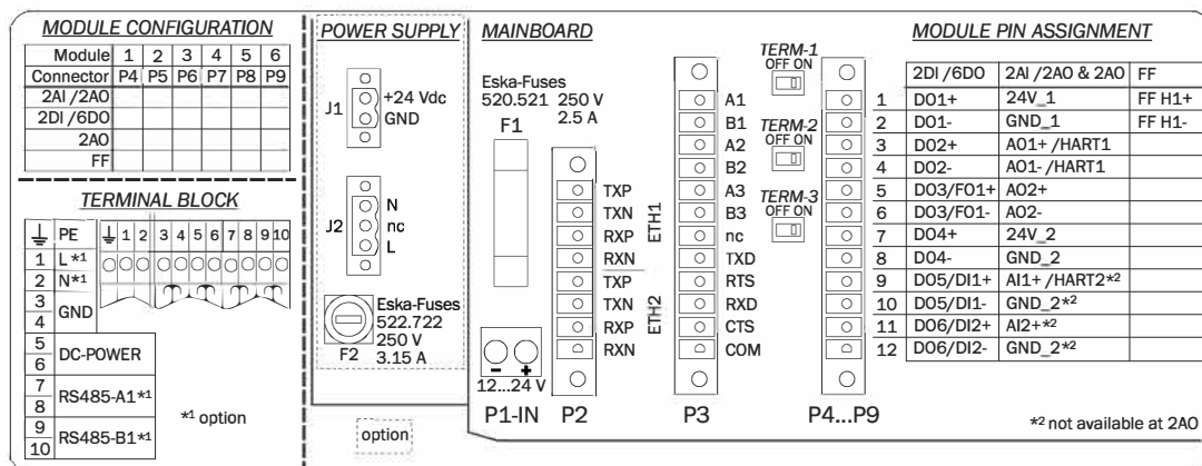
Figura 81 Diagrama de conexões
