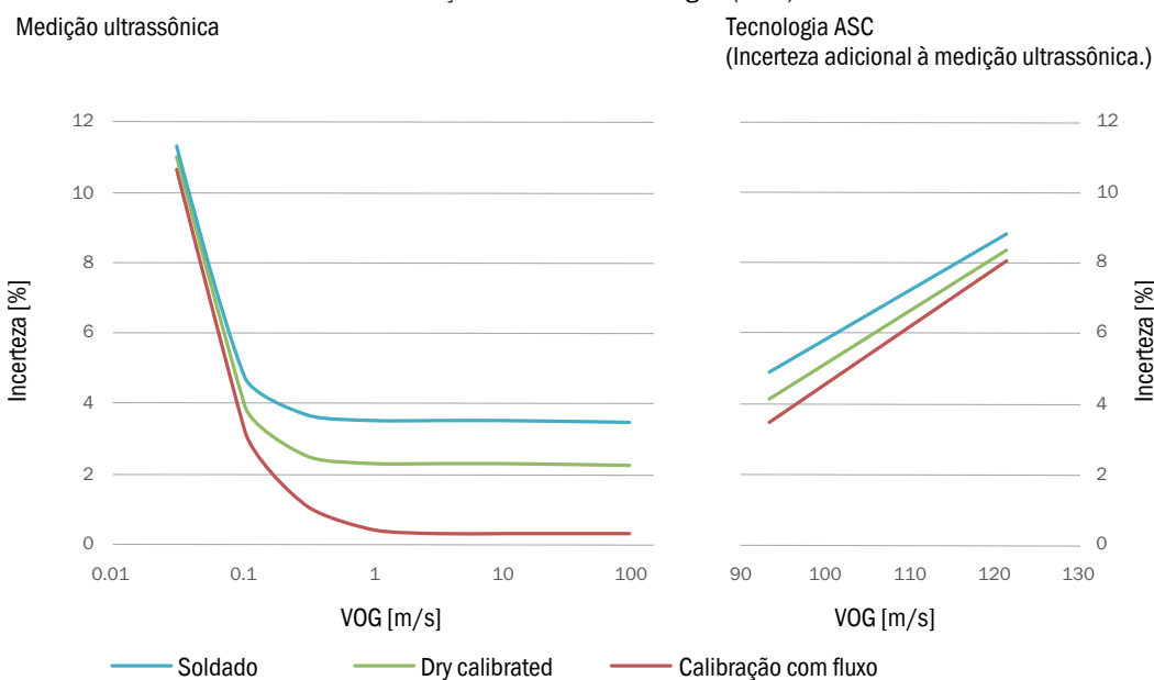
Figura 130 Incerteza da vazão volumétrica em função da velocidade do gás (VOG)
