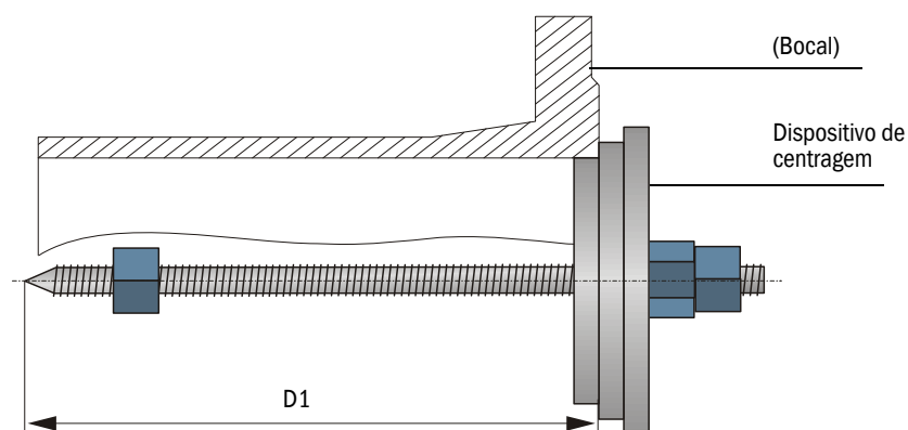
Figura 27 Determinar o comprimento efetivo do bocal
