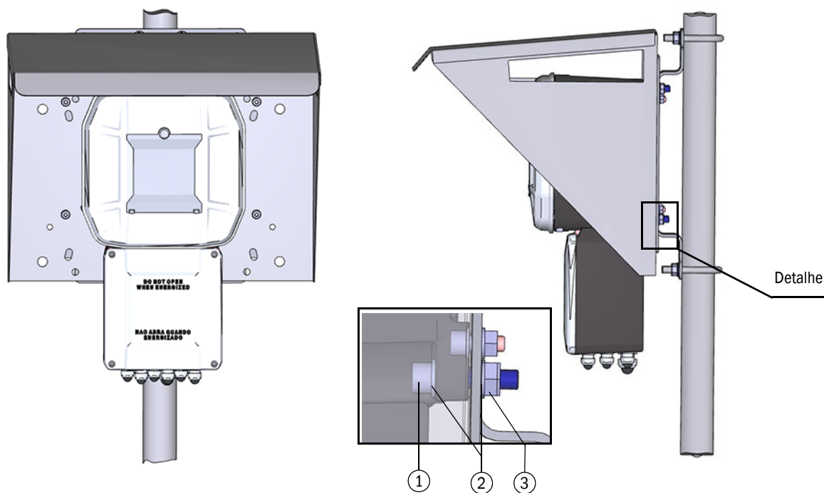
Figura 71 Interface unit zona 1 montada com proteção contra intempéries
