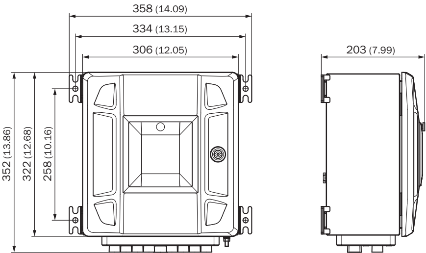
Figura 137 Interface unit cl. 1 div. 2 (dimensões em mm (pol))
