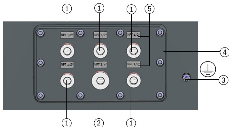
Figura 55 Tampão roscado NPT (opcionalmente disponível com 9 entradas de cabos)
