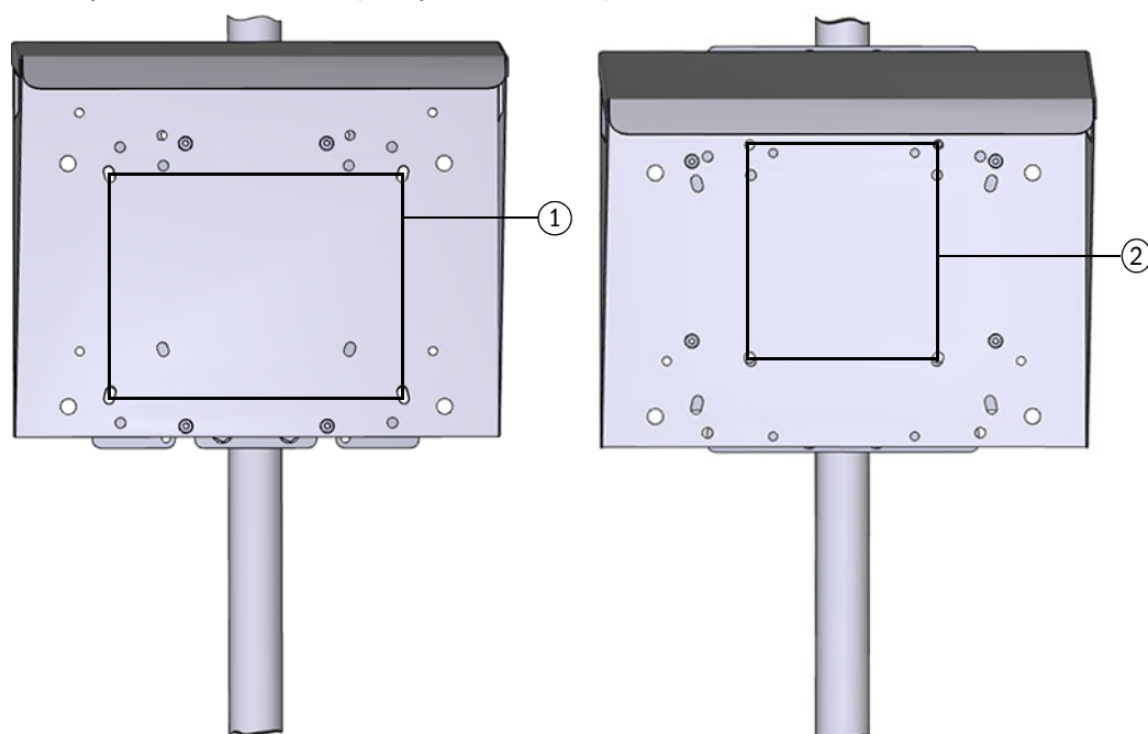
Figura 69 Instalação da interface unit na proteção contra intempéries
