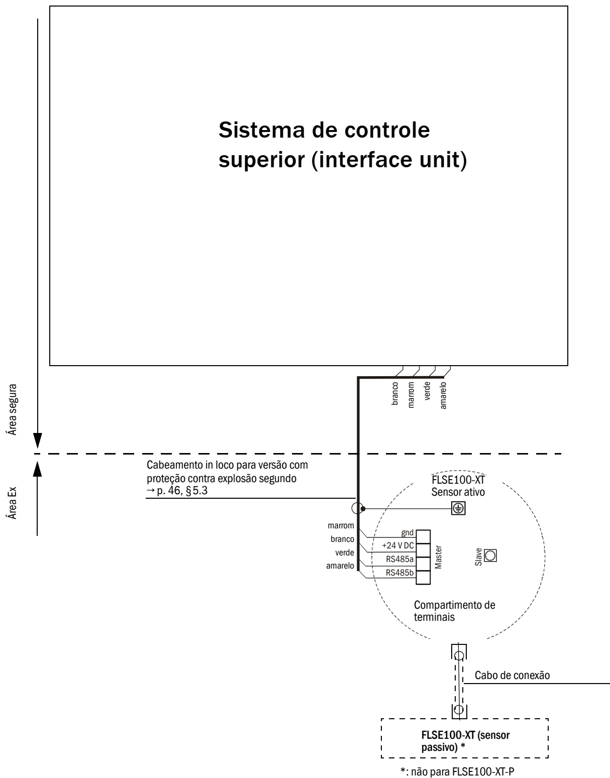
Figura 45 Cabeamento das unidades emissor / receptor
