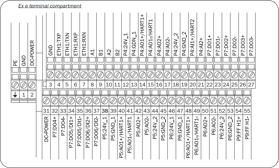
Figura 87 Exemplo configuração DC (variante L)
