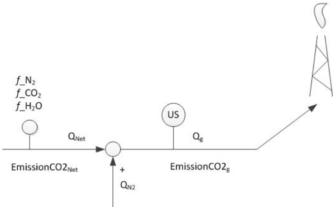
Figura 111 Modo de funcionamento da compensação de nitrogênio
