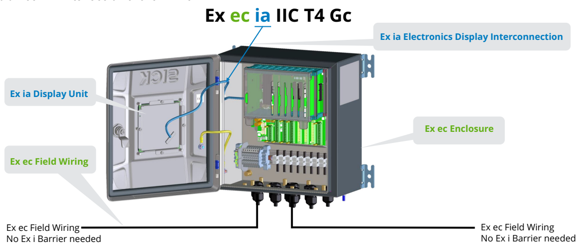
Figura 155 Interface unit zona 2 Ex e
