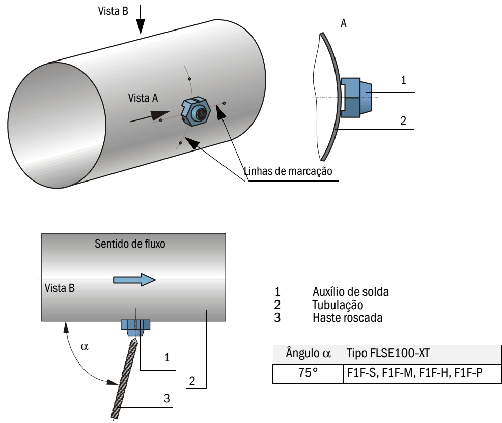
Figura 25 Posicionamento do auxílio de solda
