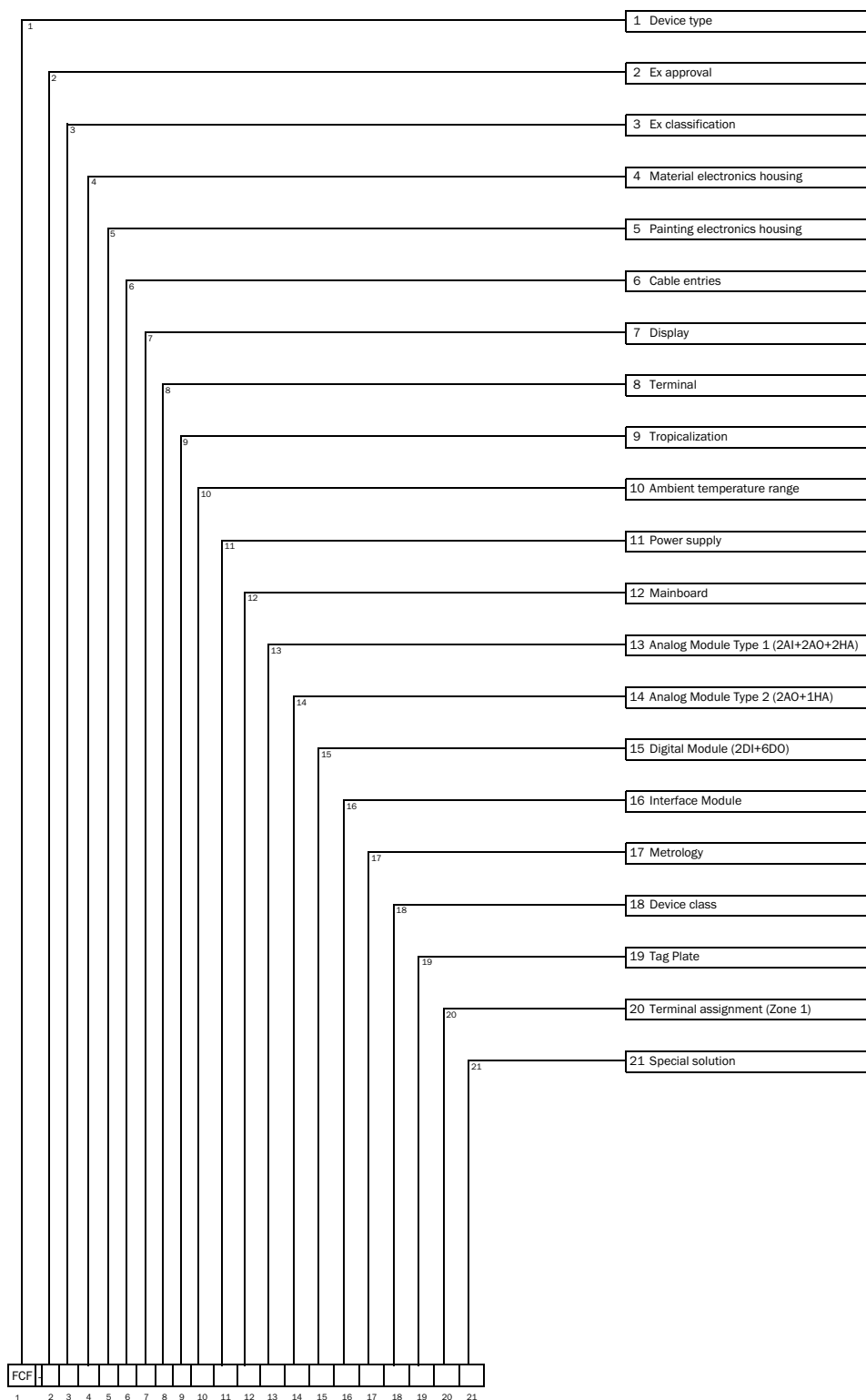
Figura 151 Chave de codificação da interface unit (visão geral)
