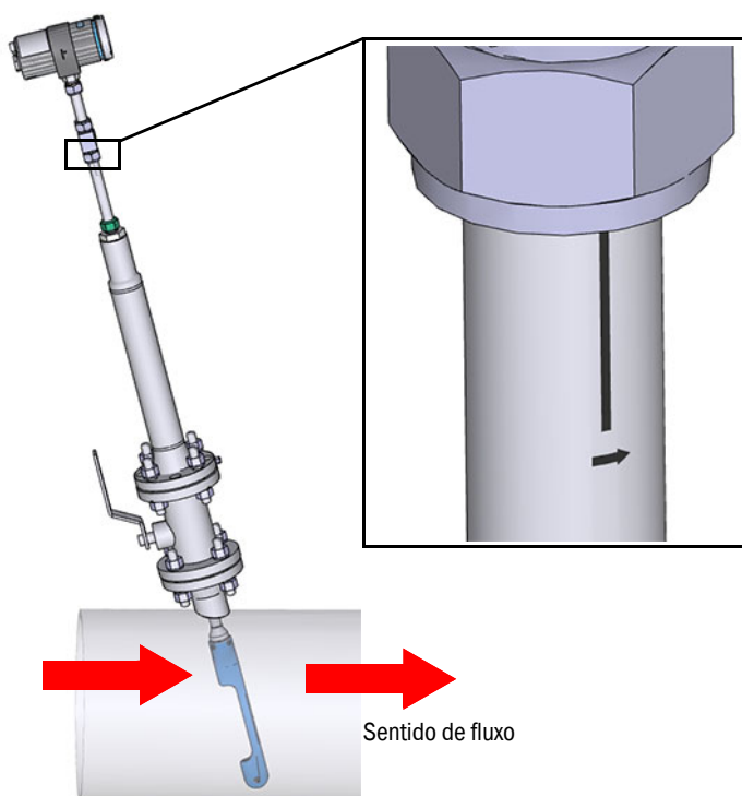
Figura 39 Marcas na versão sonda F1F-P
