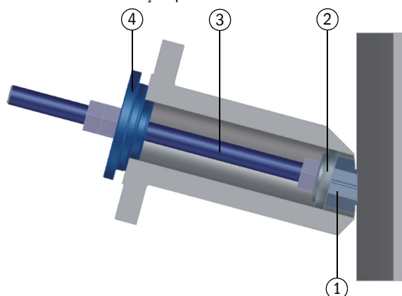
Figura 18 Ferramenta de instalação para bocais
