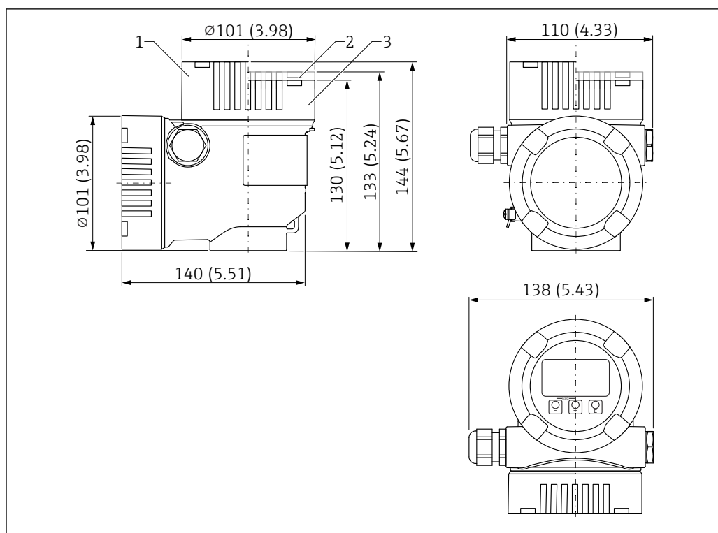
39 Dimensões; invólucro de compartimento duplo em formato de L, alumínio, revestido; incl. acoplamento e conector M20, plástico. Unidade de medida mm (in)
