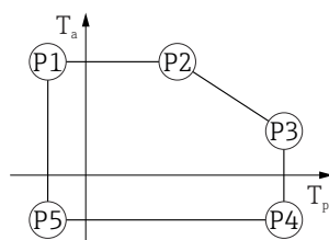
■ 25 Invólucro de alumínio, revestido; temperatura do processo -40 para +280 °C (-40 para +536 °F)
