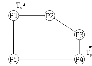
■ 18 Invólucro de plástico: temperatura do processo -40 para +280 °C (-40 para +536 °F)
