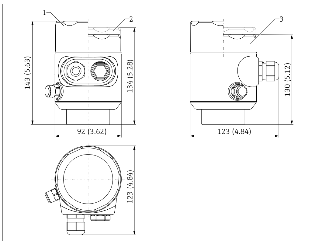
37 Dimensões; invólucro de compartimento único, 316 L, sanitário; incl. acoplamento e conector M20, plástico. Unidade de medida mm (in)
