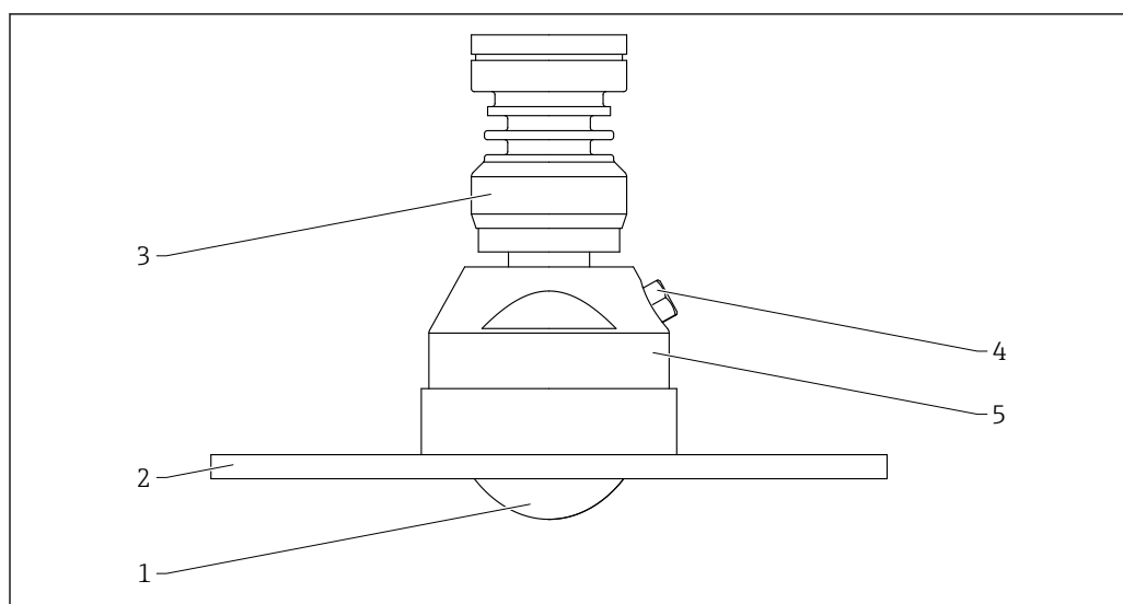
64 Material; antena, montagem flush, 80 mm (3 in), com flange UNI e conexão de ar de purga. Unidade de medida mm (in)
