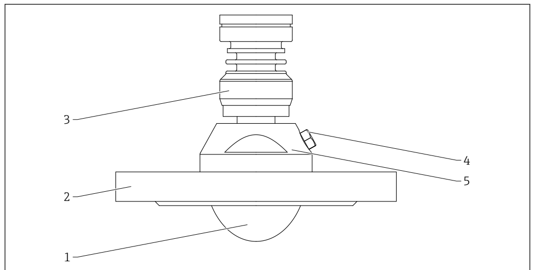
63 Material; antena, montagem flush, 80 mm (3 in), com flange e conexão de ar de purga. Unidade de medida mm (in)
