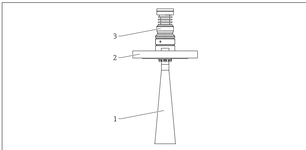
60 Material, antena piramidal 65 mm (2.6 in). Unidade de medida mm (in)
