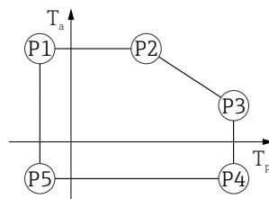
28 Invólucro 316L; temperatura do processo: -40 para +150 °C (-40 para +302 °F)
