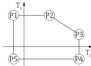
27 Invólucro 316L; temperatura do processo -40 para +80 °C (-40 para +176 °F)
