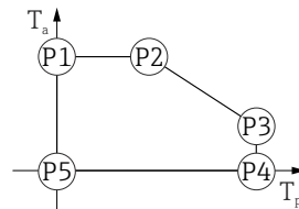
21 Invólucro de plástico; temperatura de processo 0 para +450 °C (+32 para +842 °F) com aprovação CSA C/US
