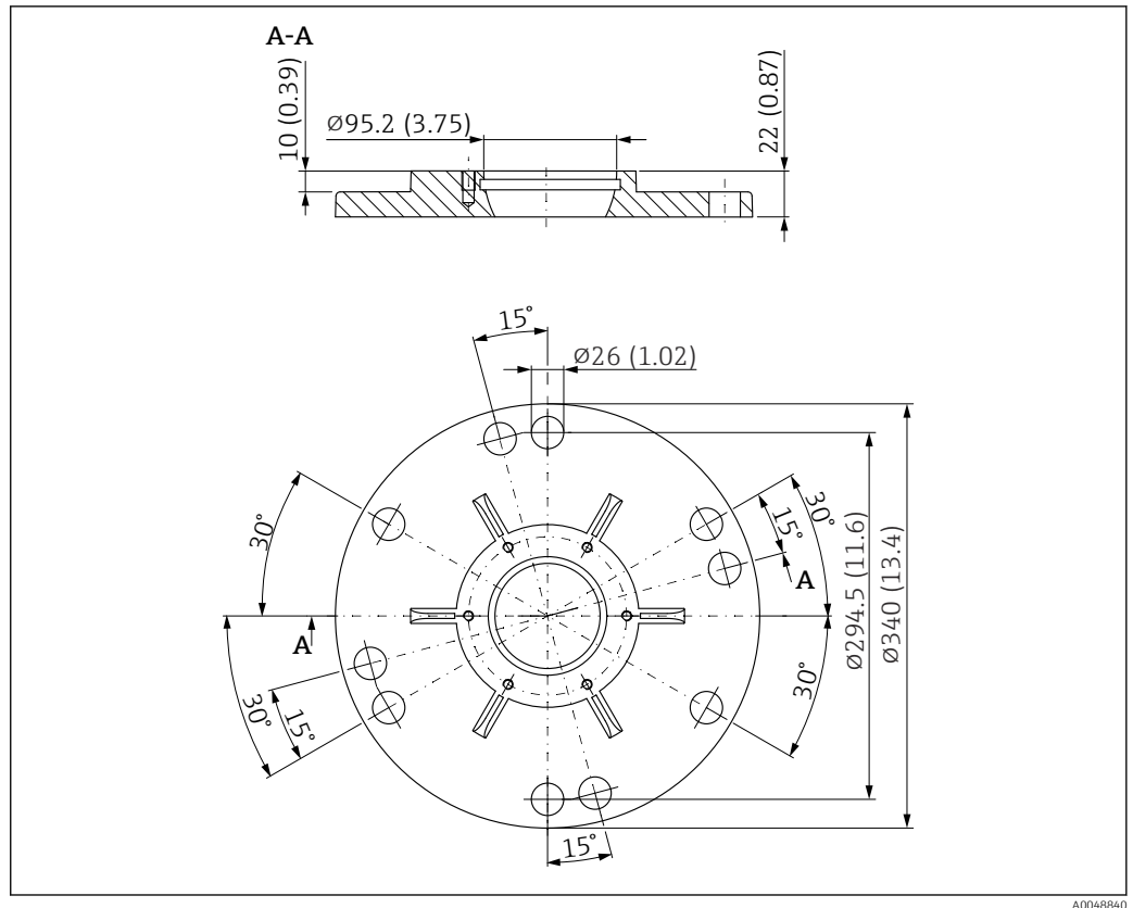
45 Dimensões da flange UNI 8"/DN200/200A para antenas com unidade de alinhamento. Unidade de medida mm (in)
