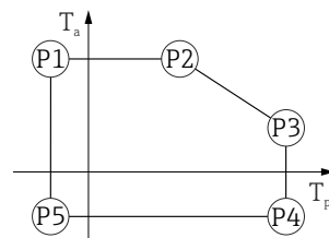
22 Invólucro de alumínio; revestido; temperatura do processo -40 para +80 °C (-40 para +176 °F)
