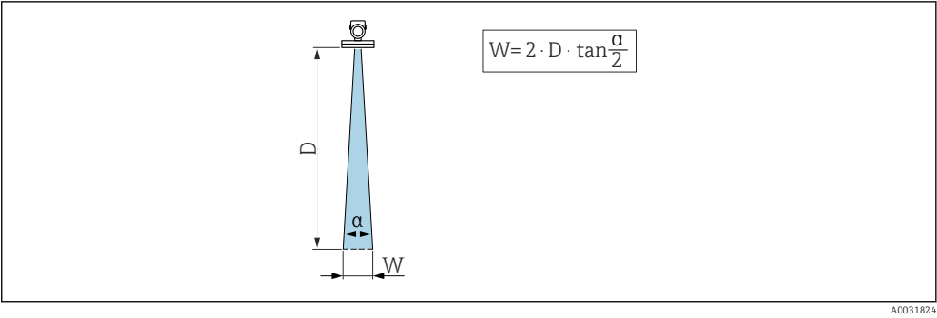
11 Relação entre o ângulo do feixe \alpha , a distância D e o diâmetro do feixe W
