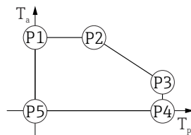
■ 19 Invólucro de plástico; temperatura de processo 0 para +280 °C (+32 para +536 °F) com aprovação CSA C/US
