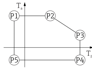
20 Invólucro de plástico: temperatura do processo -40 para +450 °C (-40 para +842 °F)
