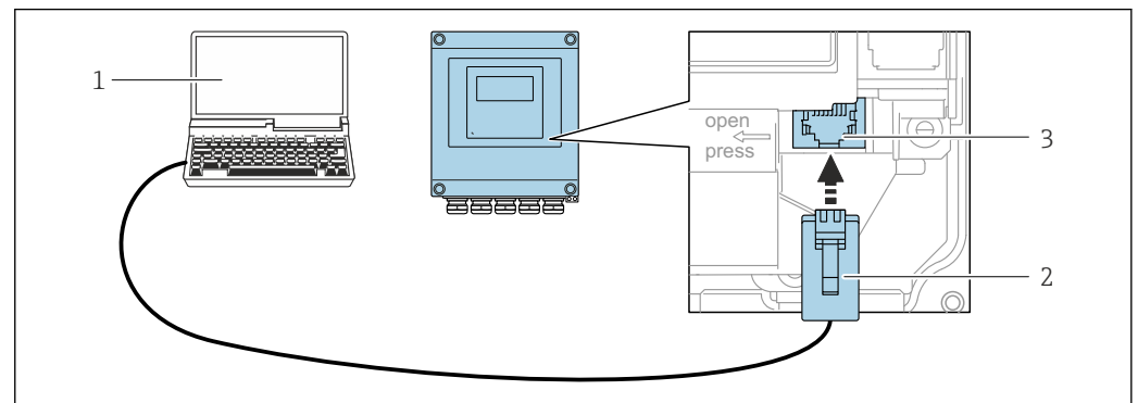
46 Conexão através de Interface de operação (CDI-RJ45)
