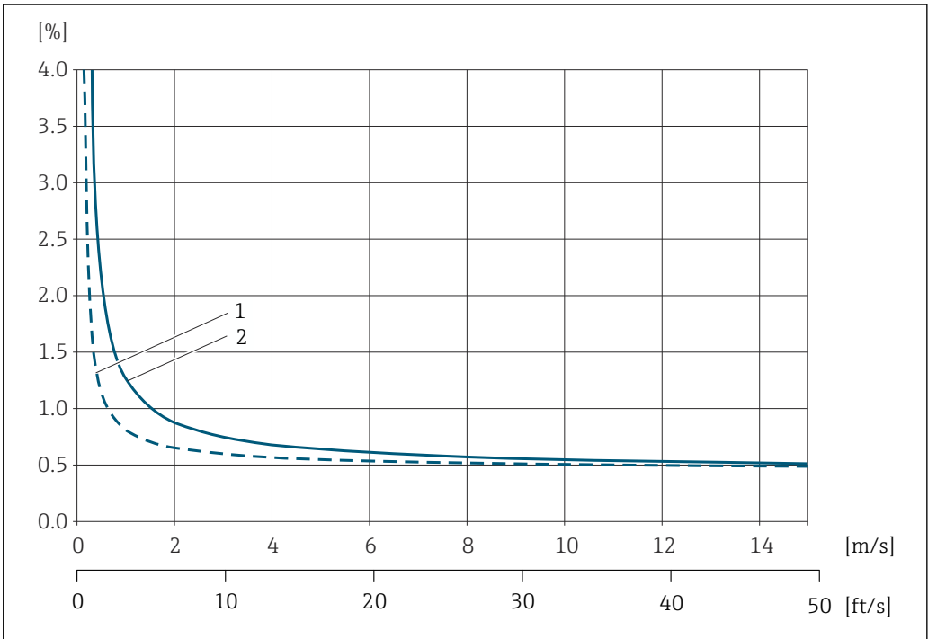
56 Exemplo de erro de medição máximo (vazão volumétrica) em % da leitura.
