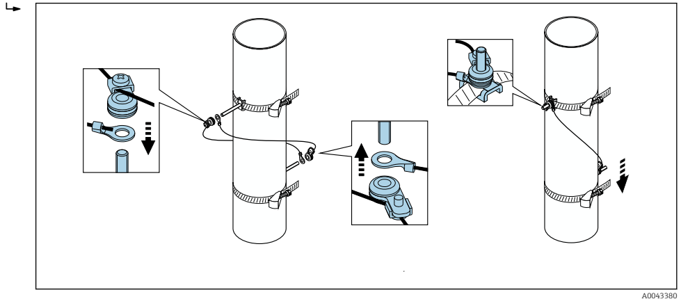
27 Posicionamento das cintas de bandagem (etapas 2 a 4)
