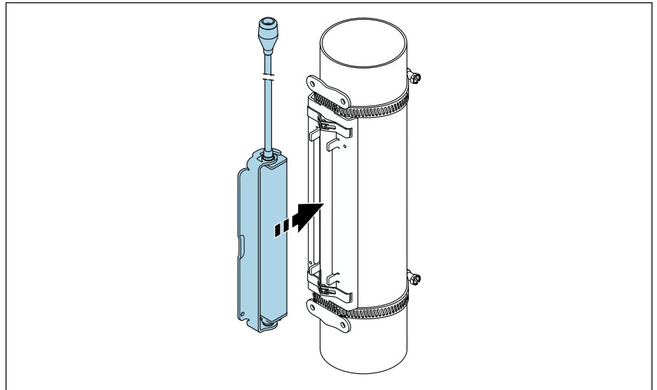
24 Posicionamento do invólucro do sensor
