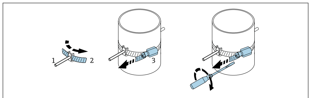
20 Porta-sensor com cintas de bandagem (diâmetros nominais médios), sem parafuso articulado
