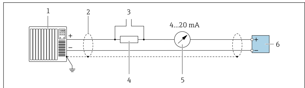
39 Exemplo de conexão para saída de corrente de 4 a 20 mA HART (ativa)
