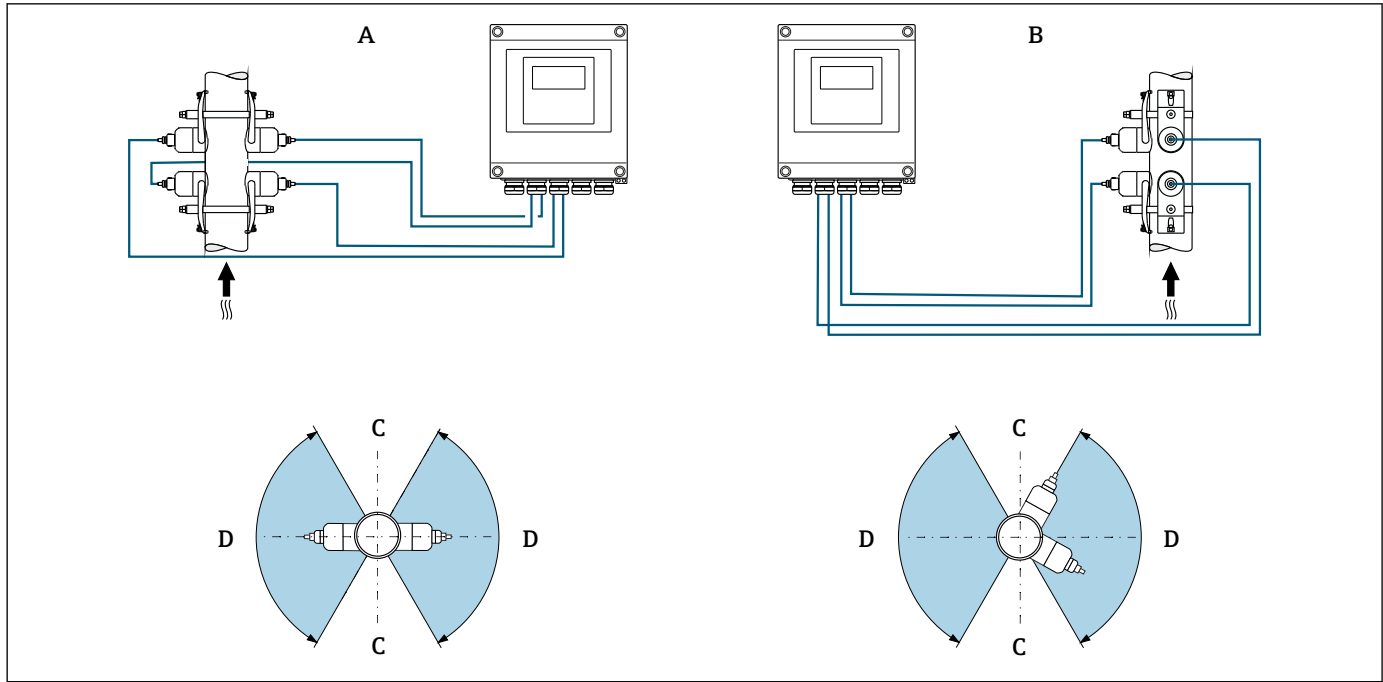
6 Medição de dois caminhos: exemplos para a disposição horizontal dos conjuntos de sensores em um ponto de medição
