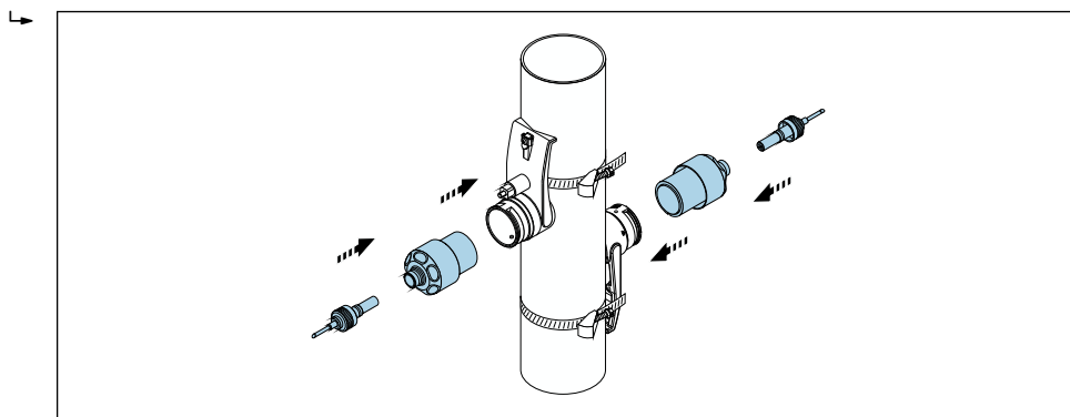
31 Instalação dos sensores e conexão do cabo do sensor
