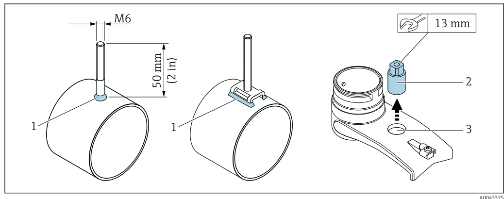
22 Suporte com parafusos soldados
