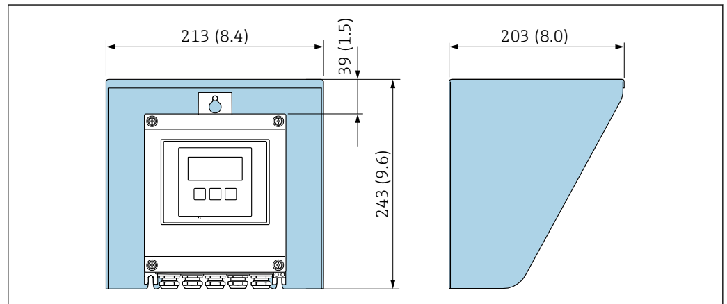
15 Tampa de proteção contra tempo; unidade de engenharia mm (pol.)
