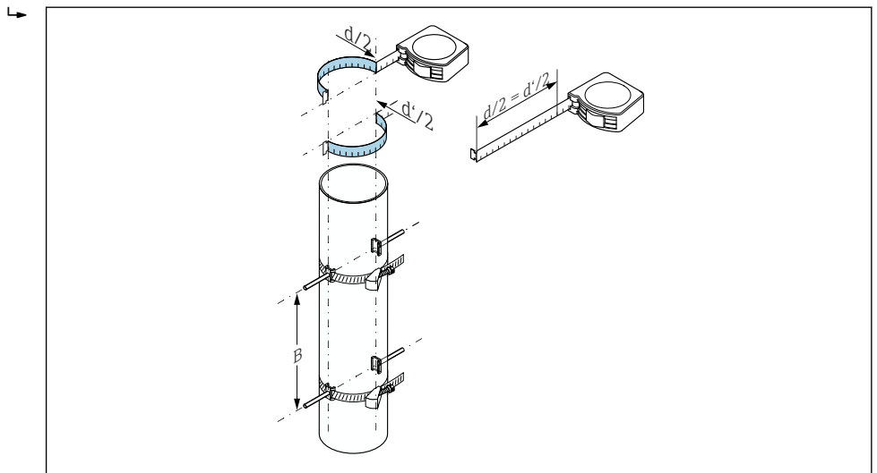
28 Posicionamento das cintas e dos parafusos de fixação com uma fita métrica (etapas 2 a 4)
