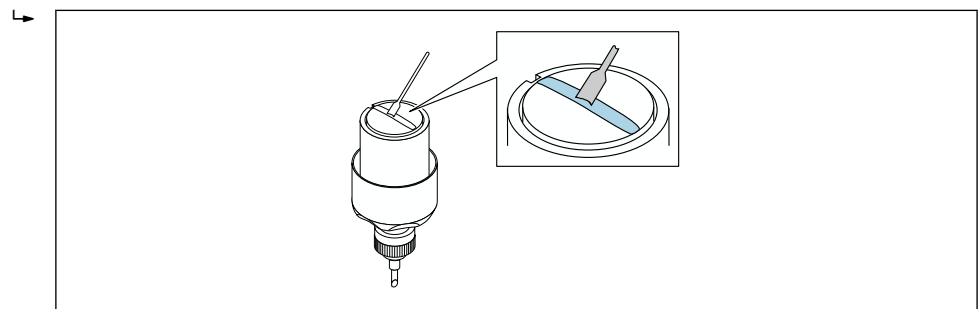
30 Cubra as superfícies de contato do sensor com gel de acoplamento (se não houver coxim de acoplamento)
