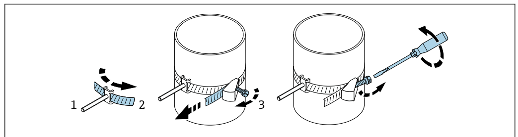
19 Porta-sensor com cintas de bandagem (diâmetros nominais médios), com parafuso articulado
