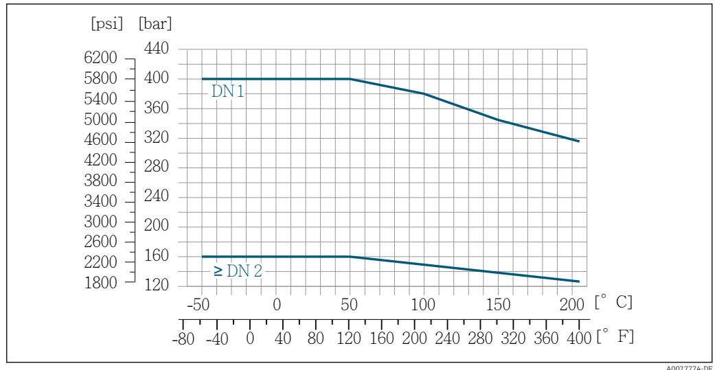
25 4-VCO-4 Kupplung: 1.4539 (904L); 8-VCO-4 Kupplung: 1.4539 (904L); NPTF Gewindeadapter: 1.4539 (904L)
