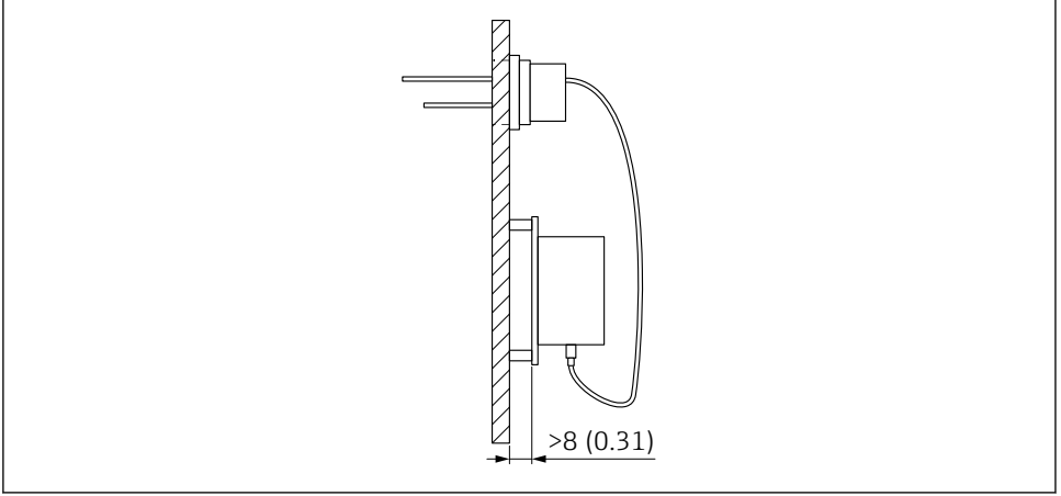
5 Yüksek yüzey sıcaklığına sahip konteyner duvarına montaj. Ölçü birimi mm (in)
