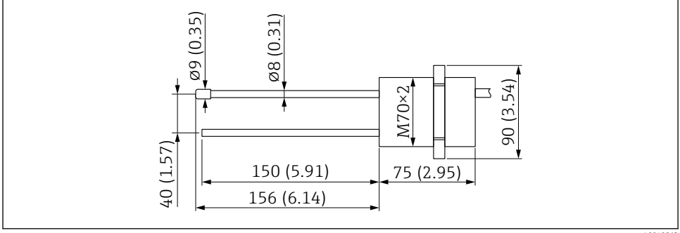
6 İki çubuklu sensör boyutları, yuvarlak tasarım. Ölçü birimi mm (in)
