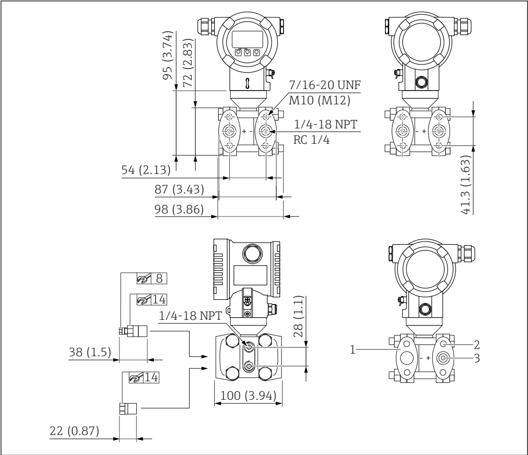
9 Вид спереди, вид слева-сбоку, вид справа-сбоку. Гайки всегда расположены на стороне низкого давления. Единица измерения мм (дюйм)
