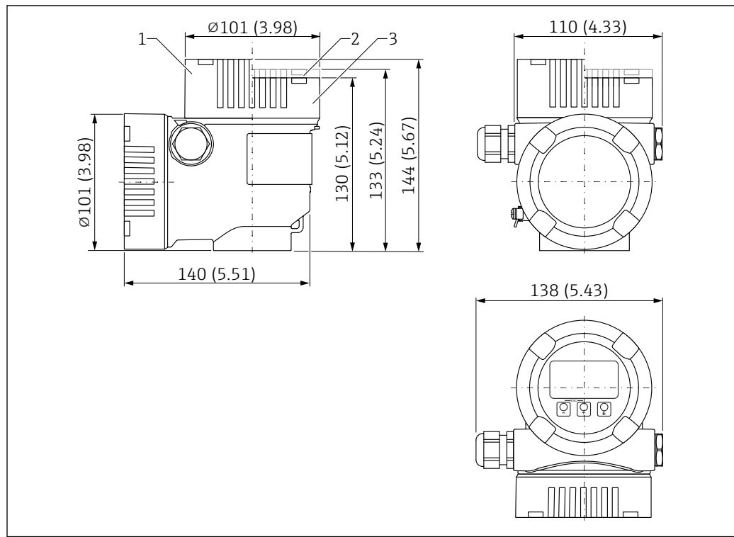
図 22 寸法 ; デュアルコンパートメントハウジング L 字型 (アルミニウム、コーティング) ; M20 カップリングおよびプラグ (プラスチック) 付き。測定単位 mm (in)
