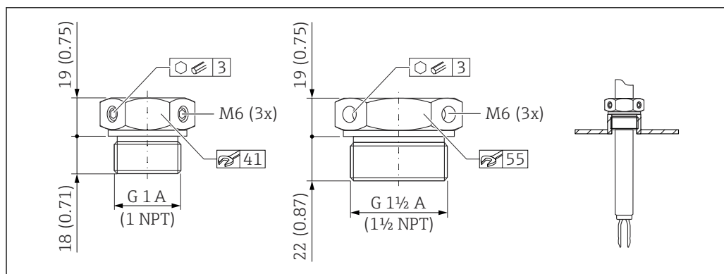
図 40 スライディングスリーブ (大気圧用 : p_e = 0 \text{ MPa} (0 psi))。測定単位 mm (in)
