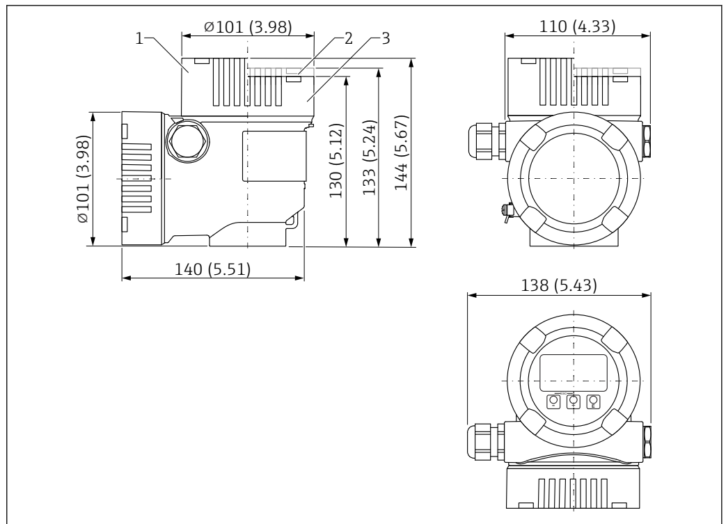
図 23 寸法；デュアルコンパートメントハウジングL字型（SUS 316 L 相当）；M20 カップリングおよびプラグ（プラスチック）付き。測定単位 mm (in)
