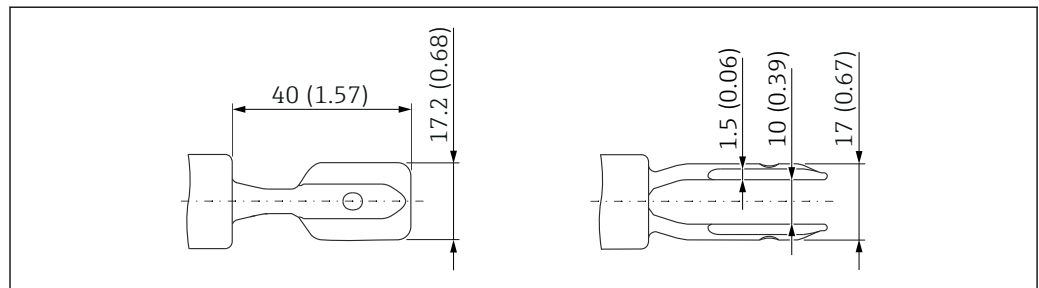
図 27 音叉部。測定単位 mm (in)
