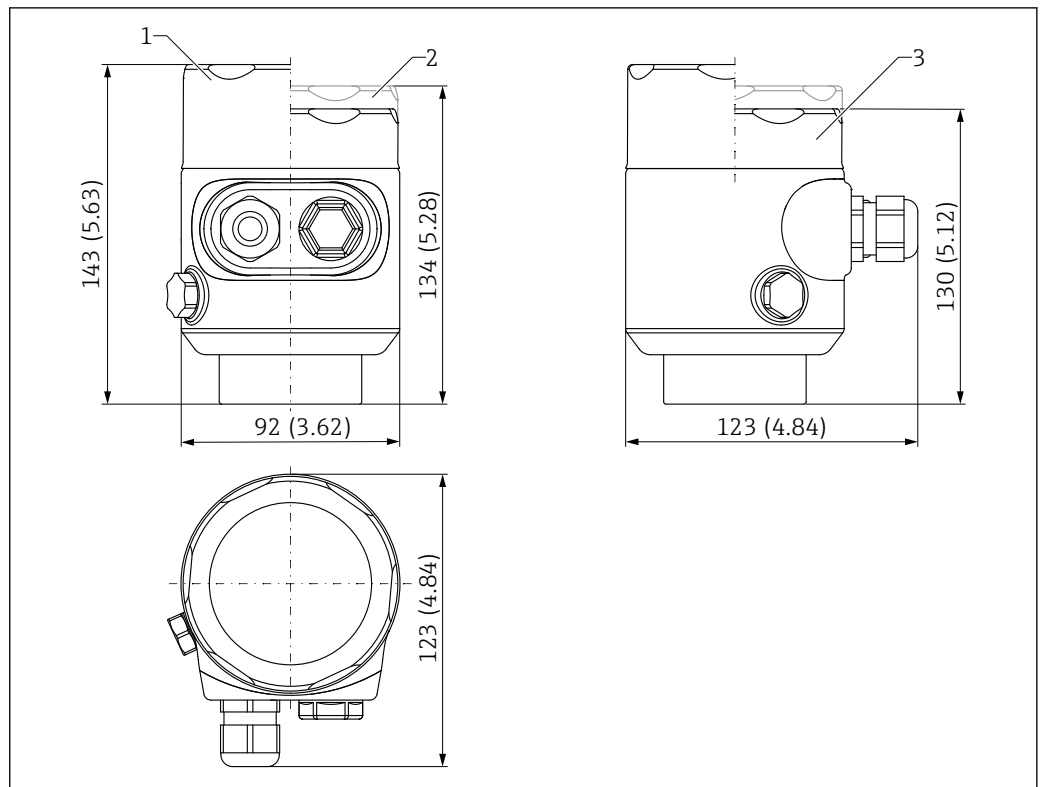
図 21 シングルコンパートメントハウジング、SUS 316L 相当、サニタリ仕様の寸法。測定単位 mm (in)
