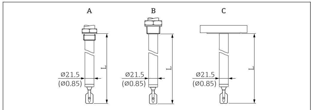
図 26 伸長パイプ（センサ長 L）。測定単位 mm (in)
