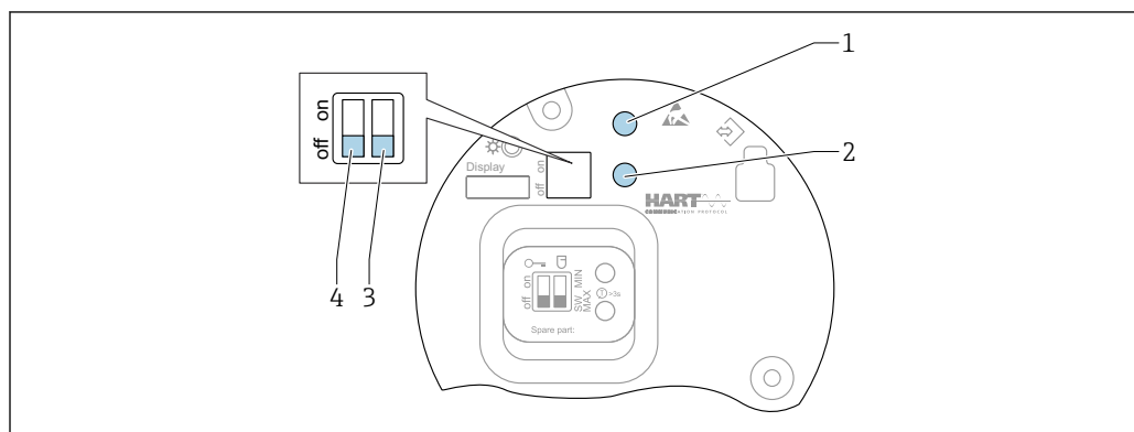
図 36 FEL60H エレクトロニックインサートの操作キーおよび DIP スイッチ
