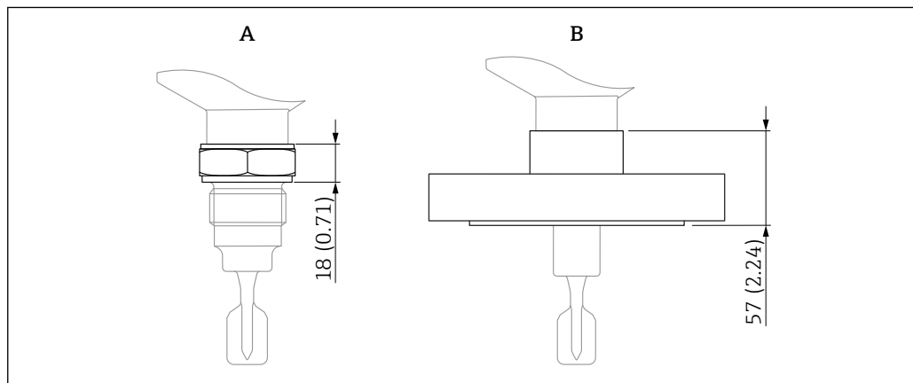
図 28 プロセス接続の最大高さ仕様
