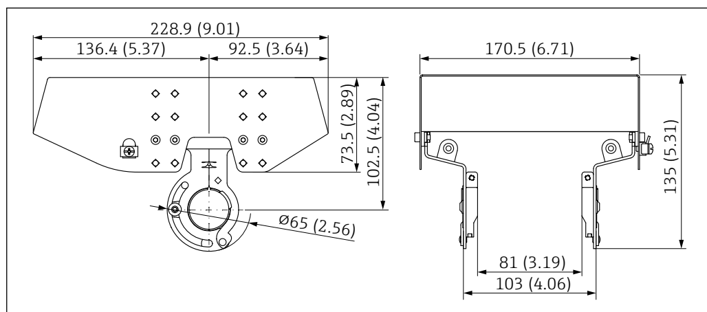
図 38 アルミニウム製デュアルコンパートメントハウジング用保護カバー。測定単位 mm (in)
