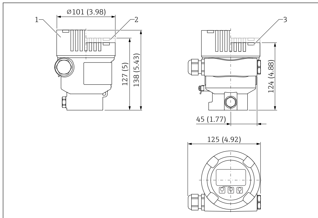
図 20 シングルコンパートメントハウジング、アルミニウム、コーティングの寸法。測定単位 mm (in)
