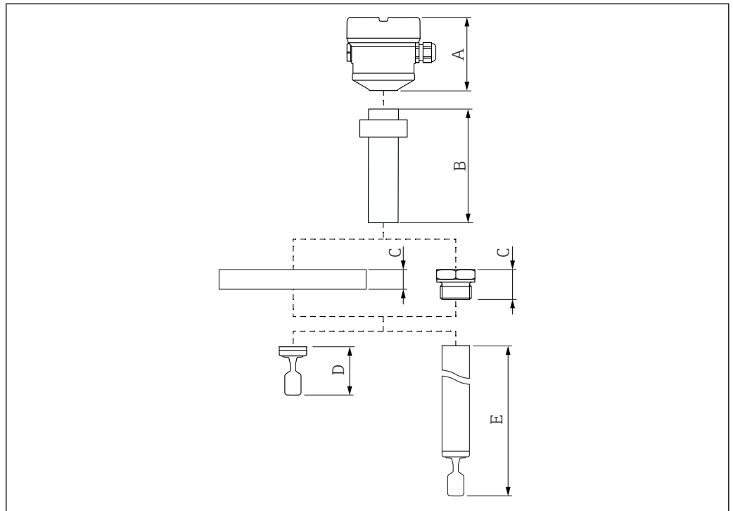
図 18 本体高さを計算するための構成品
