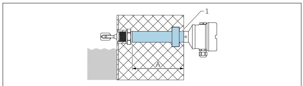
図 24 ガラスガスタイトフィードスルー付き温度セパレータ
