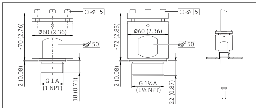
図 41 高圧用スライディングスリーブ。測定単位 mm (in)
