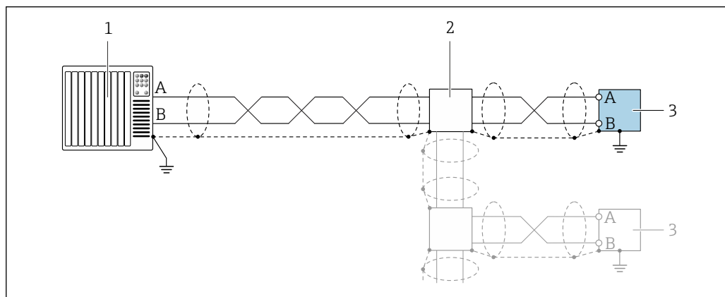
18 Пример подключения для Modbus RS485
