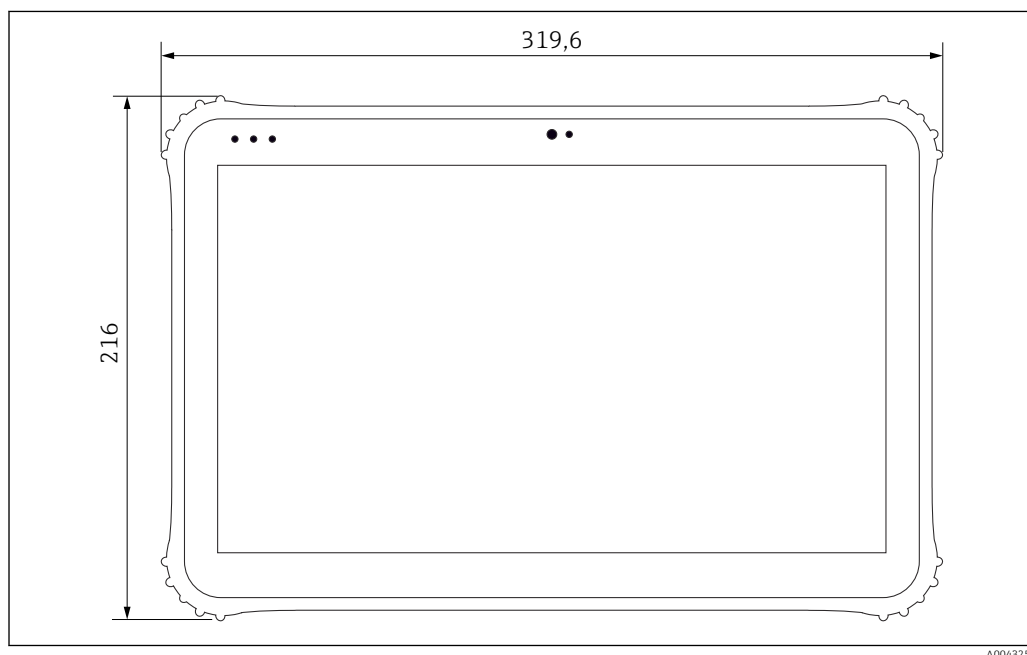
10 Vorderansicht
