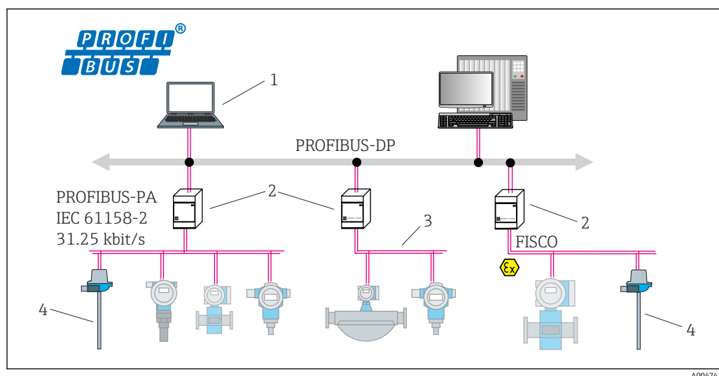
図 2 PROFIBUS® PA 通信の機器構成
