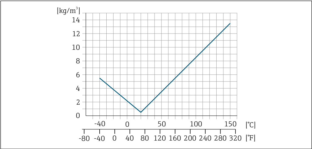
45 Ajustage sur site de la masse volumique, par exemple à +20 °C (+68 °F)
