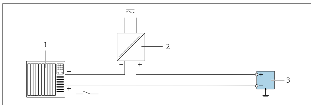
25 Exemple de raccordement pour l'entrée état
