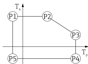
44 Корпус 316L, гигиенический; рабочая температура -40 до +80 °C ( -40 до +176 °F)
