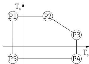
46 Корпус 316L, гигиенический; рабочая температура -40 до +200 °C ( -40 до +392 °F)
