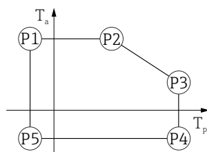
42 Корпус 316L; рабочая температура -40 до +280 °C ( -40 до +536 °F)
