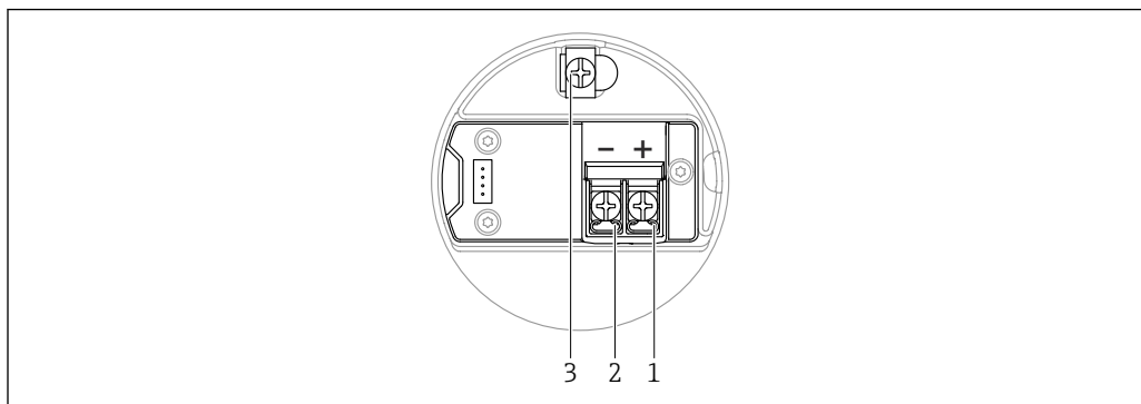
9 Соединительные клеммы и клемма заземления в клеммном отсеке
