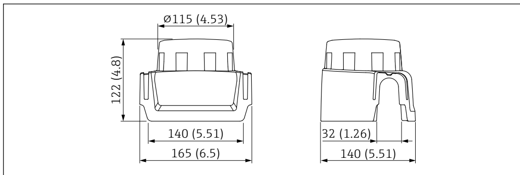
23 Размеры защитного козырька от погодных явлений, пластмасса, XW111. Единица измерения мм (дюйм)
