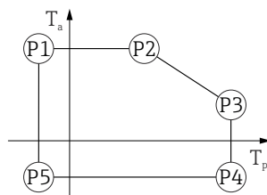
34 Алюминиевый корпус с покрытием; рабочая температура -40 до +80 °C ( -40 до +176 °F)
