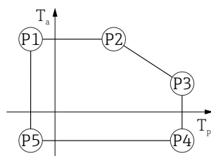
41 Корпус 316L; рабочая температура -40 до +200 °C ( -40 до +392 °F)
