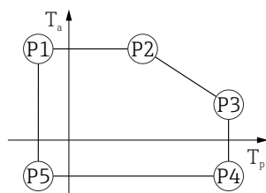
45 Корпус 316L, гигиенический; диапазон рабочей температуры: -40 до +150 °C ( -40 до +302 °F)
