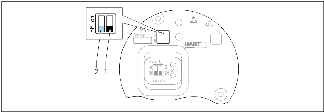
图 27 FEL60H 电子插件上的 DIP 开关的功能
