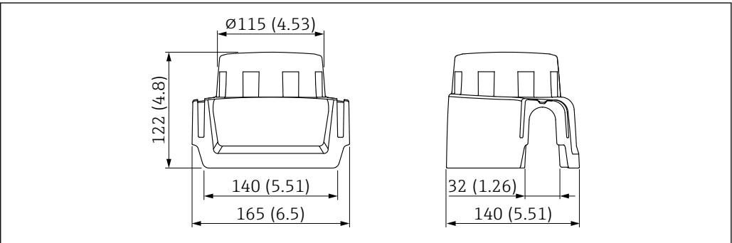
30 防护罩，适用单腔体铝外壳。测量单位 mm (in)
