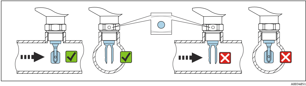
12 安装在管道中（注意叉体安装位置和标记）
