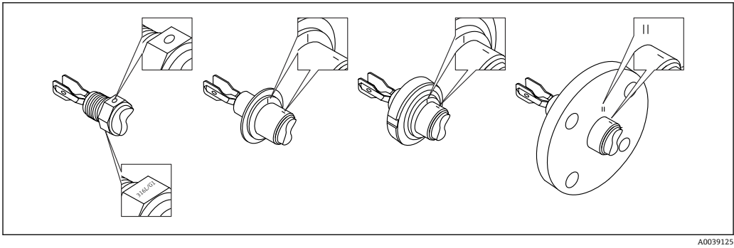
11 参照标记水平安装在罐体中时的叉体位置
