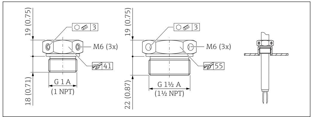
图 32 常压滑动套管 p_e = 0 \text{ bar (0 psi)} 。测量单位 mm (in)
