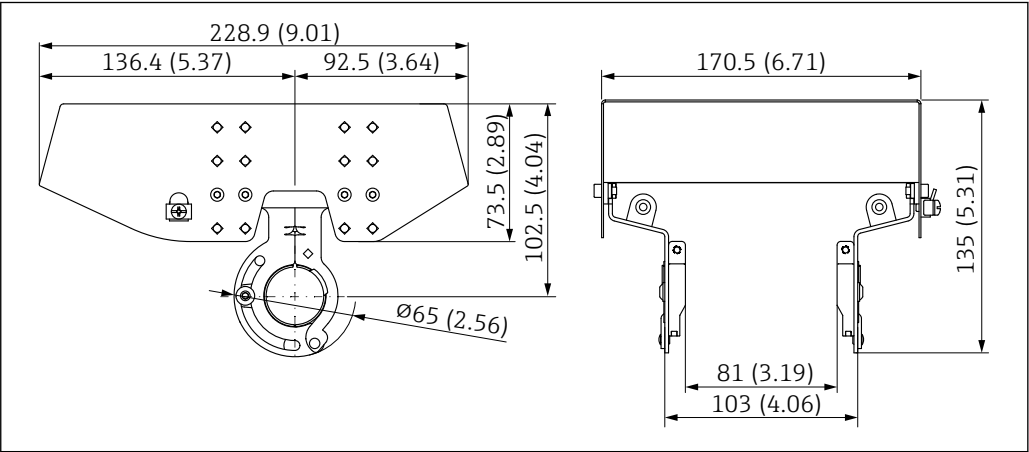
29 防护罩，适用双腔体外壳。测量单位 mm (in)
