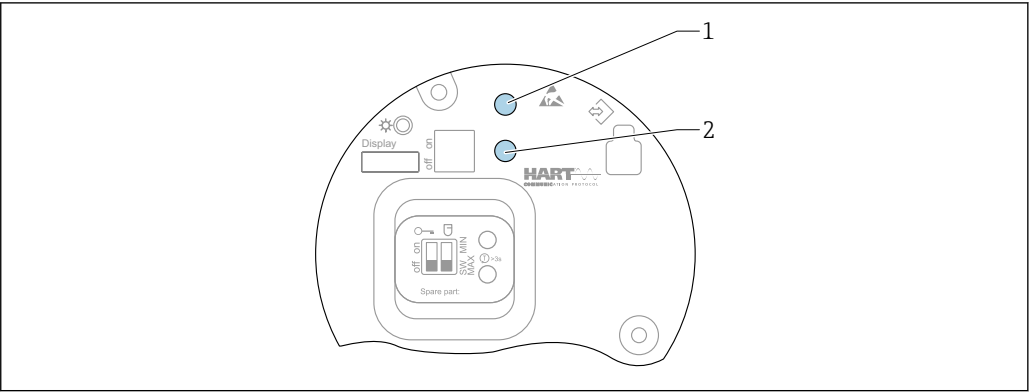
图 28 FEL60H 电子插件上的操作按键 1+2 同时按下：复位设备的操作按键（恢复出厂状态）
