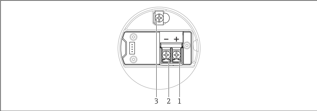
图 19 接线腔中的接线端子和接地端
