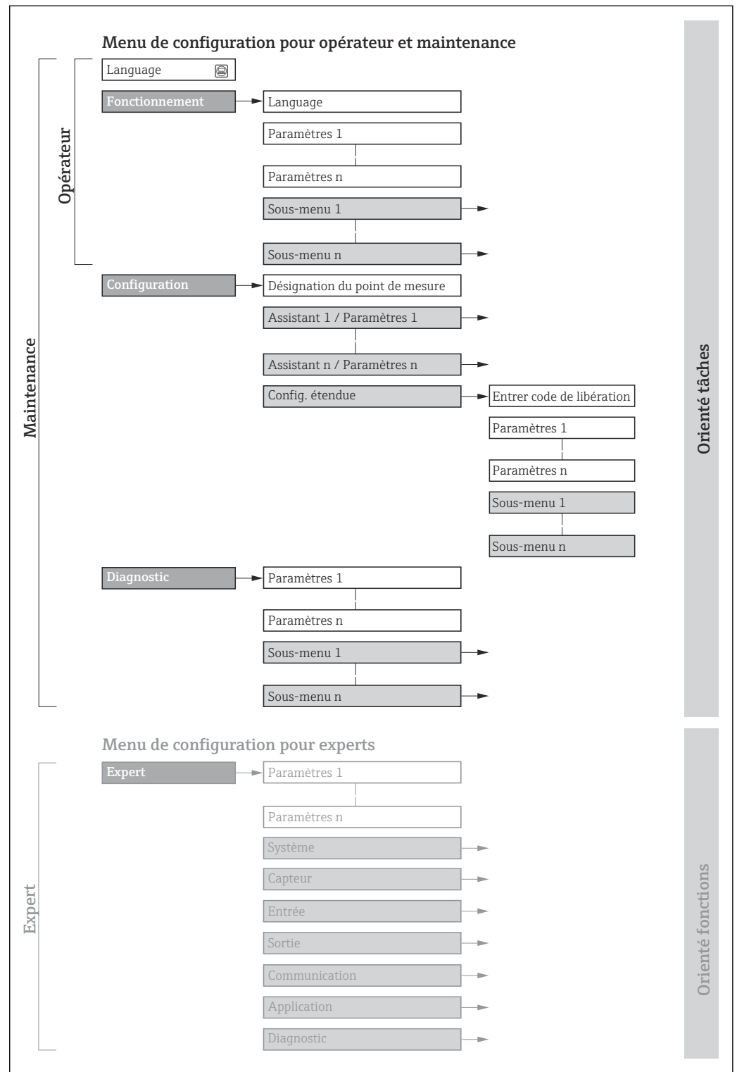
23 Structure schématique du menu de configuration
