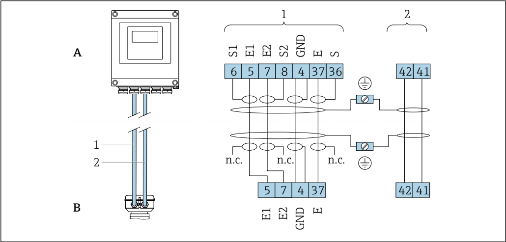
12 Asignación de terminales en la versión separada
