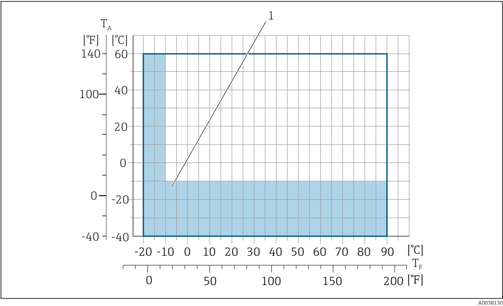
T_A Rango de temperaturas ambiente T_F Temperatura fluido 1 Área coloreada: el rango de temperaturas ambiente de -10 ... -40 °C (+14 ... -40 °F) y el rango de temperaturas del fluido de -10 ... -20 °C (+14 ... -4 °F) solo son válidos para las bridas de acero inoxidable
