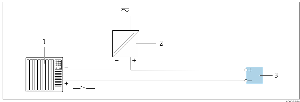
24 Ejemplo de conexión de entrada de estado
