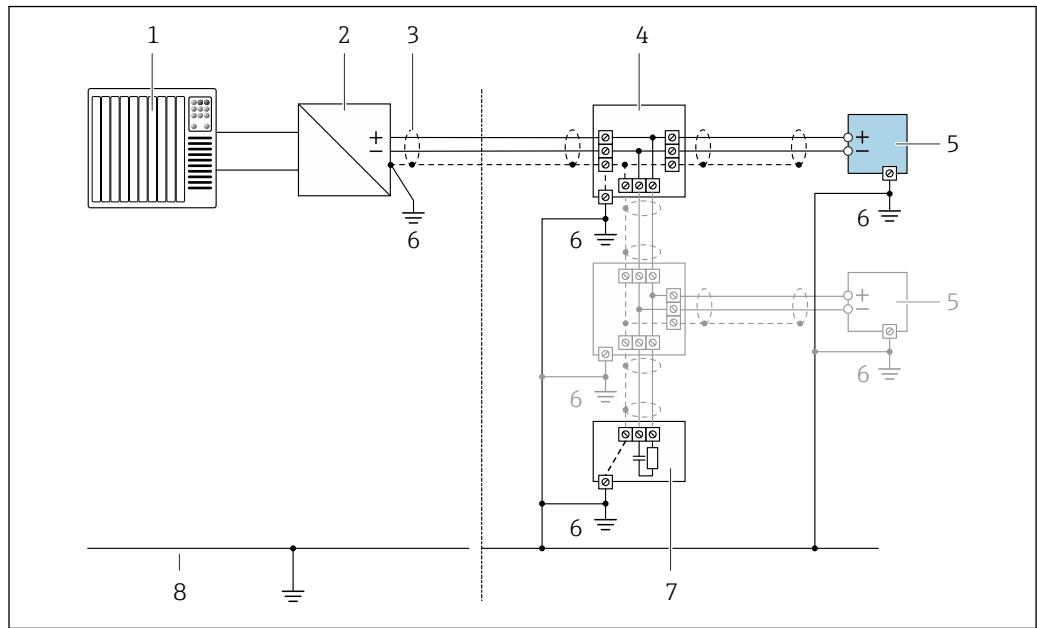
26 Пример подключения для интерфейса FOUNDATION Fieldbus
