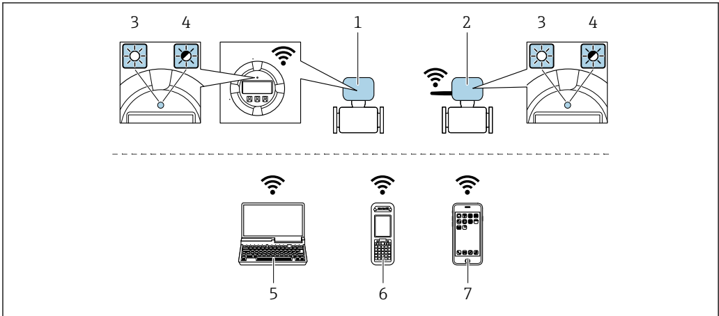
1 Преобразователь со встроенной антенной WLAN 2 Преобразователь с внешней антенной WLAN 3 Светодиод горит постоянно: на измерительном приборе активировано соединение с WLAN 4 Светодиод мигает: установлено соединение по сети WLAN между устройством управления и измерительным прибором 5 Компьютер с интерфейсом WLAN и веб-браузером для доступа к веб-серверу встроенного устройства или с операционной системой (например, FieldCare, DeviceCare) 6 Мобильный портативный терминал с интерфейсом WLAN и веб-браузером для доступа к веб-серверу или операционной системе встроенного устройства (например, FieldCare, DeviceCare) 7 Смартфон или планшет (например, Field Xpert SMT70)
