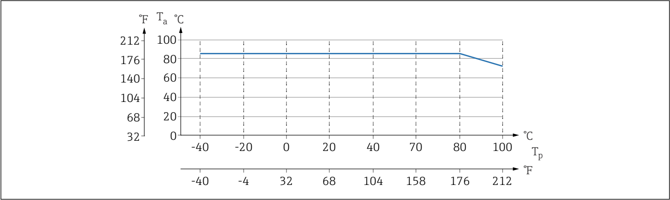
图 12 以上为无保温层垂直安装时的温度范围。
