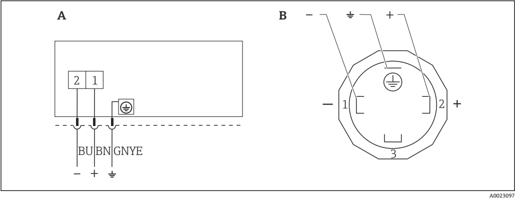
图 6 BN = 棕色, BU = 蓝色, GNYE = 绿/黄相间
