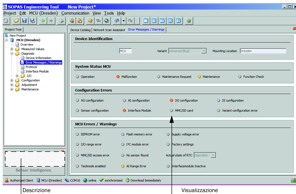
Figura 89 Direttorio "Diagnosis / Errors/Warnings"
