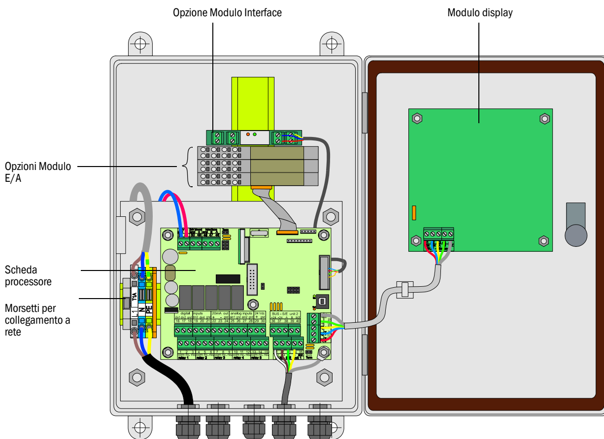
Figura 24 MCU nella custodia a parete
