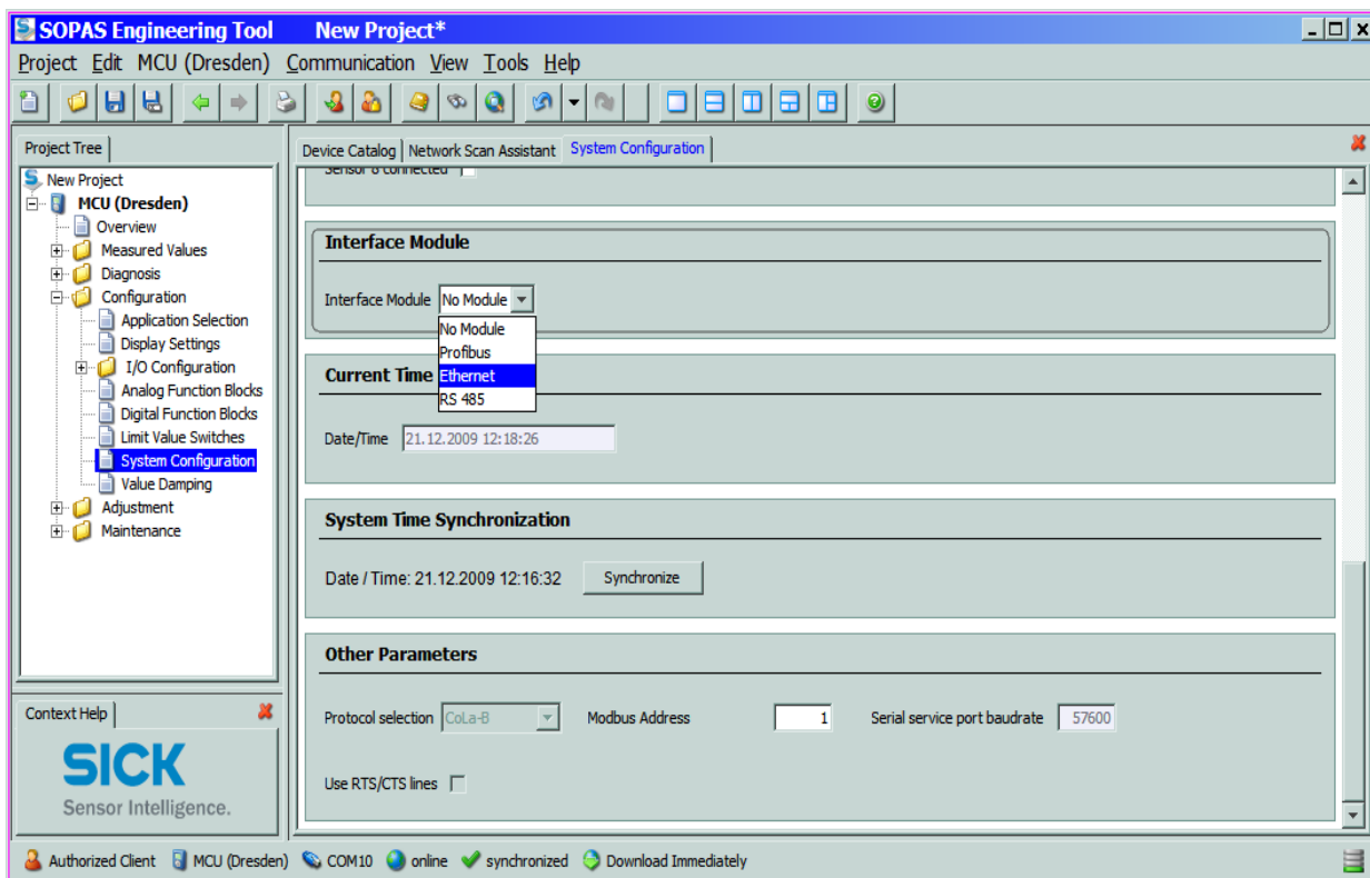
Figura 74 Direttorio "Configuration / System Configuration"
