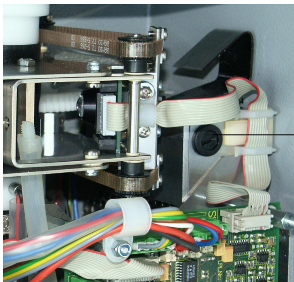
Figura 88 Portafusibili in caso di opzione blocco di alimentazione
