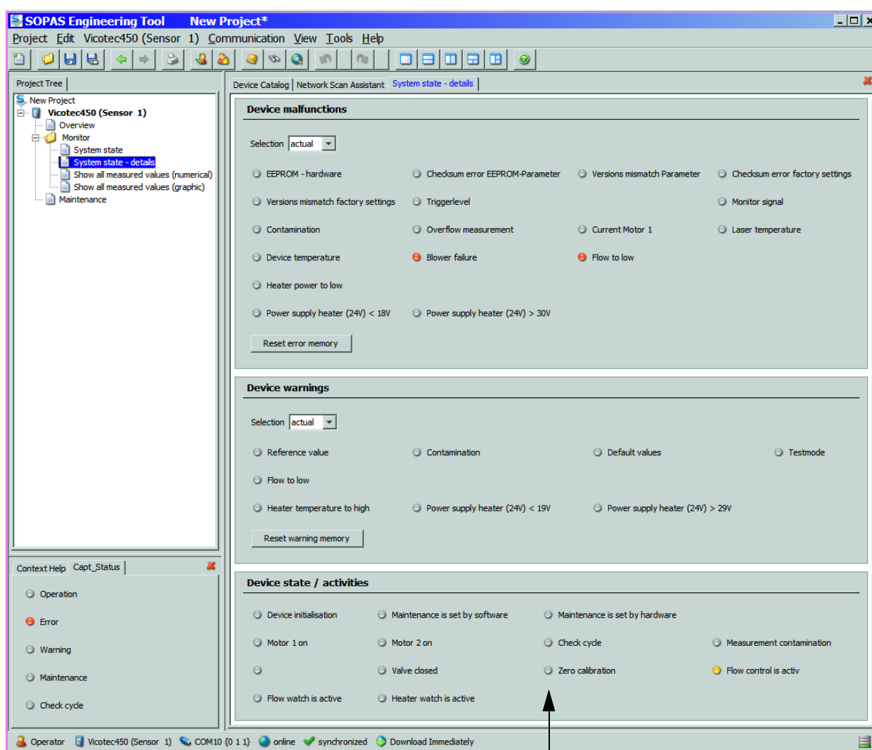
Figura 87 Direttorio "Monitor / System state - details"
