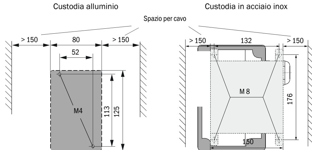
Figura 22 Ingombri di montaggio del modulo d'interfaccia
