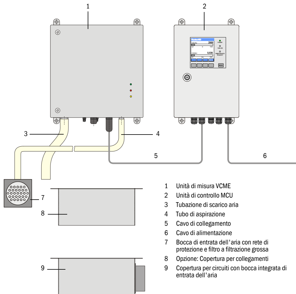
Figura 6 Componenti VICOTEC450
