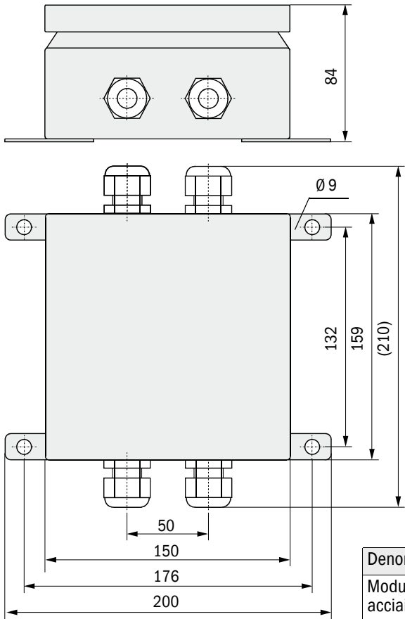
Figura 102 Modulo d'interfaccia in custodia in acciaio inox
