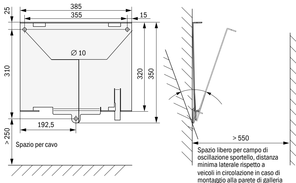
Montaggio dell'opzione piastra di montaggio
