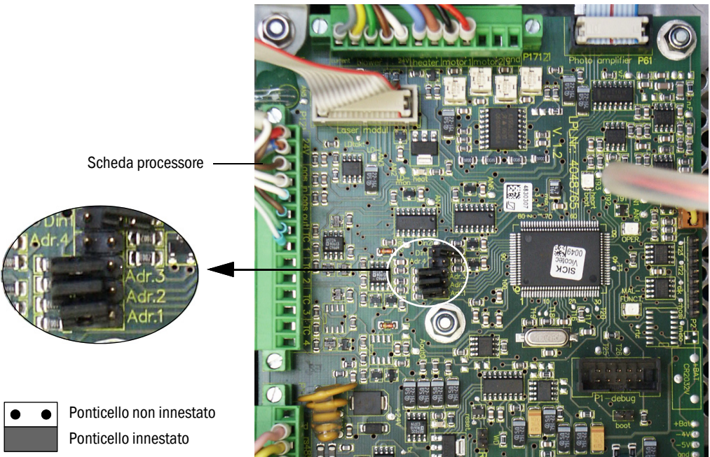
Figura 40 Indirizzamento dell'unità di misura tramite hardware
