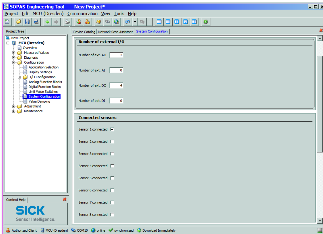
Figura 70 Direttorio "Configuration / System Configuration" (esempio per impostazioni)
