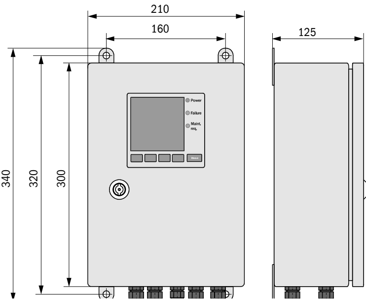
Figura 99 Unità di controllo MCU in custodia a parete (visualizzazione con opzione Modulo Display)
