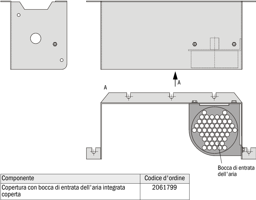
Figura 96 Copertura con bocca di entrata dell'aria integrata da sotto
