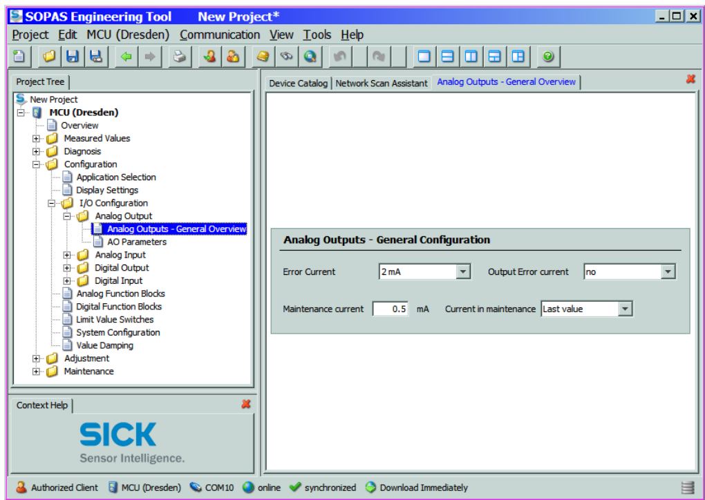
Figura 62 Sottodirettorio "Overview analog output" (esempio per impostazioni)
