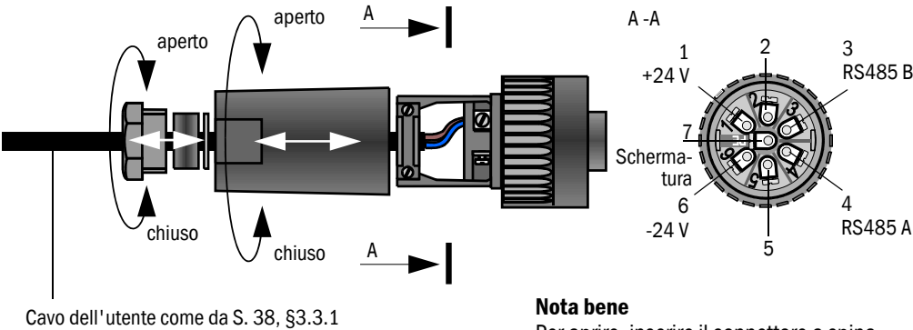
Figura 26 Collegamento connettore a spina con il cavo installato sul luogo
