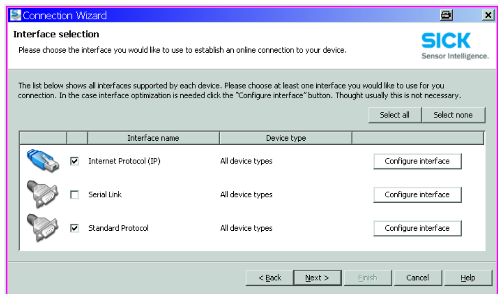
Figura 51 Selezione dell'interfaccia
