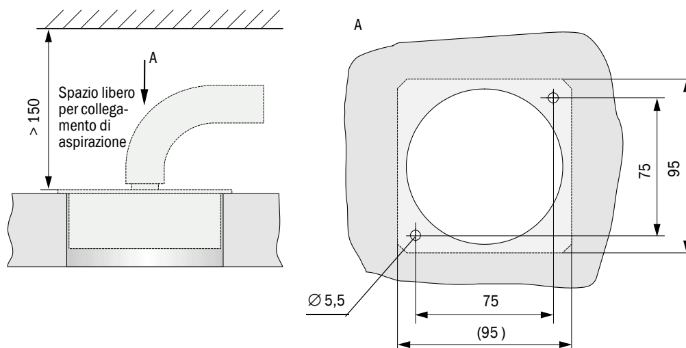
Figura 20 Ingombri di montaggio per bocca di entrata dell'aria con rete di protezione per installazione in soffitto intermedio
