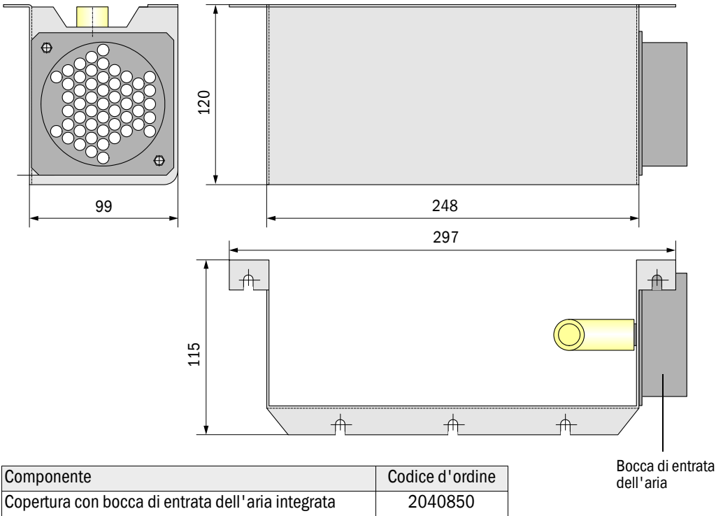
Figura 96 Copertura con bocca di entrata dell'aria integrata da sotto
