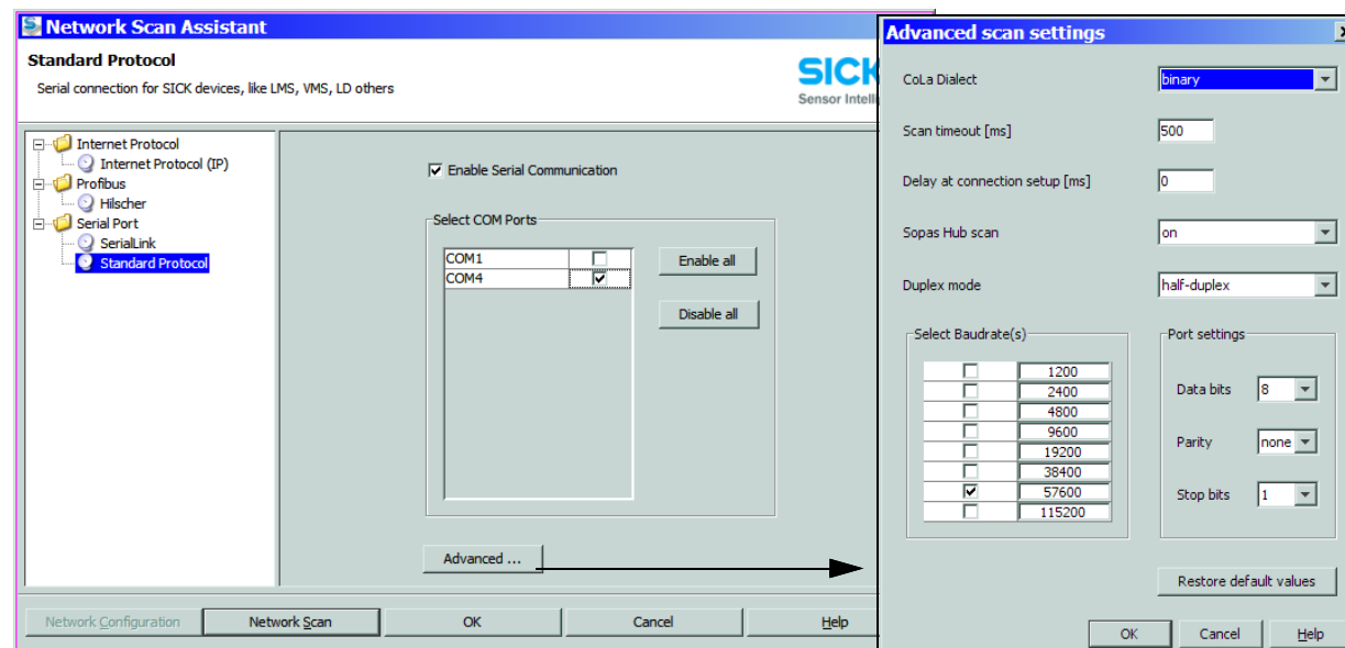
Figura 46 Selezione e configurazione della COM Port
