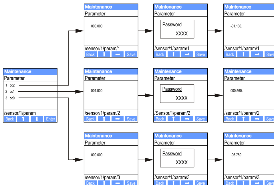
Figura 82 Impostazione dei coefficienti di regressione
