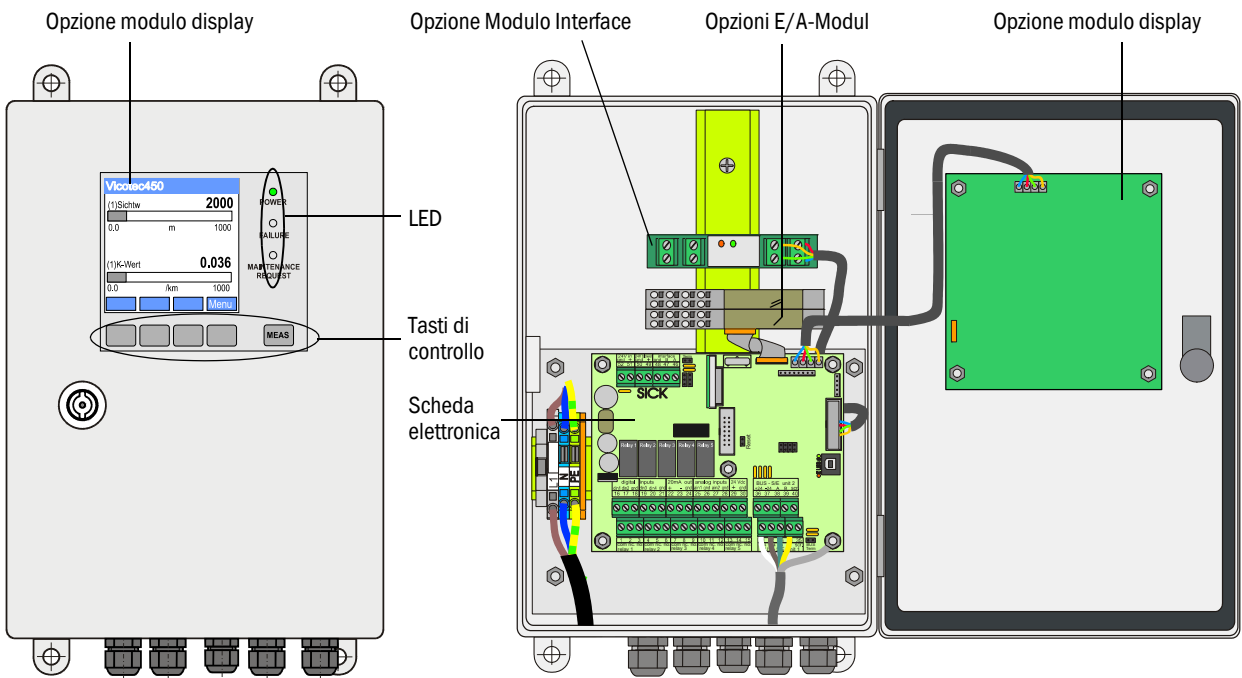
Figura 10 Unità di controllo MCU nella custodia a parete con opzioni
