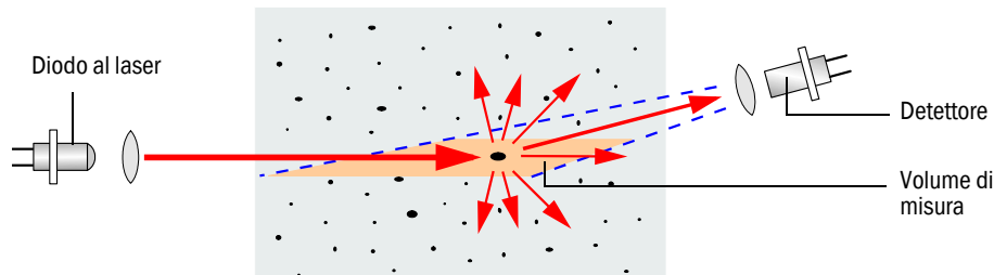
Figura 3 Principio di misurazione dispersione della luce
