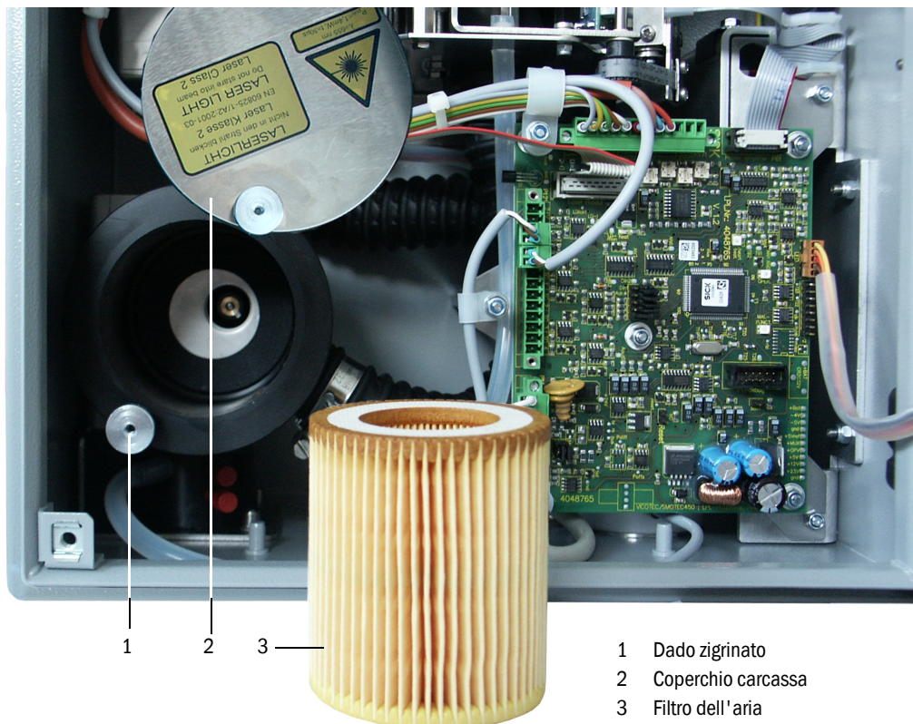
Sostituzione del filtro dell'aria
