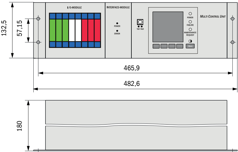
Figura 100 Unità di controllo MCU in unità a innesto 19" (visualizzazione con opzione Modulo Display)
