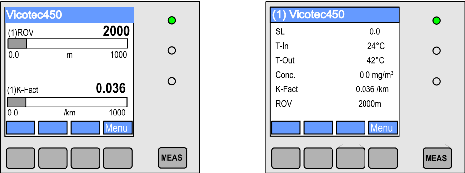
Figura 12 Display LC con visualizzazione grafico (a sinistra) e indicazione di testo (a destra) (esempio)
