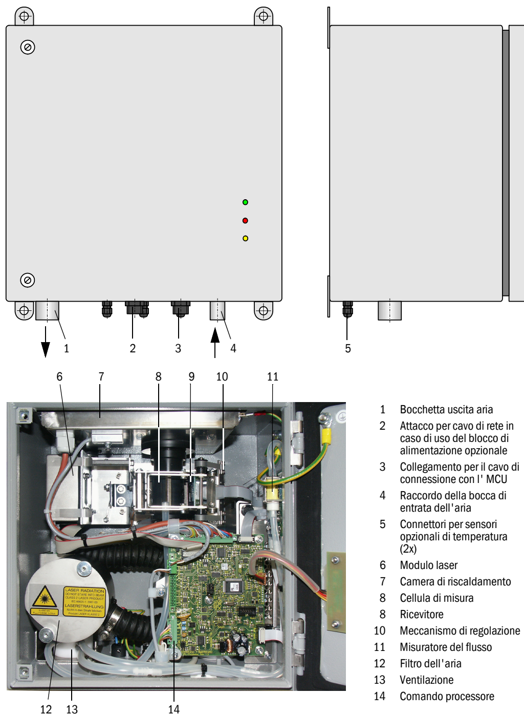
Unità di misura VCME
