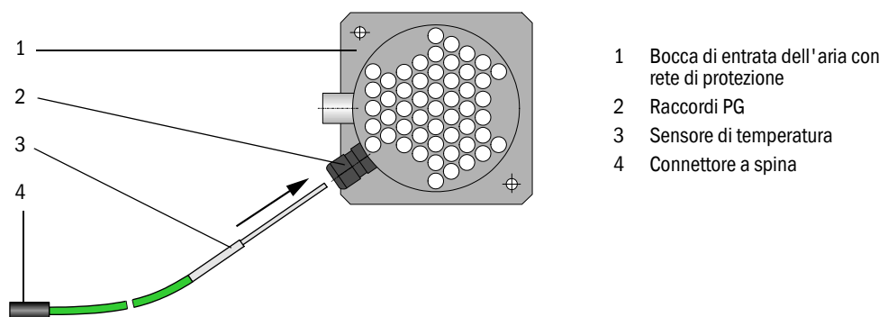
Figura 23 Installare il sensore di temperatura nella bocca di entrata dell'aria con rete di protezione
