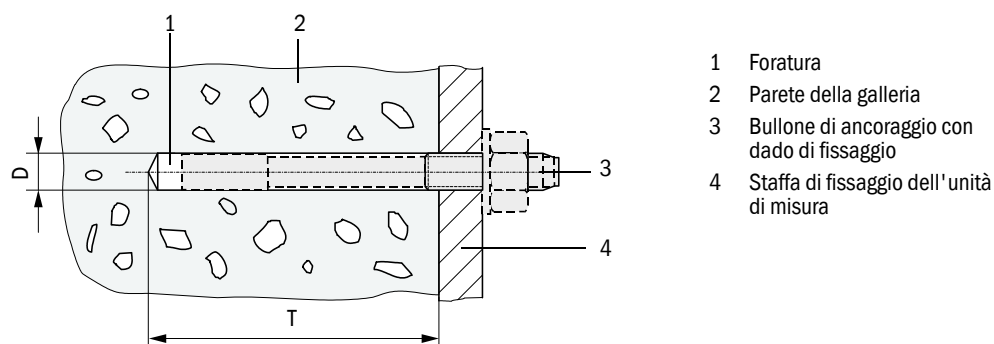
Dimensioni dei fori
