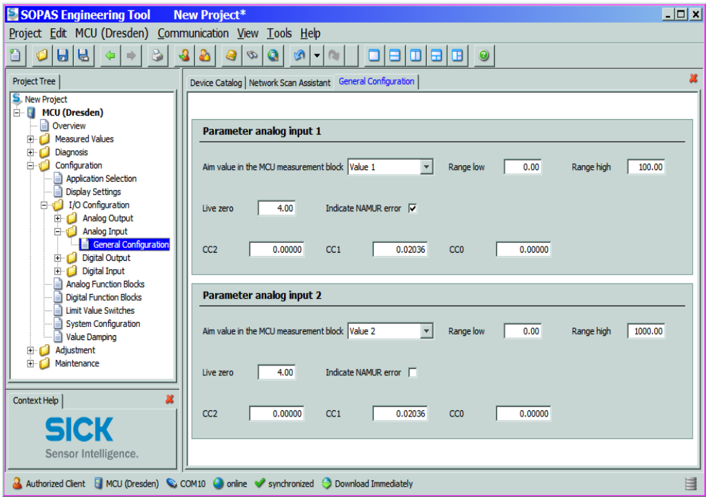
Figura 64 Direttorio "Configuration / I/O Configuration / Analog input"(esempio per impostazioni)
