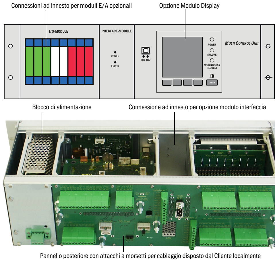
Figura 11 Unità di controllo MCU in custodia 19" con opzioni
