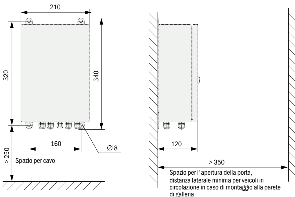
Figura 21 Ingombri di montaggio per MCU nella custodia a parete
