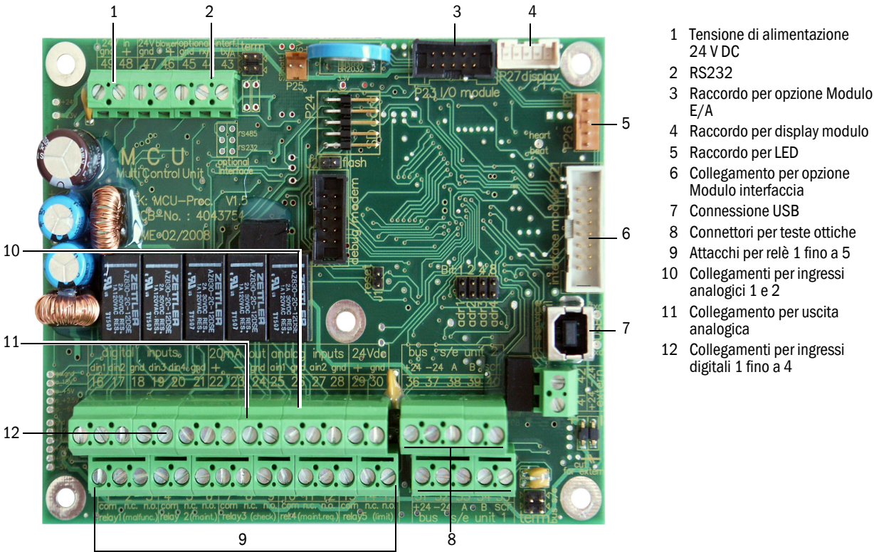
Figura 25 Attacchi della scheda processore
