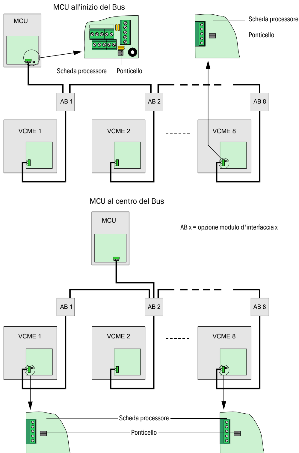
Terminazione Bus
