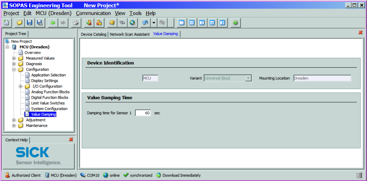
Figura 67 Direttorio "Configuration / Value Damping" (illustrazione per una unità di misura collegata)
