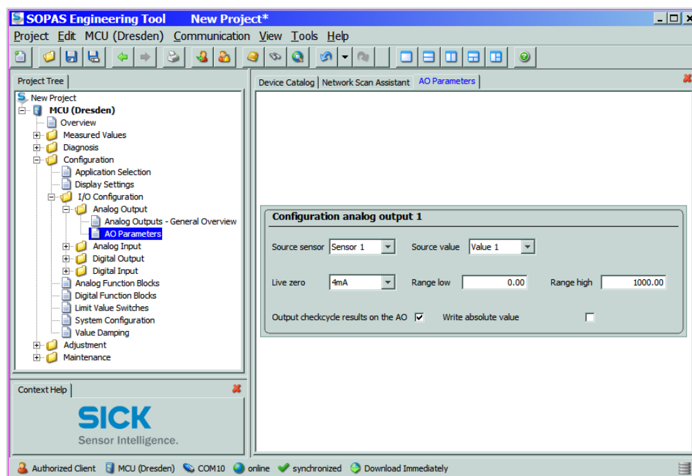
Figura 63 Sottodirettorio "Analog output" (esempio per impostazioni)
