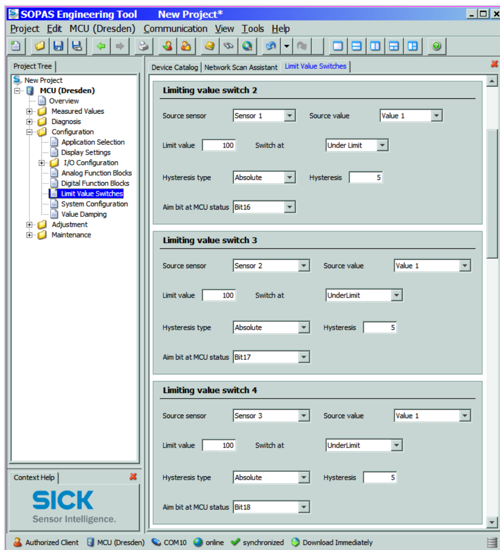
Figura 73 Direttorio "Configuration / Limit Value Switches"
