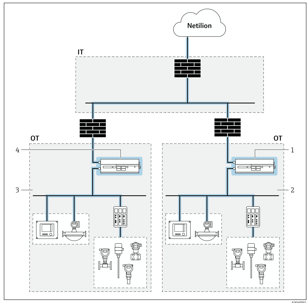
2 Empfohlene Segmentierung bei mehreren Feldbusnetzwerken mit mehreren FieldEdge SGC500 (blaue Markierung zeigt die Systemgrenzen für dieses Handbuch)
