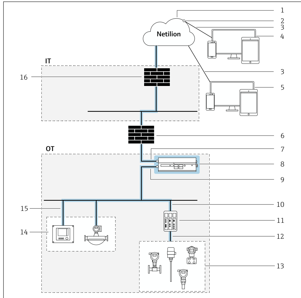
1 Anbindung des FieldEdge SGC500 über getrennte Schnittstellen für Internet und Feldbusnetzwerk (blaue Markierung zeigt die Systemgrenzen für dieses Handbuch)
