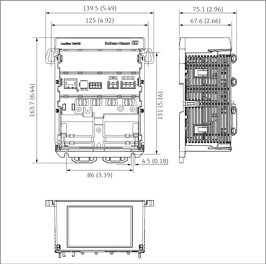
44 设备的外形尺寸示意图；单位：mm (in)
