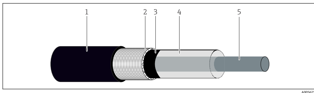
图 12 同轴电缆结构
