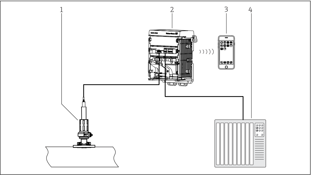
图 2 安装有 Liquiline CM42B（导轨盘装型设备）的测量系统示意图
