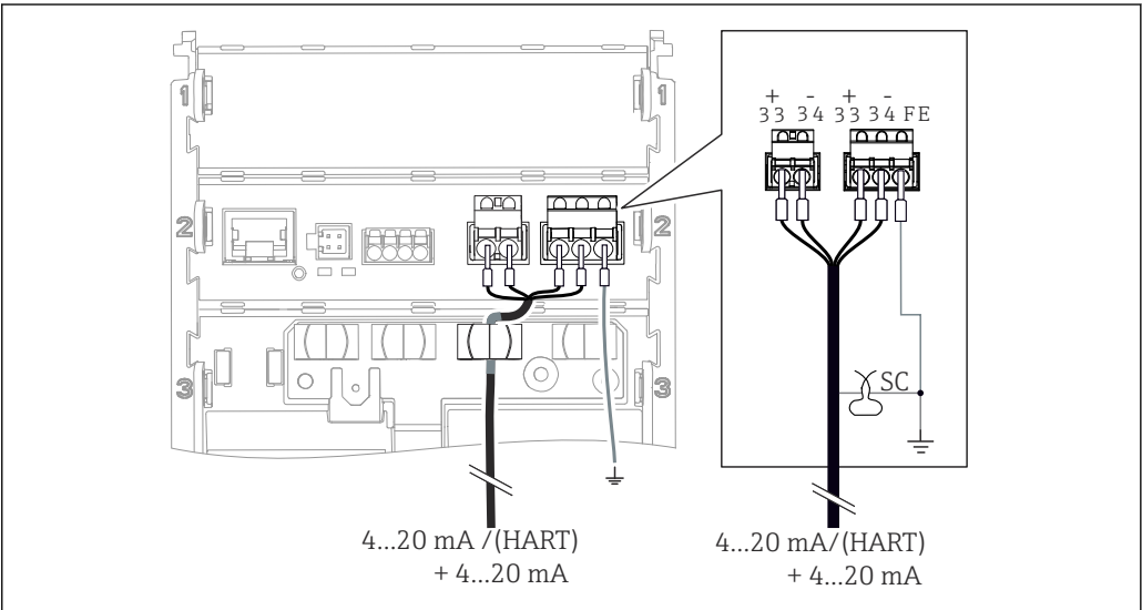
27 通过 1 根屏蔽电缆连接 2 路电流输出（电流输出 1 叠加 HART 信号）
