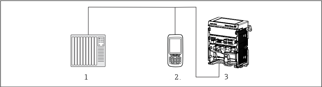
49 接线图：通过 HART 通信进行远程操作（DIN 导轨盘装型设备）
