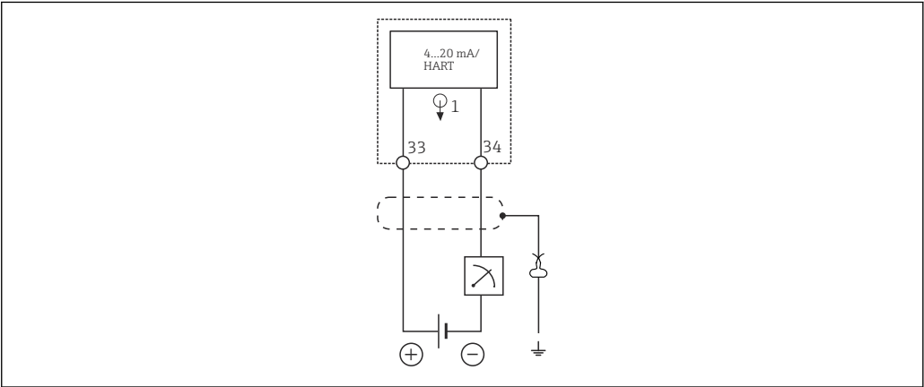
26 接线图：1 路电流输出（电流输出叠加 HART 信号）
