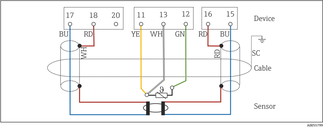
图 9 CLS54 的接线图
