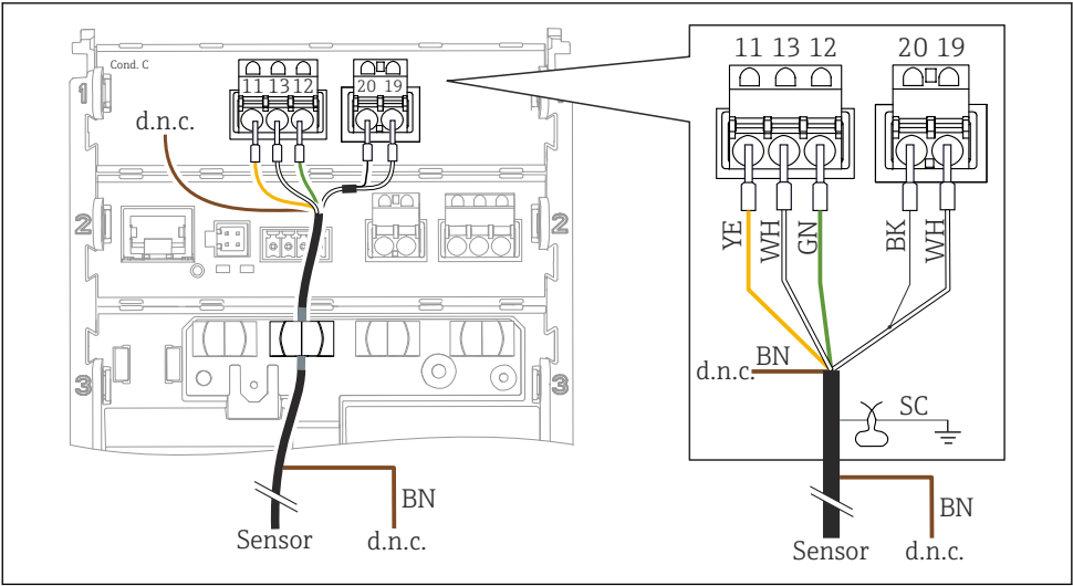
图 10 设备视图
