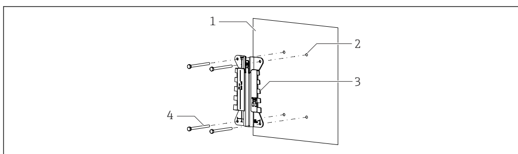
图 32 墙装
