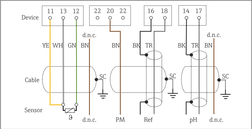
图 22 接线图
