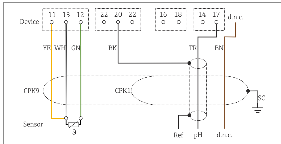
16 接线图
