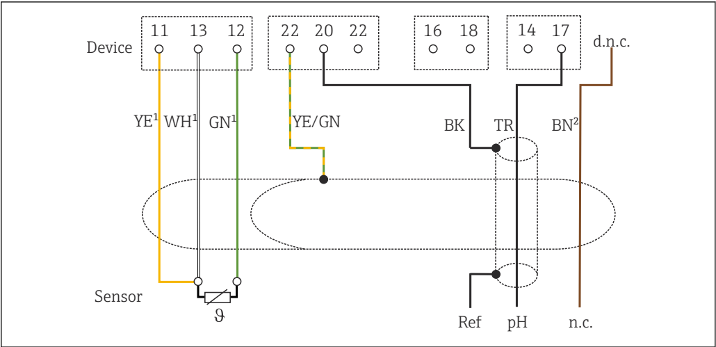
18 接线图
