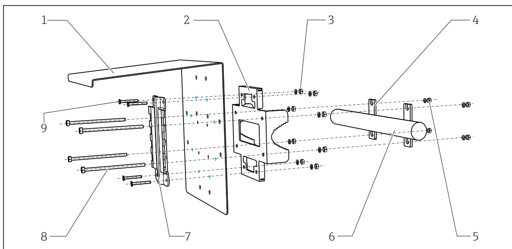
图 36 安装在护栏上
