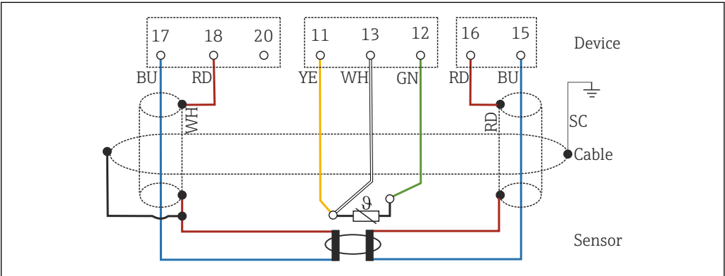
8 CLS50 的接线图
