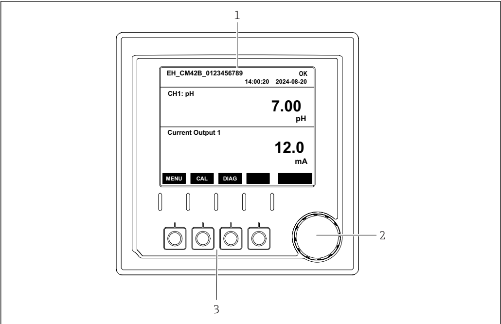
45 操作部件
