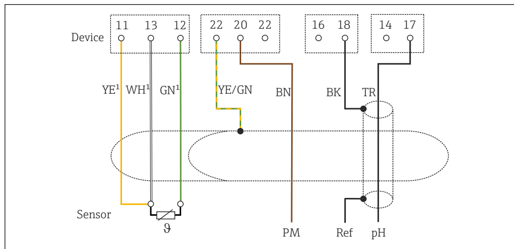
20 接线图
