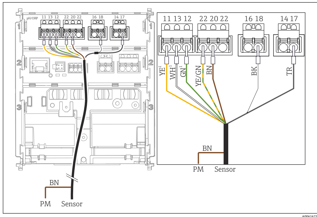
19 设备视图
