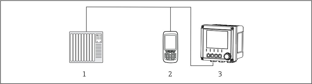
48 接线图：通过 HART 通信进行远程操作（现场型设备）
