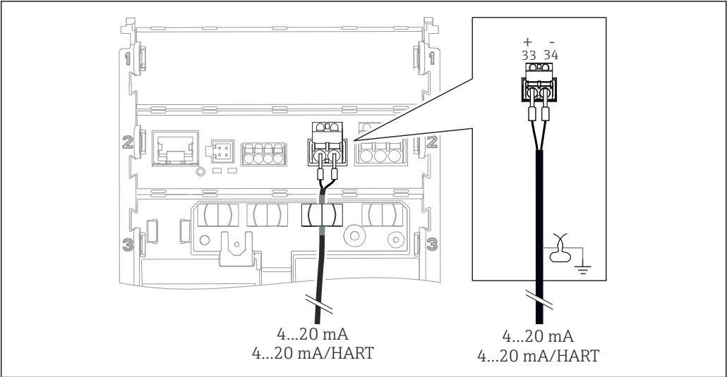
25 连接 1 路电流输出（实例：HART 设备）
