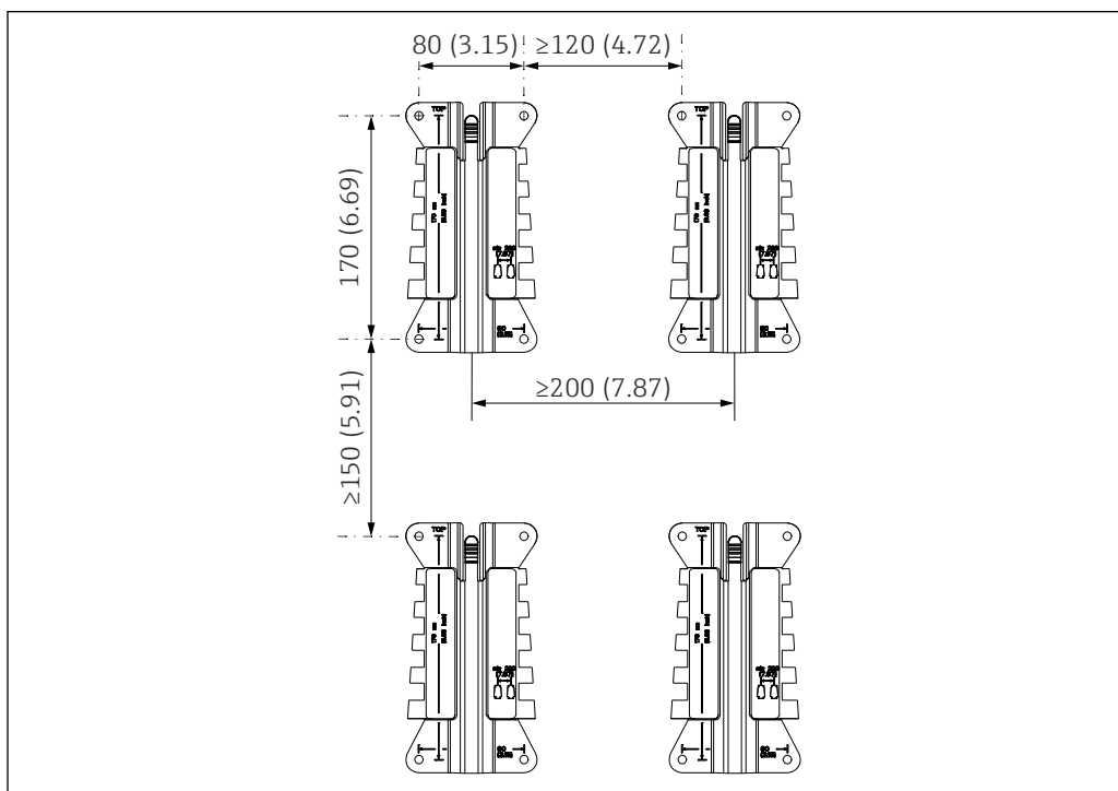
图 31 安装间距尺寸; 单位: mm (in)
