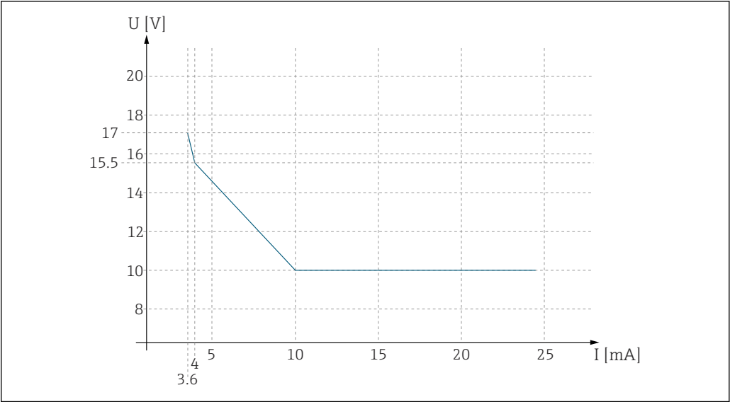
图 30 变送器的最小供电电压，取决于输出电流
