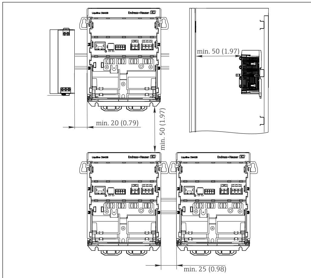
38 最小安装间距；单位：mm (in)
