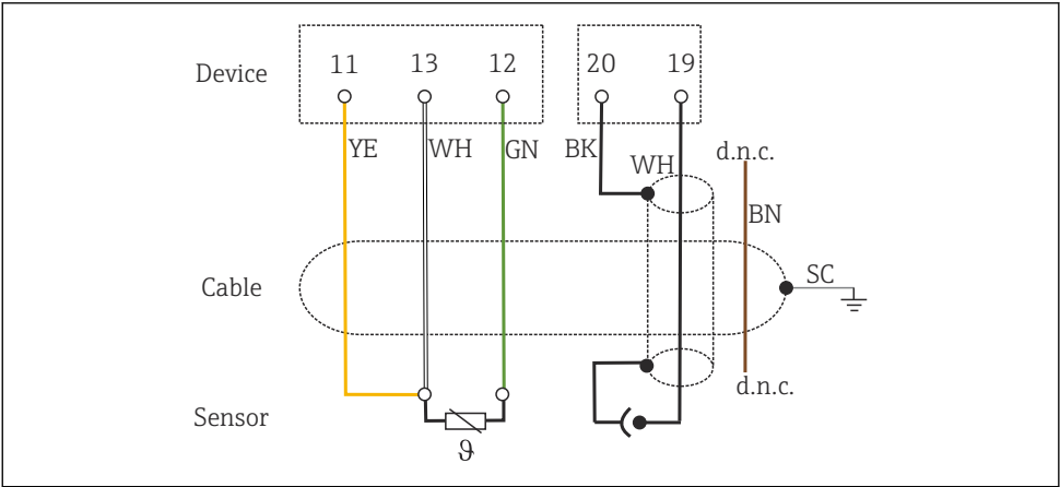
图 11 接线图
