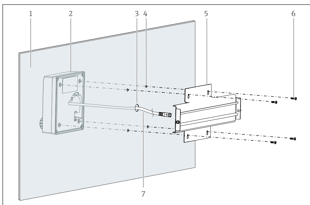
图 40 安装外接显示单元和 DIN 导轨
