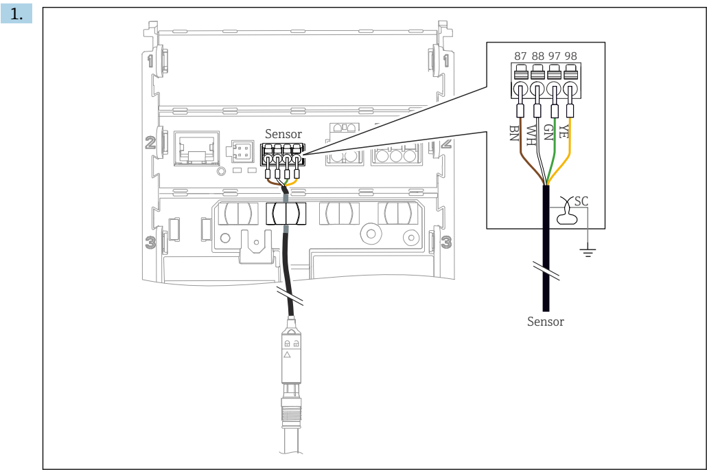
图 6 连接 Memosens 数字式传感器
