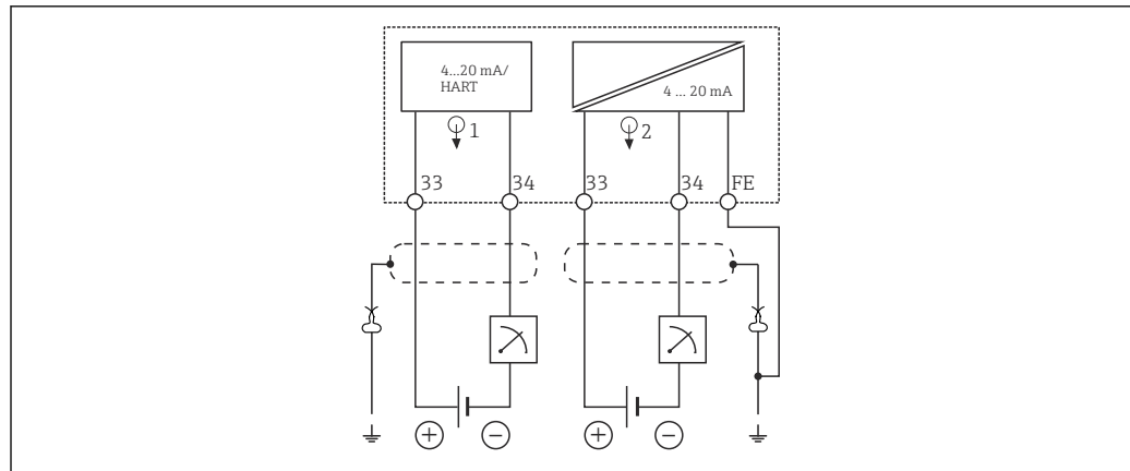
图 29 接线图：2 路电流输出（电流输出 1 叠加 HART 信号）
