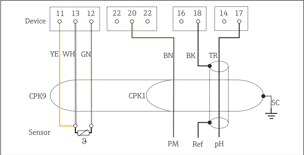
14 接线图
