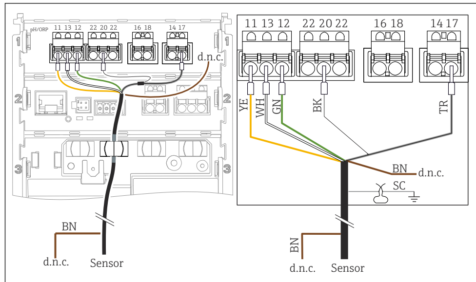
15 设备视图
