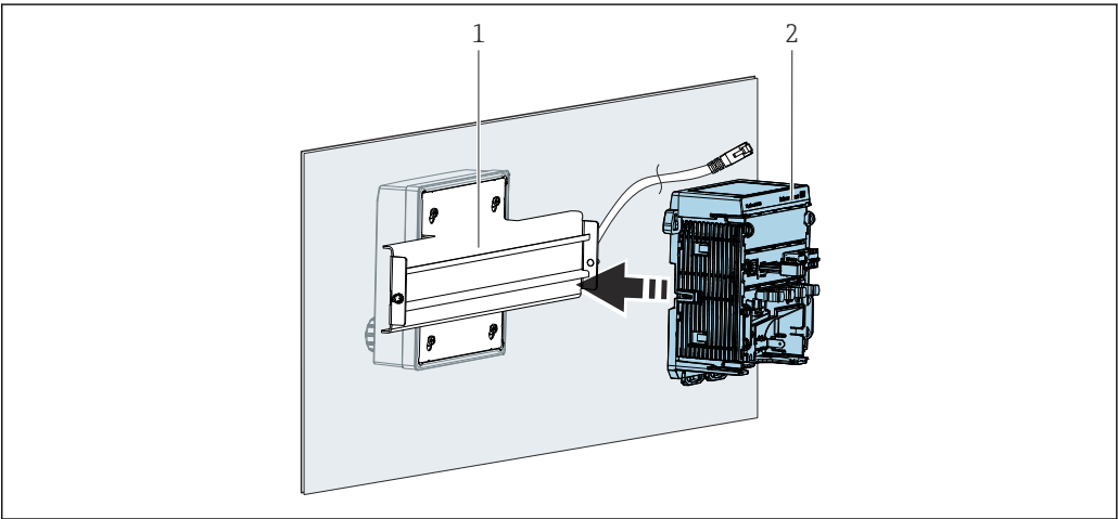
图 42 安装变压器
