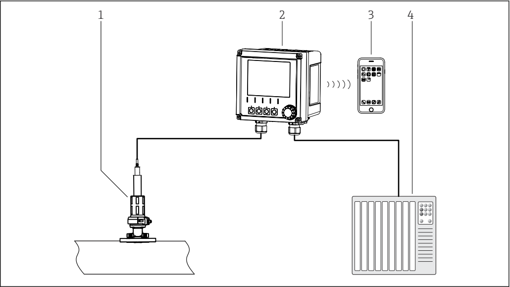
图 1 安装有 Liquiline CM42B（现场型设备）的测量系统示意图
