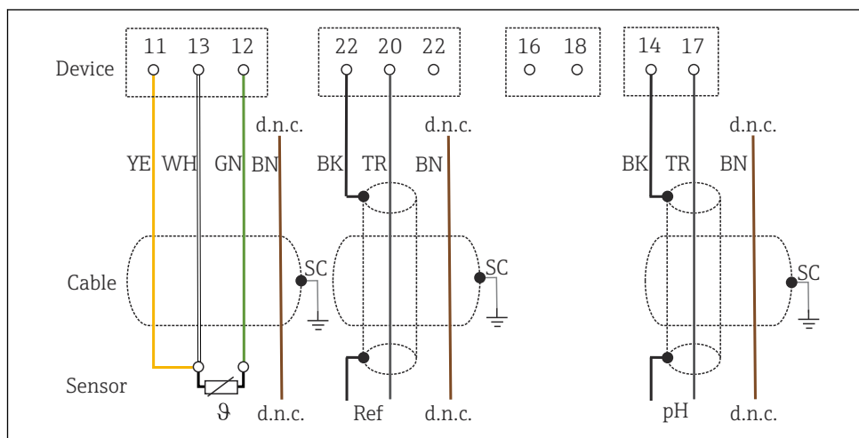
图 24 接线图
