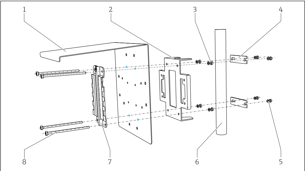
34 立柱安装
