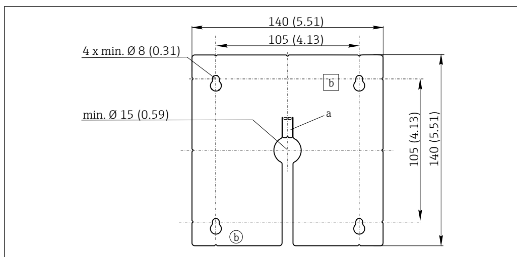
图 39 外接显示单元的安裝板的外形尺寸示意图；单位：mm (in)
