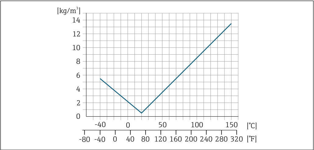
35 Ajustage sur site de la masse volumique, par exemple à +20 °C (+68 °F)
