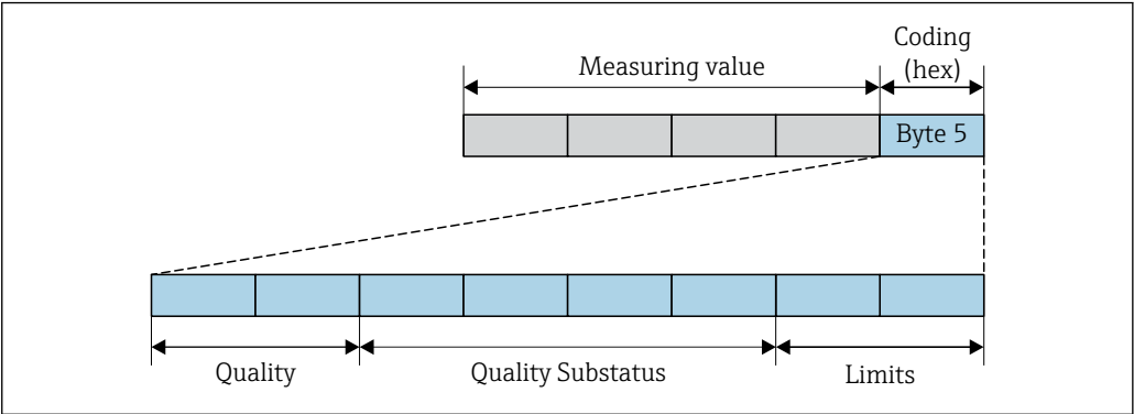
32 Structure de l'octet de codage
