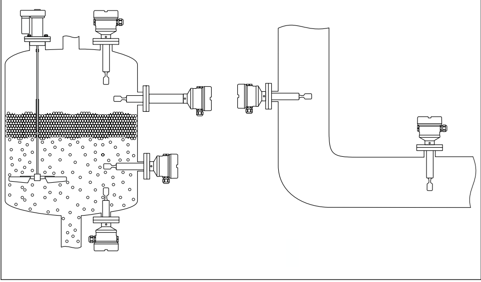
2 Bir kanal, tank veya boru için kurulum örnekleri
