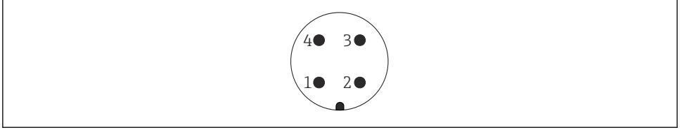
16 M12 fiş, pin ataması
