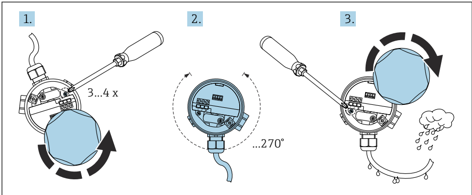
14 Kilitleme vidası bulunan muhafaza; kabloda damlama döngüsü oluşturun
