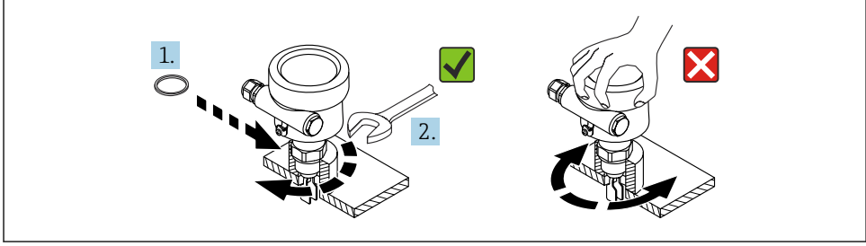
13 Cihazın vidalanması
