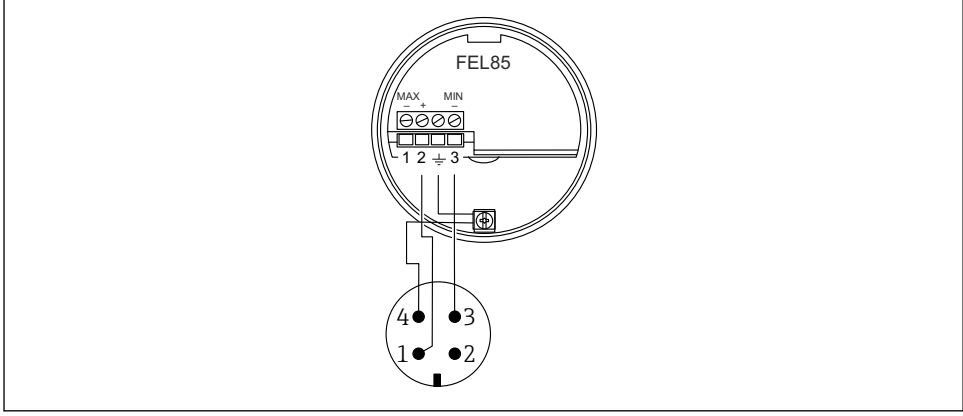
18 M12 konnektörlü terminal ataması, minimum algılama çalışma modu
