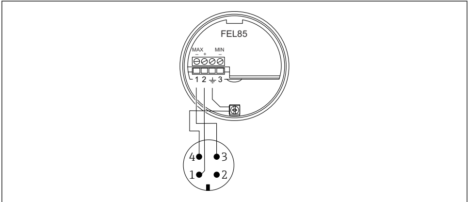
17 M12 konnektörlü terminal ataması, maksimum algılama çalışma modu
