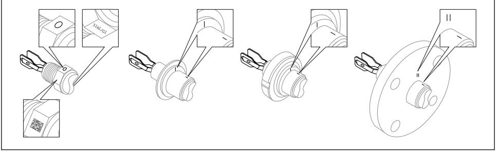
11 İşaretleme kullanılarak kaba yatay olarak monte edildiğinde titreşim çatalının konumu
