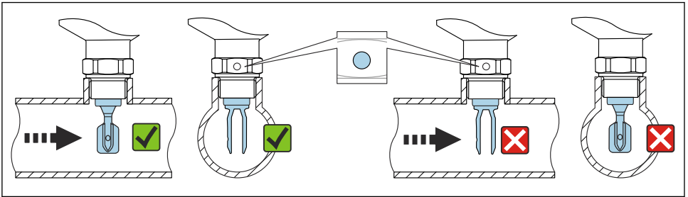
12 Boru tesisatına montaj (çatal pozisyonunu ve işareti dikkate alın)
