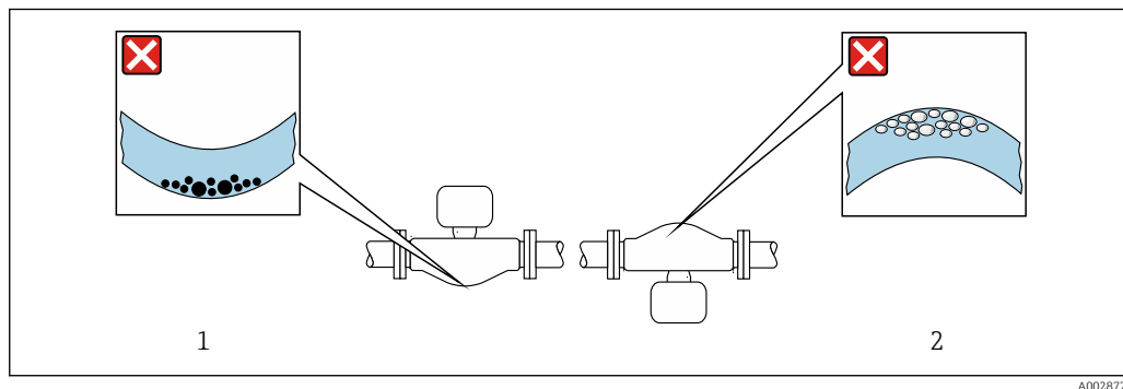
15 Orientamento del sensore con tubo di misura curvo
