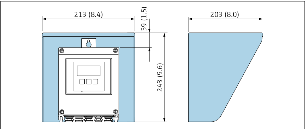
34 Tettuccio di protezione dalle intemperie per Proline 500 – digital; unità ingegneristica mm (in)
