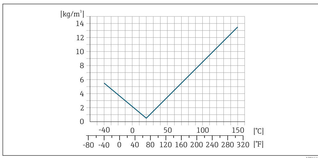
13 Regolazione della densità in campo, ad es. a +20 °C (+68 °F)
