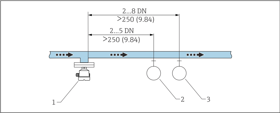
9 后直管段的安装。测量单位 mm (in)
