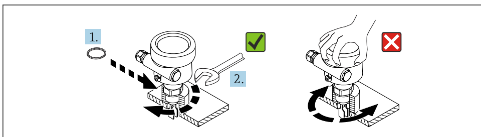
15 旋转拧入设备
