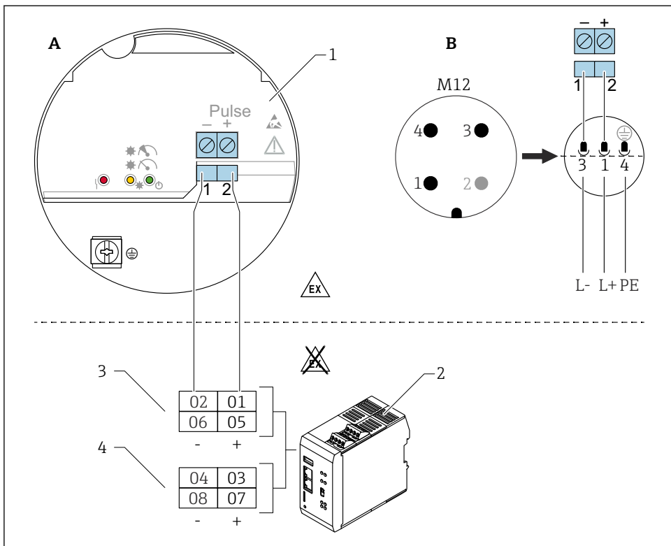
图 19 电子插件 FEL60D 和密度计算仪 QML51 的接线图
