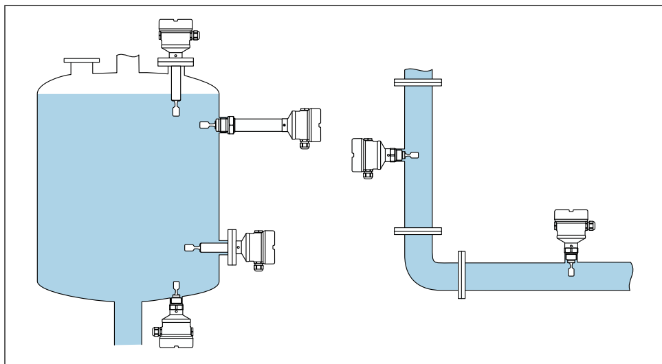
图 4 安装实例：安装在容器、罐体或管道中
