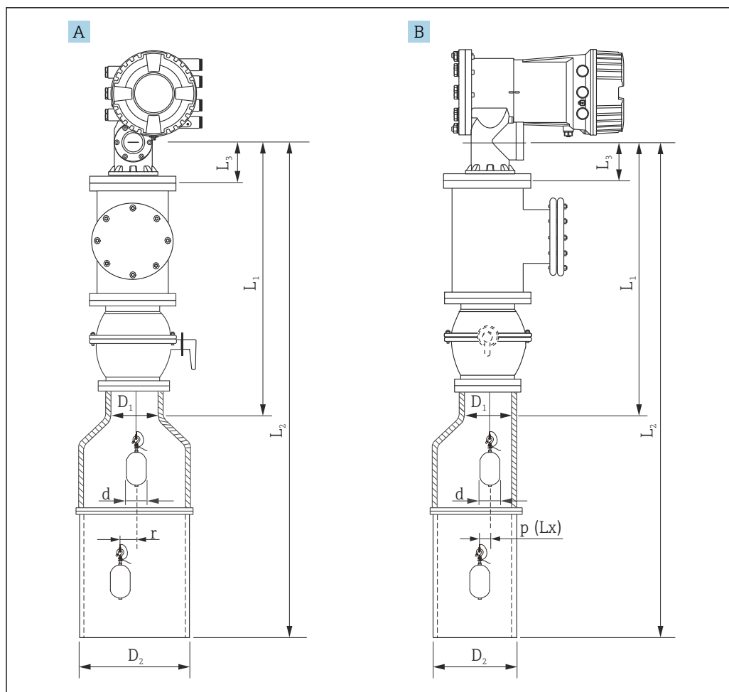
■ 15 Montaje con tubo tranquilizador asimétrico
