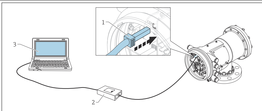
23 Configuración a través de la interfaz de servicio
