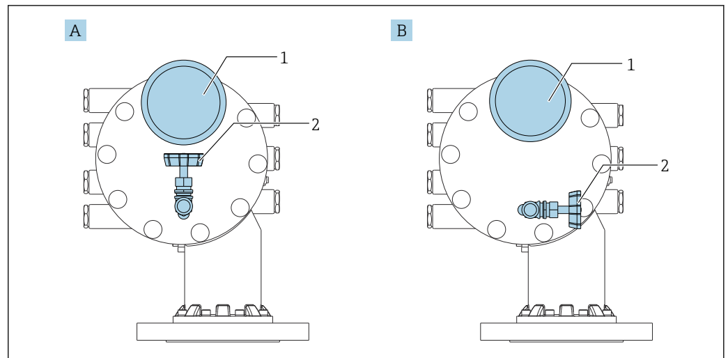
28 Posición de montaje de la válvula de descarga y el medidor de presión
