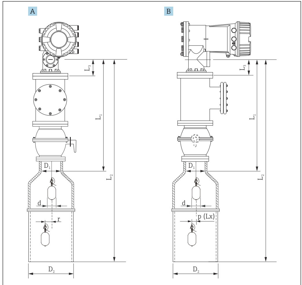
14 Montaje con tubo tranquilizador concéntrico
