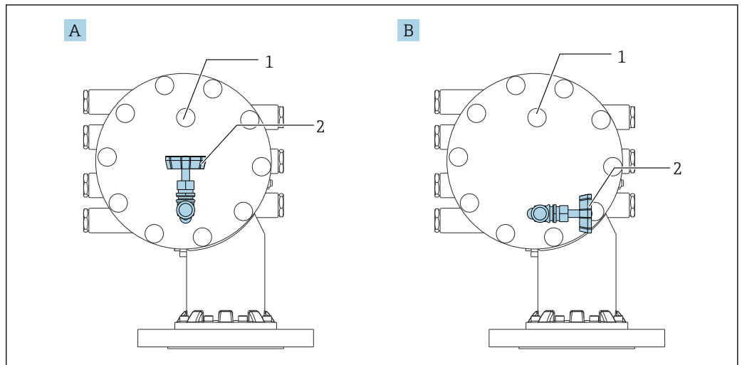
32 Boquilla de limpieza y válvula de alivio de presión
