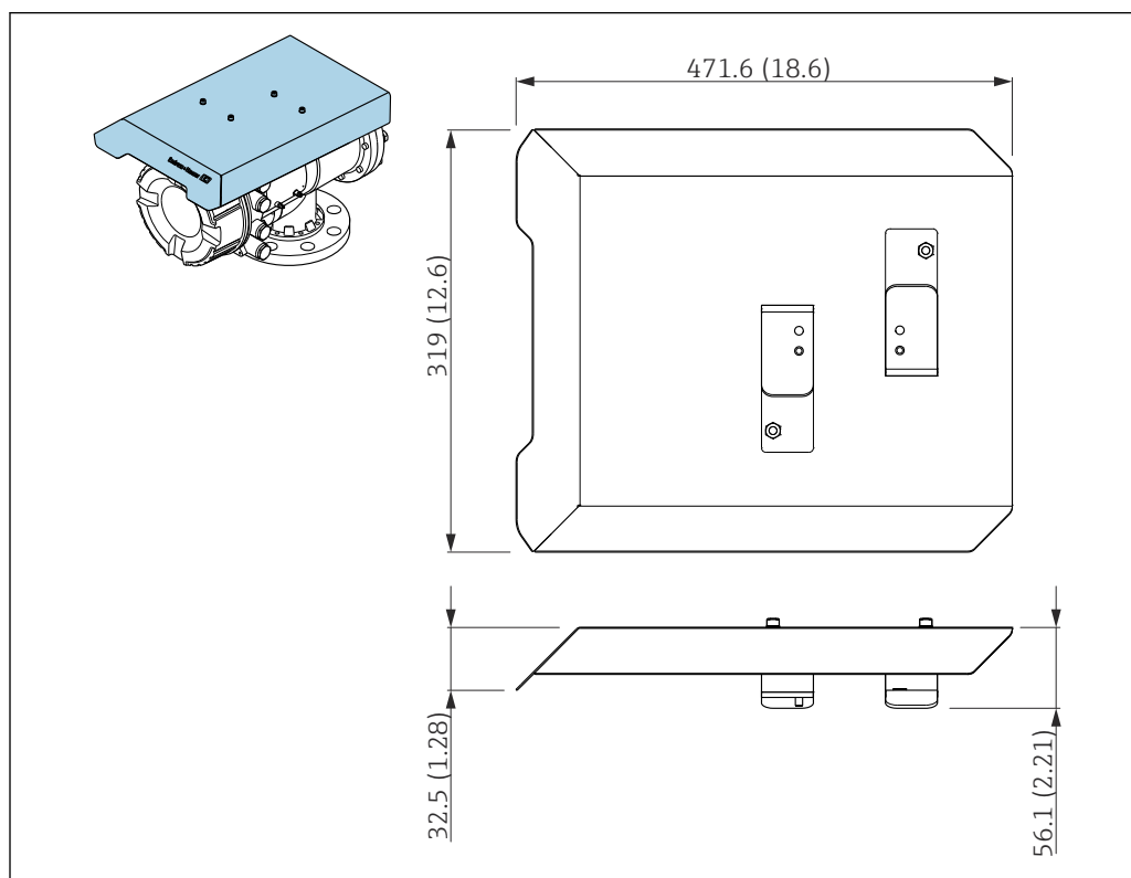
27 Tapa de protección ambiental, medidas: mm (in)
