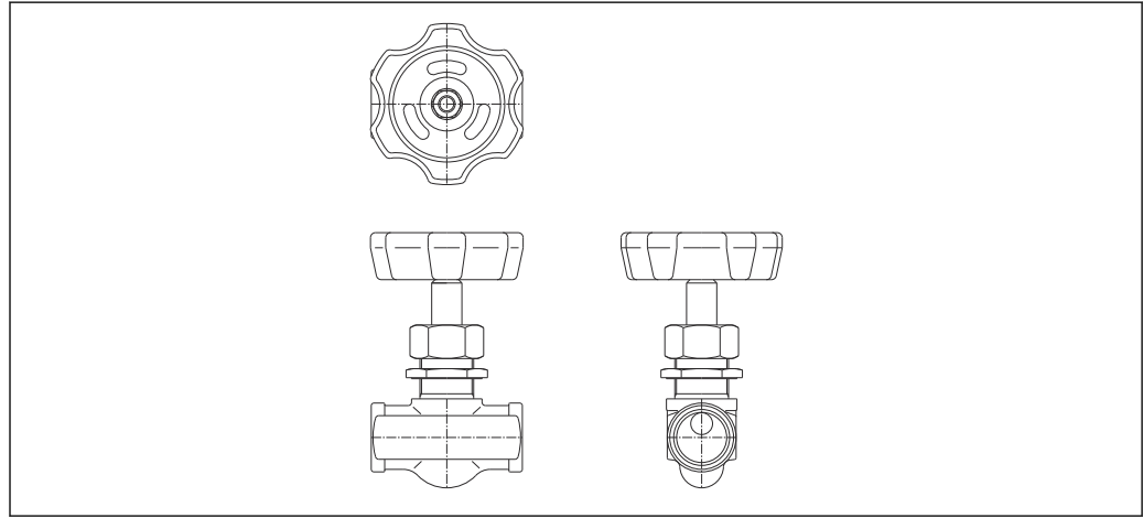
29 Válvula de descarga
