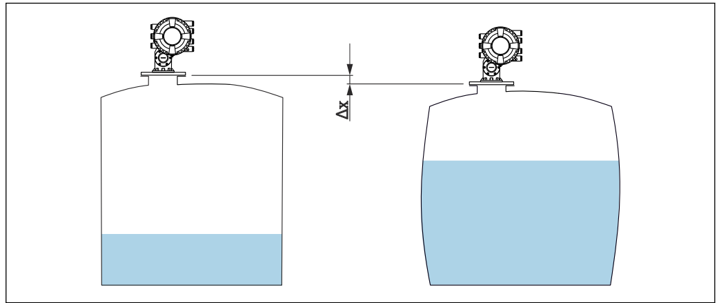
24 Movimiento \Delta x de la altura de referencia del depósito debido al pandeo de la pared del depósito causado por la presión hidrostática
