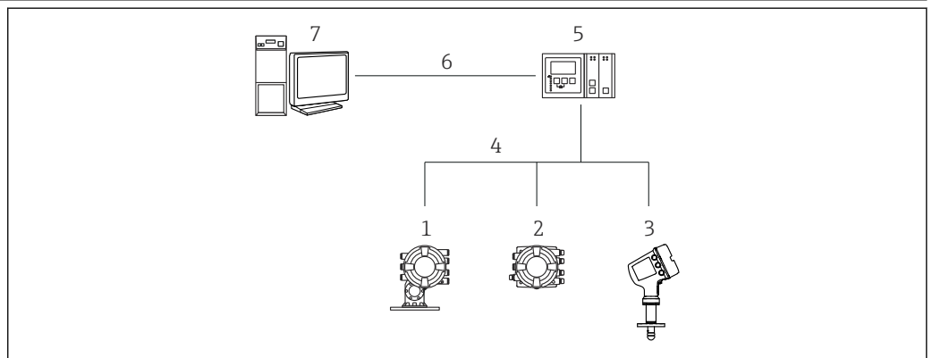
Fig. 22 Configuración a distancia de equipos de medición de depósitos
