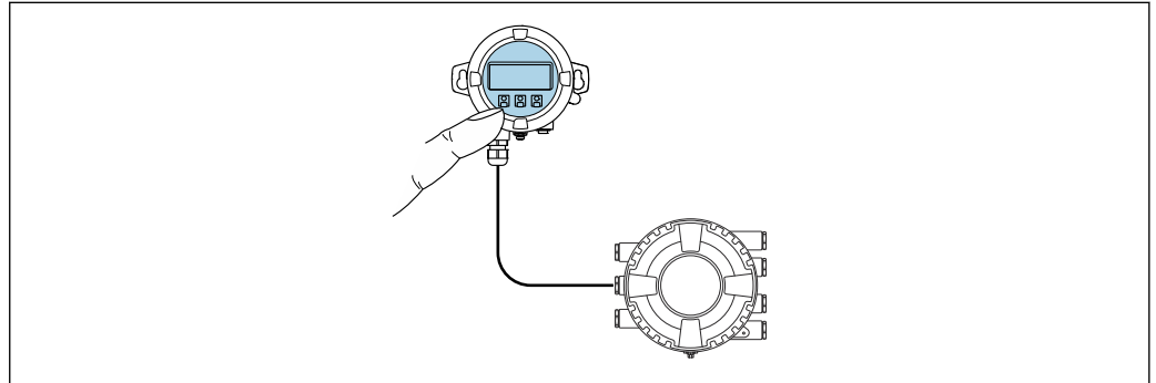
Fig. 21 Configuración a través del módulo de indicación y configuración a distancia DKX001
