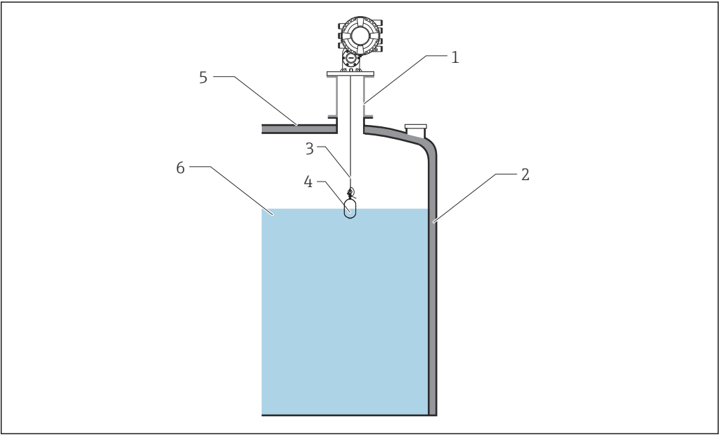
18 Sellado del proceso
