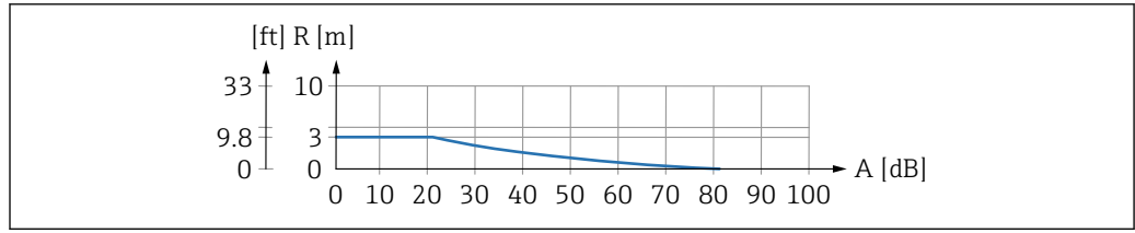
☐ 2 초음파 센서의 범위 차트
