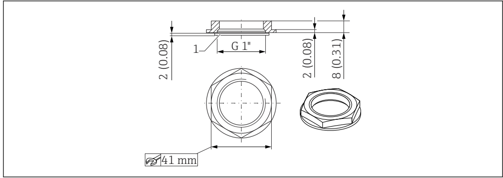
☞ 11 카운터 너트; 치수. 측정 단위 mm (in)
