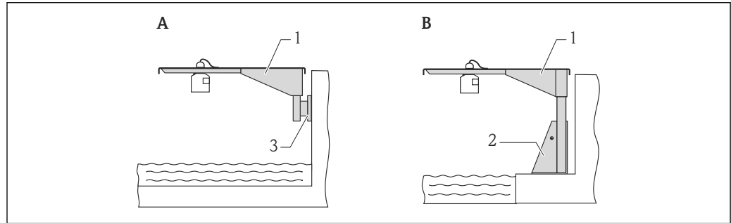
16 캔틸레버 암을 사용한 센서 설치
