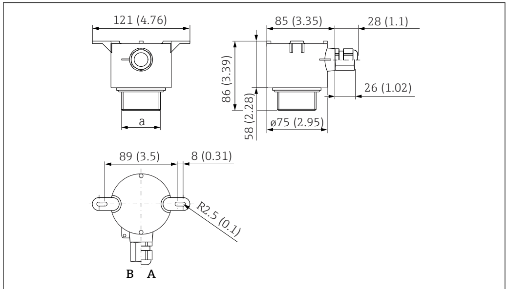
☐ 10 FDU90-*W*** (천장 설치). 측정 단위 mm (in)
