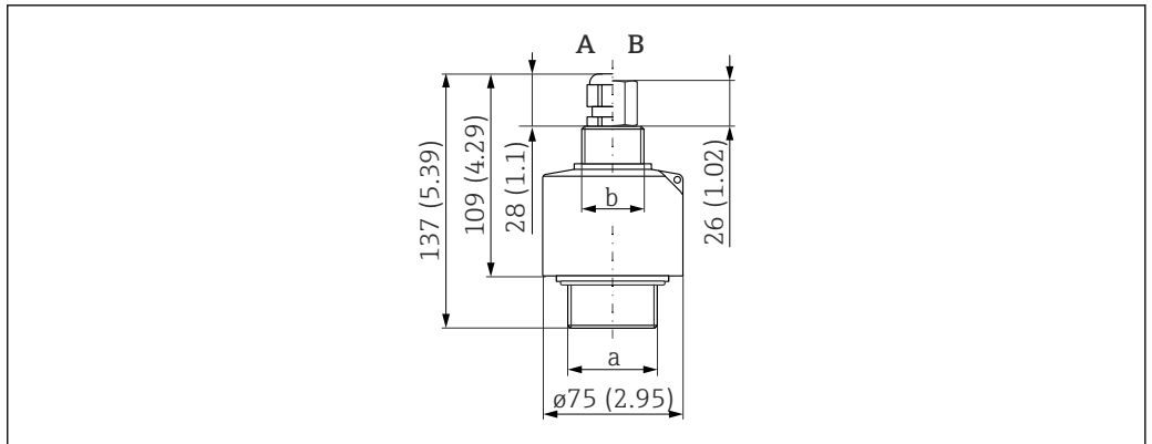
☐ 9 FDU90-*G*** (G1 및 G1-1/2 나사); FDU90-*N*** (NPT 1 및 NPT 1-1/2 나사). 측정 단위 mm (in)
