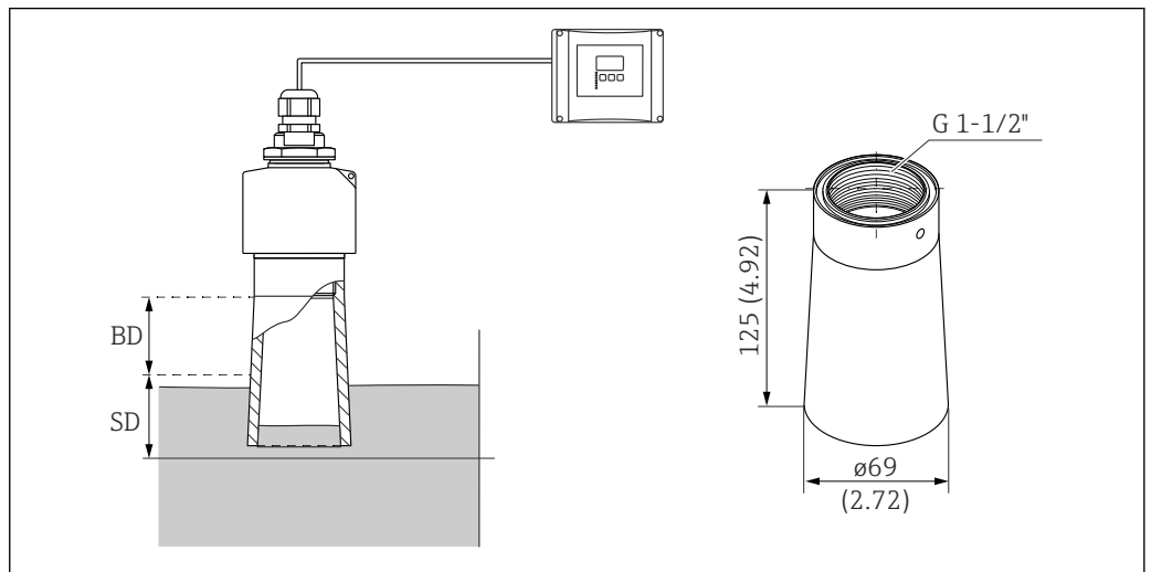
15 침수 방지 튜브. 측정 단위 mm (in)
