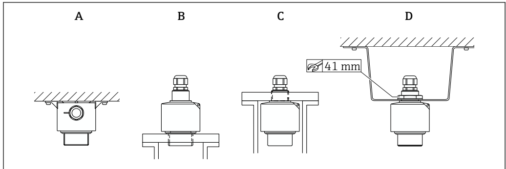
☞ 8 초음파 센서 고정
