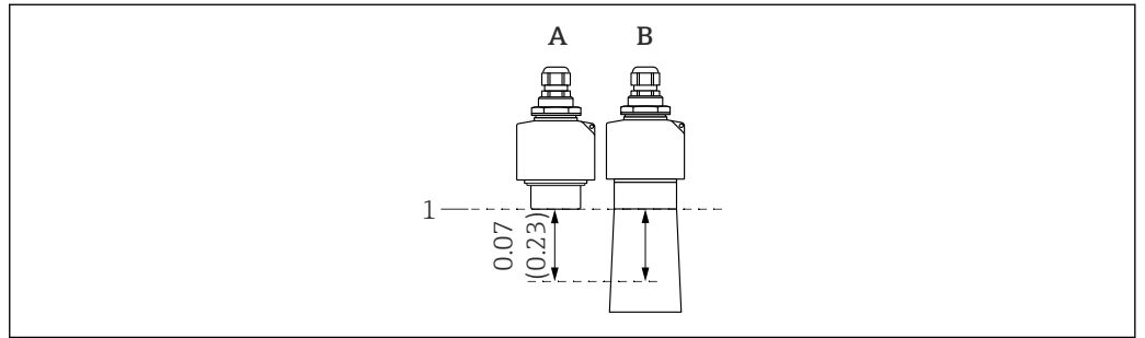
☐ 1 초음파 센서의 불감대. 공학 단위 m (ft)
