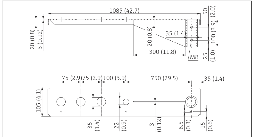
☒ 18 치수. 측정 단위 mm (in)
