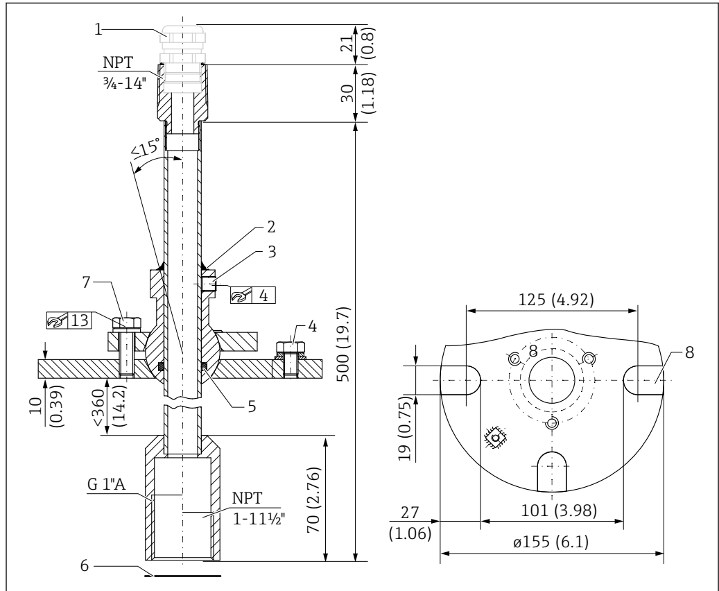
☐ 23 FAU40 정렬 장치. 측정 단위 mm (in)
