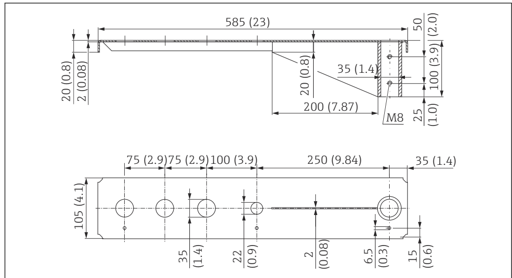
17 치수. 측정 단위 mm (in)
