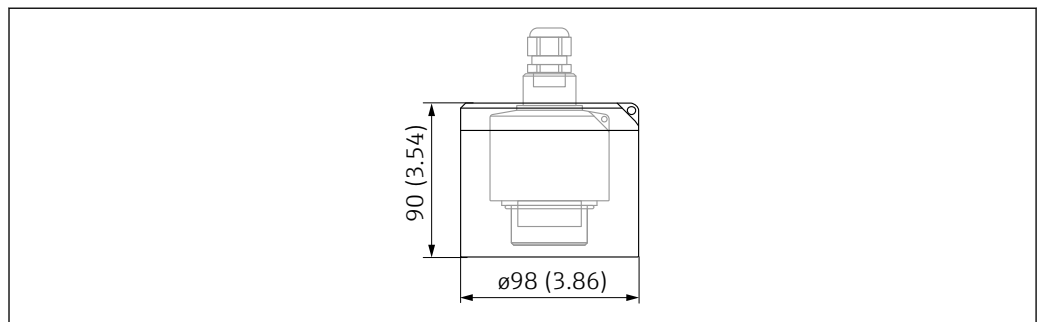
14 내후성 커버. 측정 단위 mm (in)
