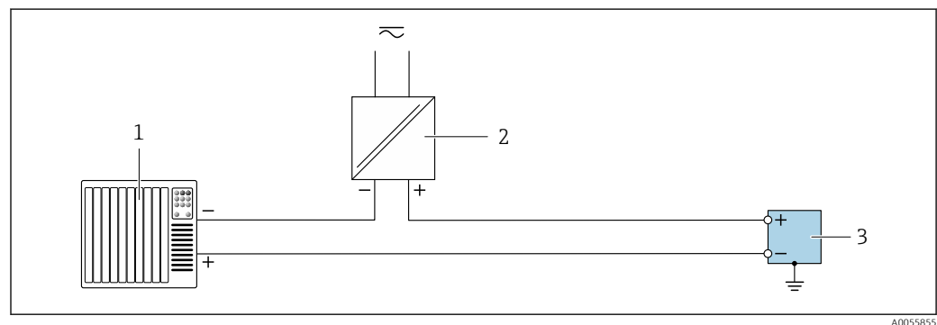
9 Exemple de raccordement pour sortie impulsion / sortie fréquence / sortie tout ou rien (passive)
